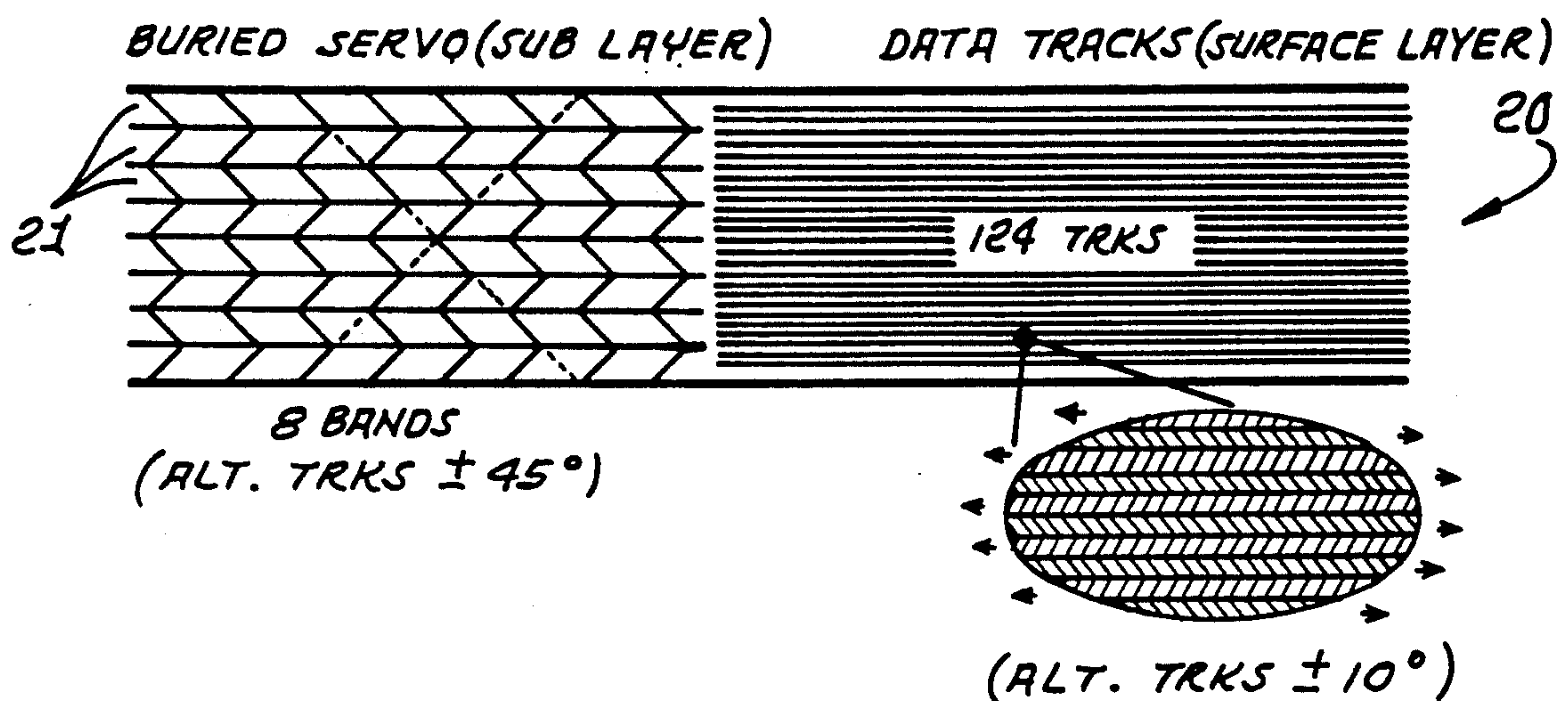
FIG. 2. TAPE FORMAT
