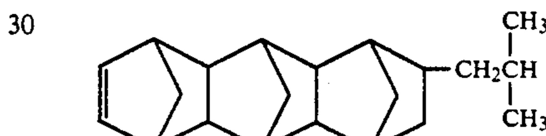
12-Isobutylhexacyclo[6,6,1,1 3.6 ,1 10.13 ,0 2.7 ,0 9.14 ]-4-heptadecene
