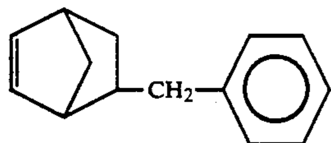
5-Benzylbicyclo[2,2,1]hept-2-ene
