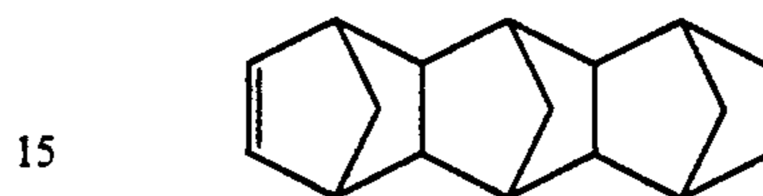
Hexacyclo[6,6,1,1 3.6 ,1 10.13 ,0 2.7 ,0 9.14 ]-4-heptadecene
