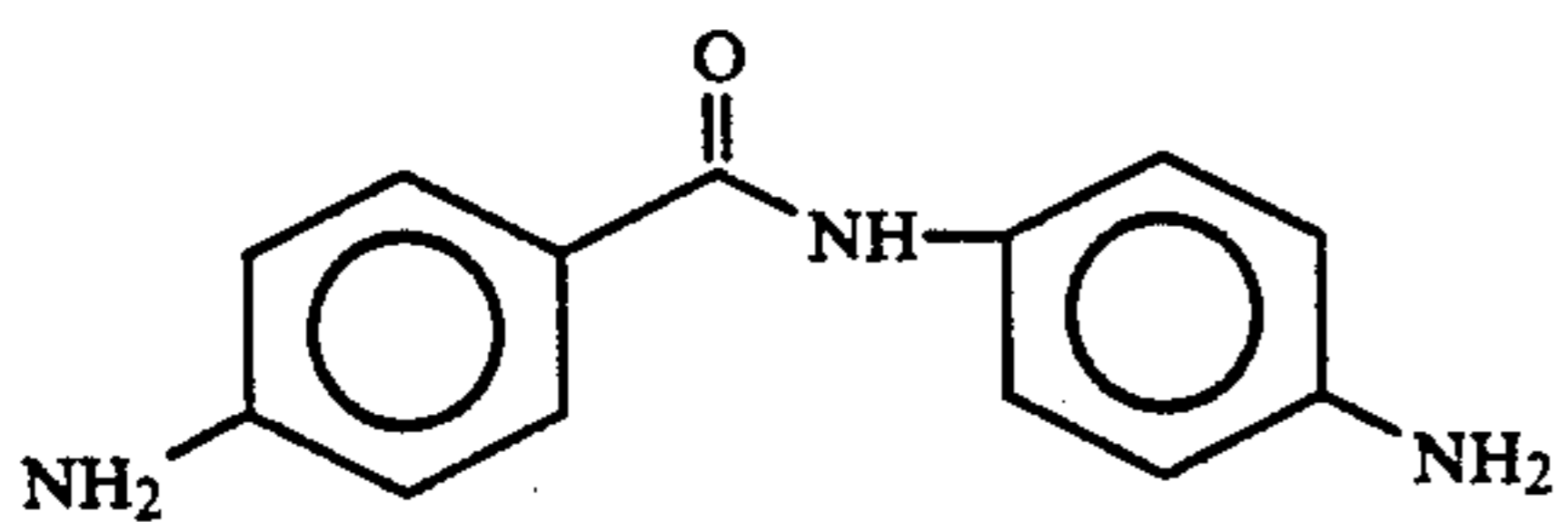
DABA
