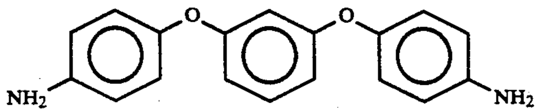
RODA
