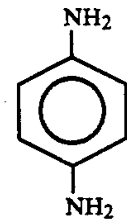
PPD
