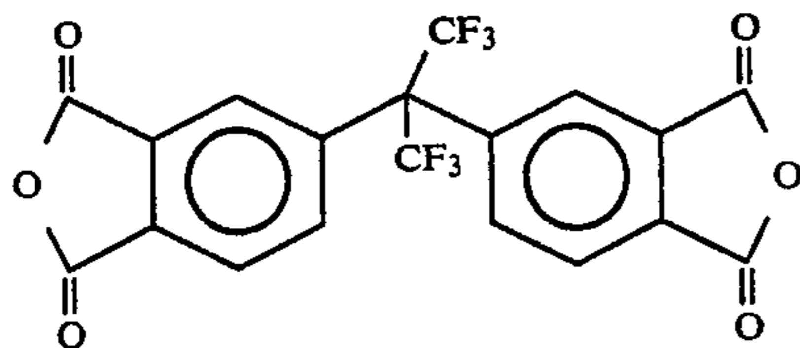
6FDA
