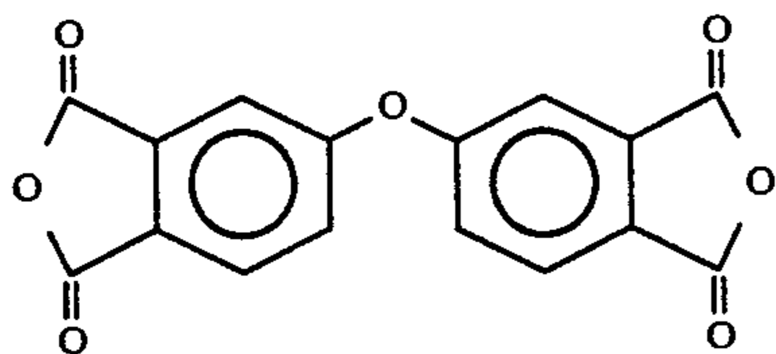
ODPA
