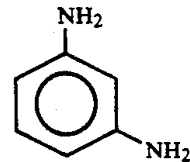
MPD
