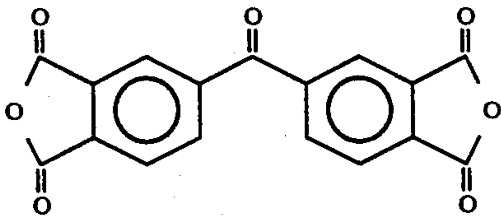
BTDA
