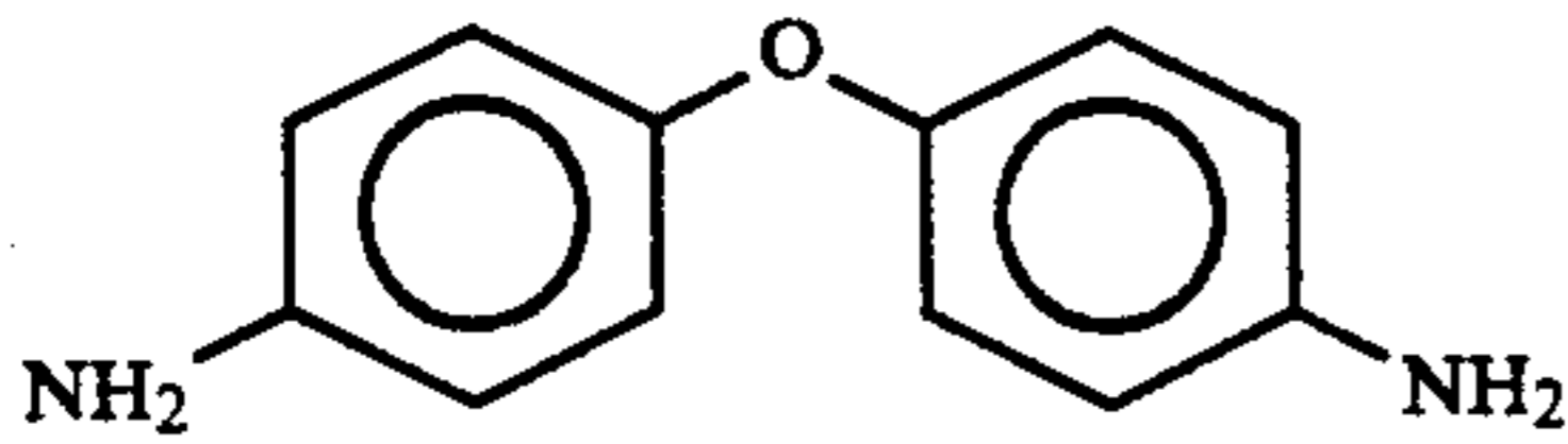
ODA
