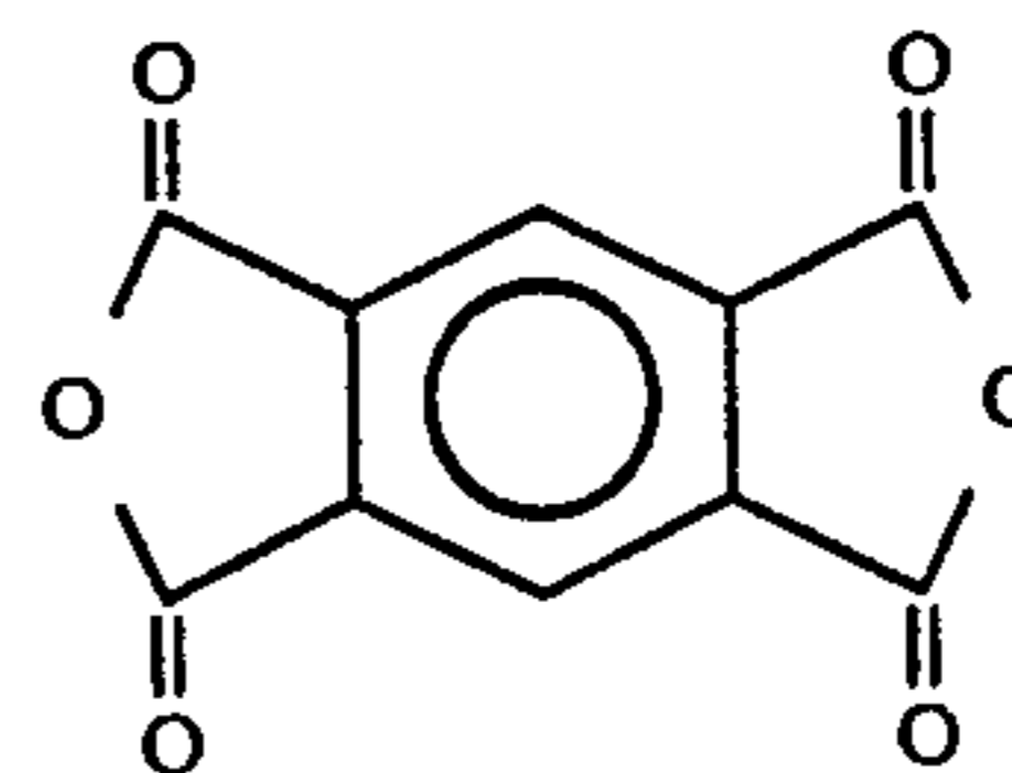
PMDA
