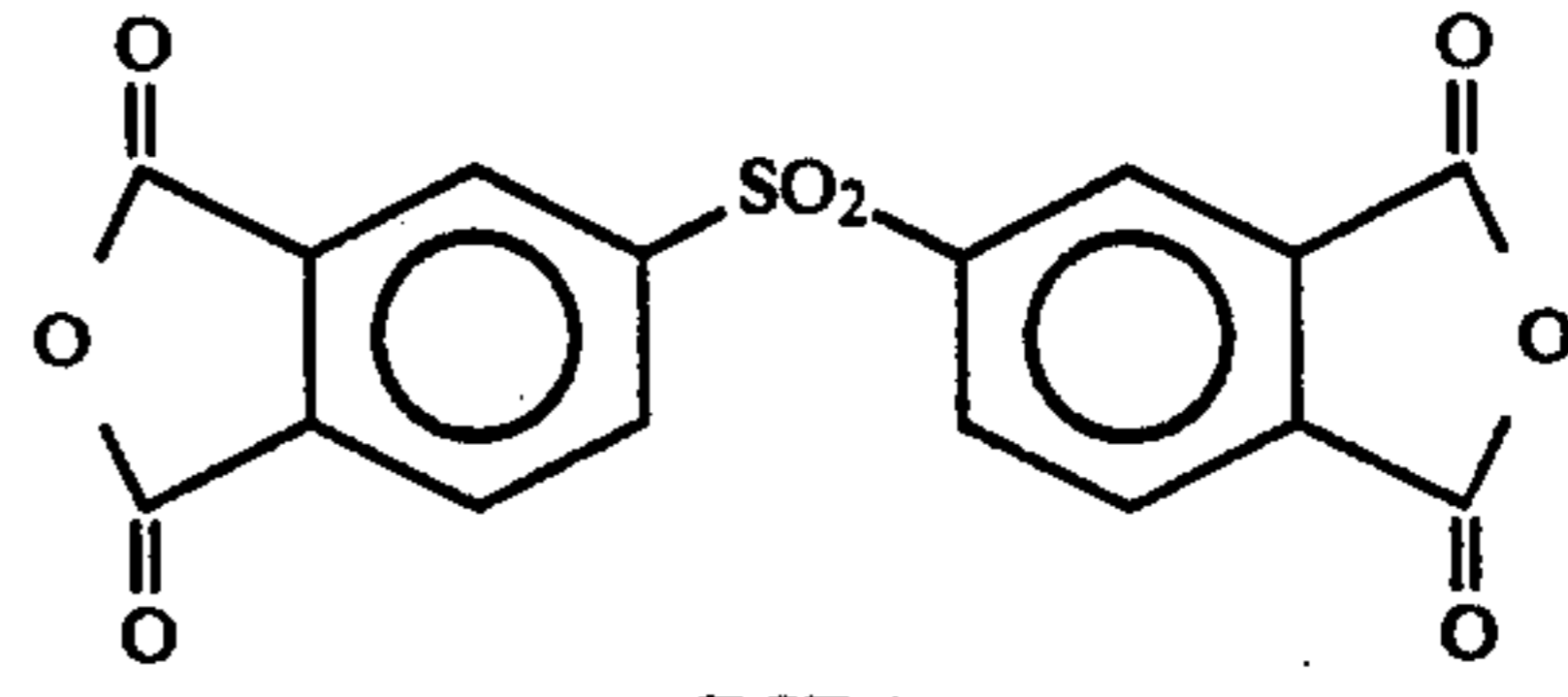
DSDA
