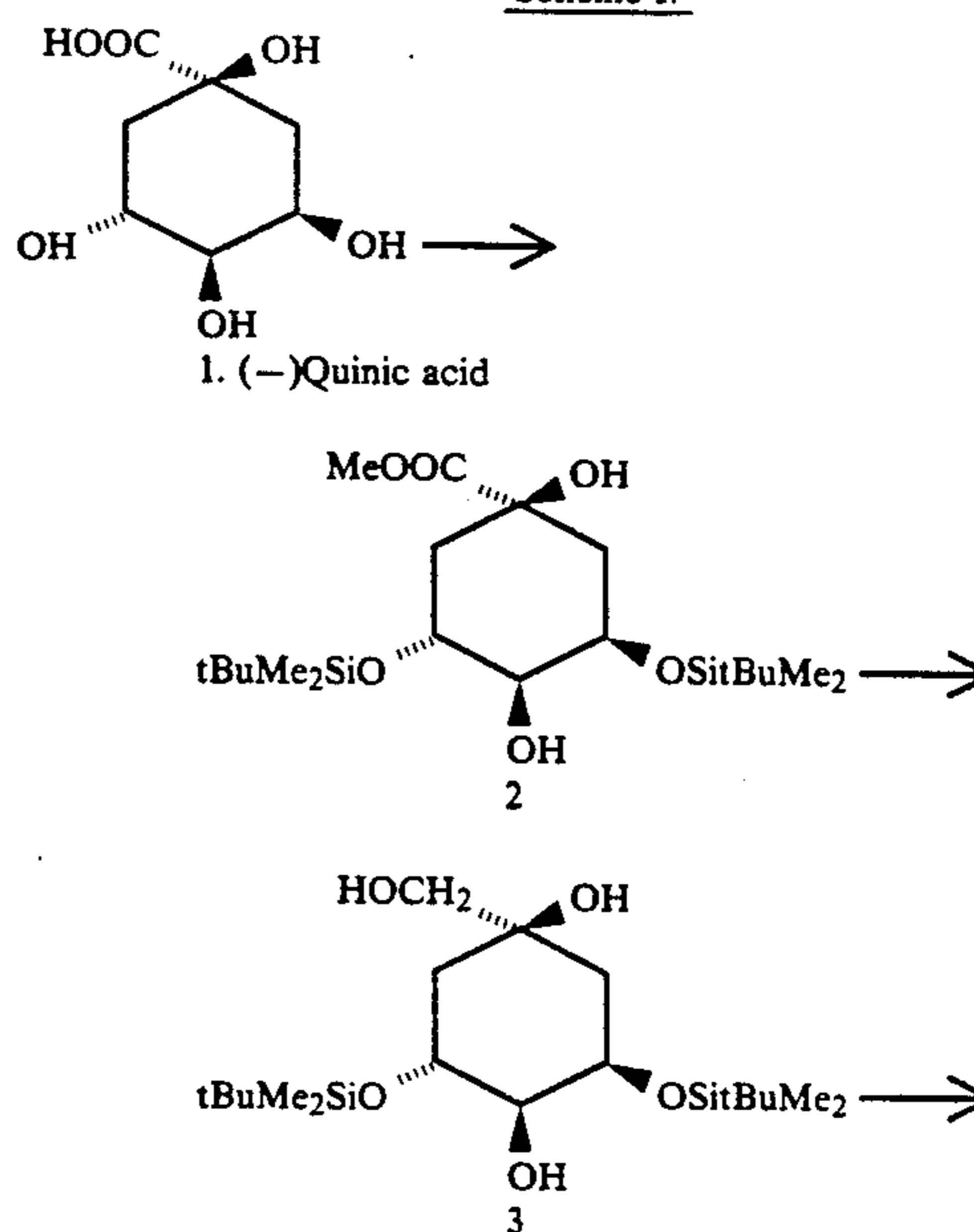
Scheme I.
