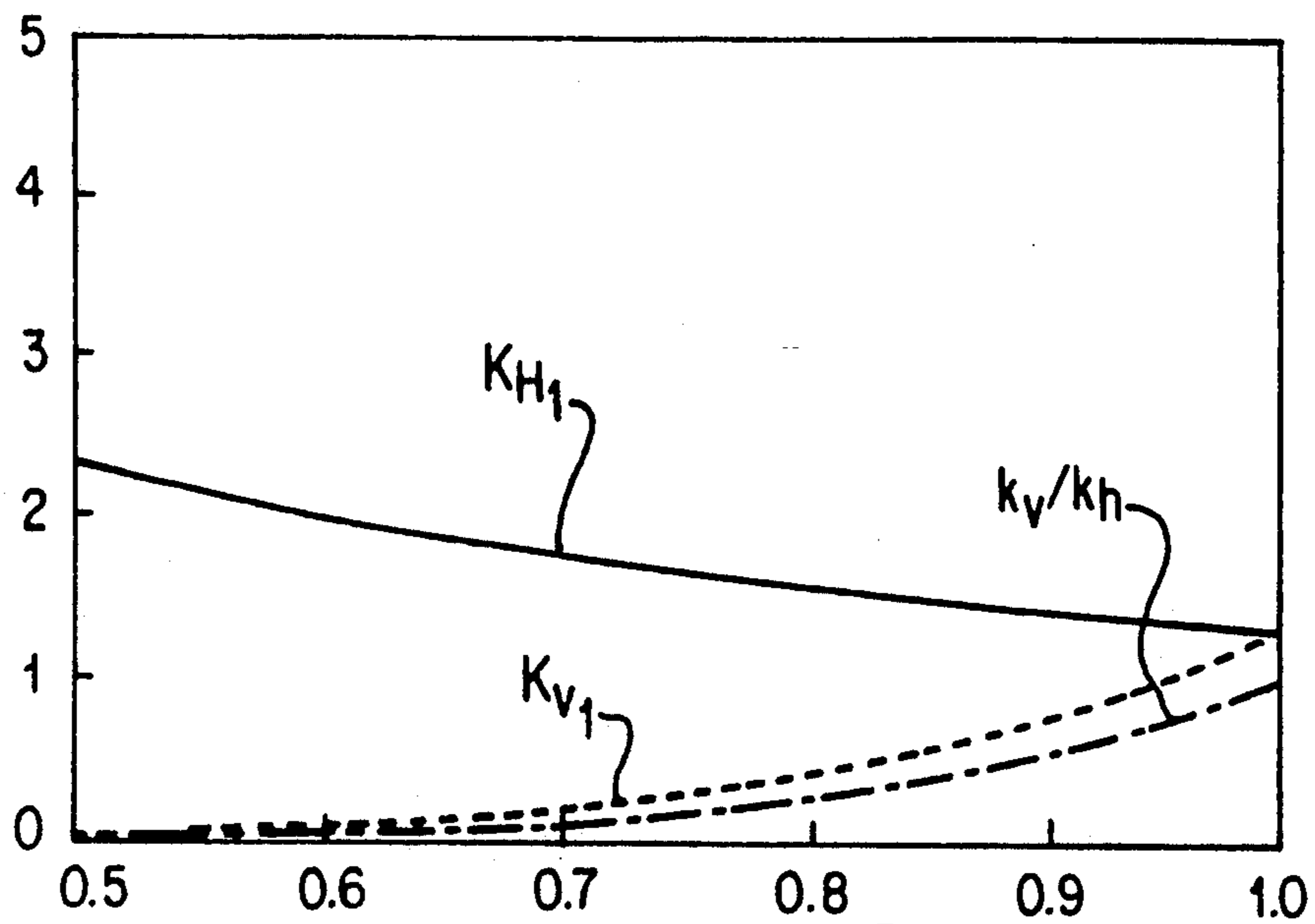
FIG. 19
