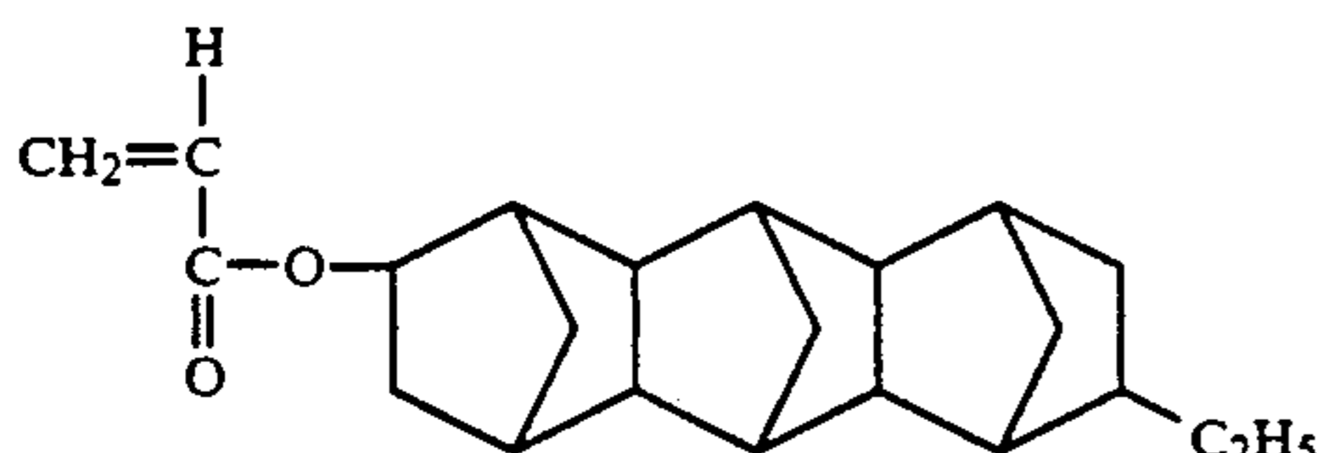
11-Ethylhexacyclo[6.6.1.1.3.6.10.13.0.2.7.0.9.14]heptadecyl-4-acrylate
