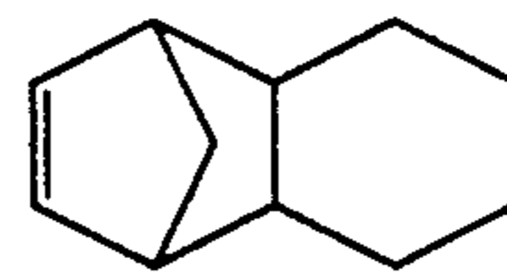
Tricyclo[4.4.0.1 2,5 ]-3-undecene
