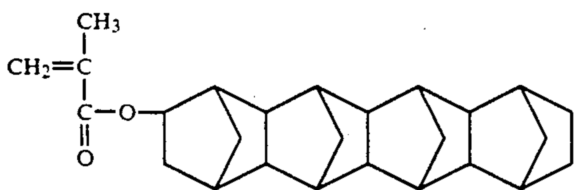
Octacyclo[8.8.12.9.14.7.11.18.15.16.0.3.8.0.12.17]-docosyl-5-methacrylate
