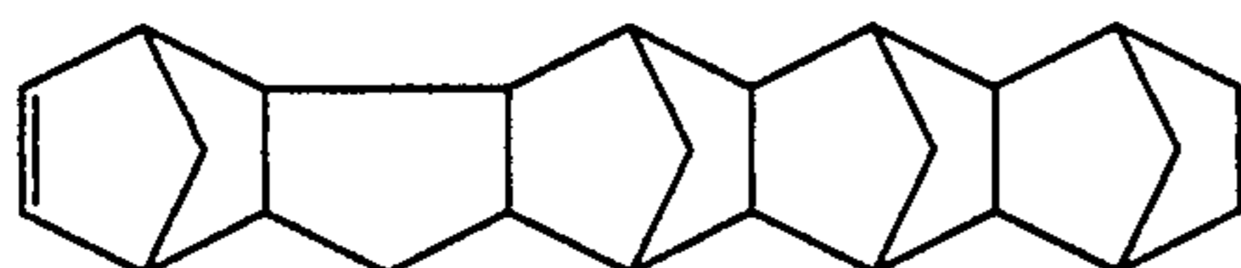
Nonacyclo[9.10.1.14.7.03.8.02.10.012.21.113.20.014.19.115.18]-5-pentacosene
