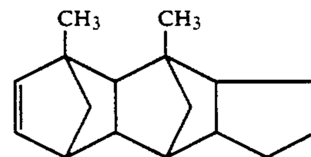
1,3-Dimethylpentacyclo[6.5.1.1.3.6.0.2.7.0.9.13]-4-pentadecene
