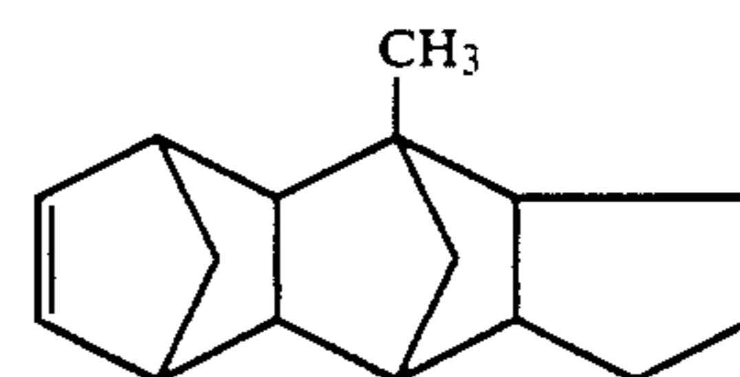
1,3-Dimethylpentacyclo[6.5.1.1.3.6.0.2.7.0.9.13]-4-pentadecene
