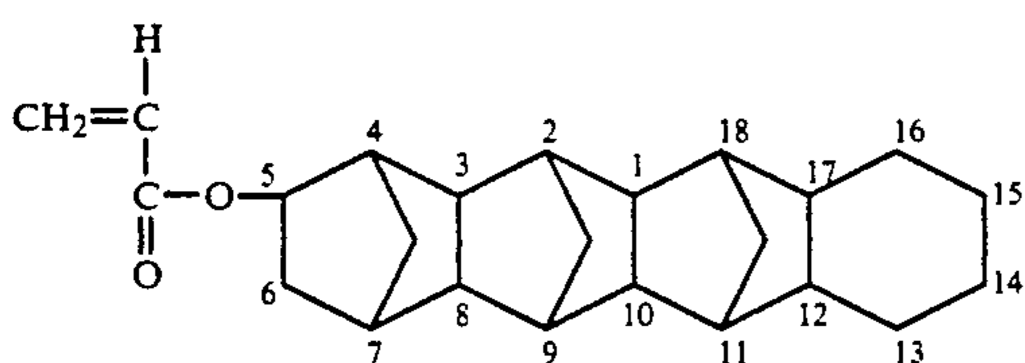
Octacyclo[8.8.12.9.14.7.11.18.15.16.0.3.8.0.12.17]docosyl-5-acrylate
