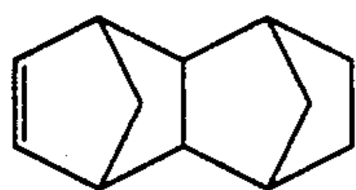
Tetracyclo[4.4.0.1 2,5 .1 7,10 ]-3-dodecene
