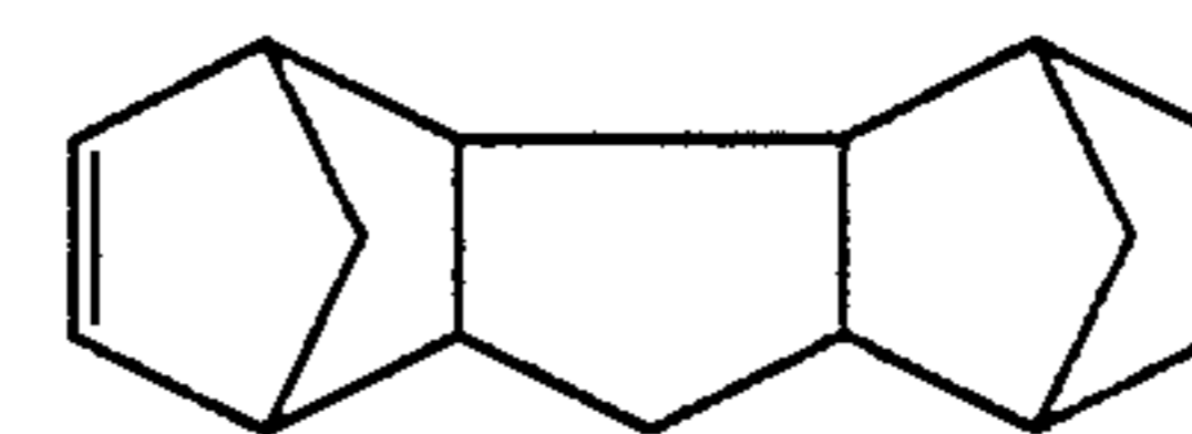
Pentacyclo[4.7.0.1 2,5 .0 8,13 .1 9,12 ]-3-pentadecene
