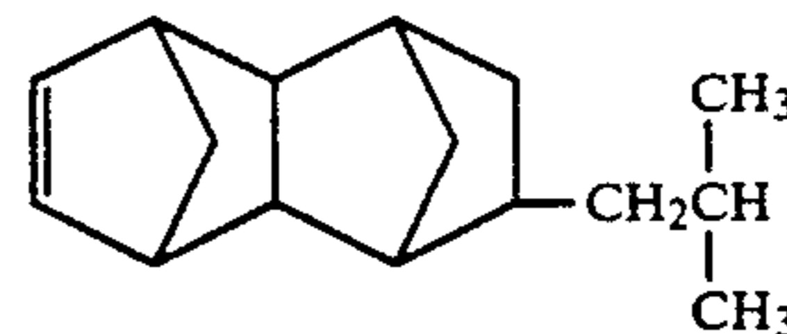
8-Isobutyltetracyclo[4.4.0.1 2,5 .1 7,10 ]-3-dodecene
