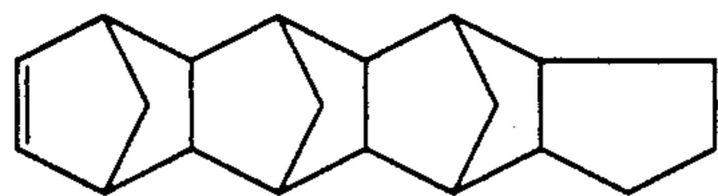
Heptacyclo[8.7.0.1.2.9.1.4.7.1.11.17.0.3.8.0.12.16]-5-eicosene
