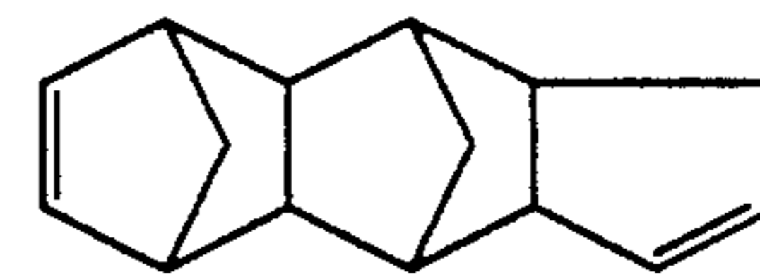
Pentacyclo[6.5.1.1.3.6.0.2.7.0.9.13]-4.10-pentadecadiene
