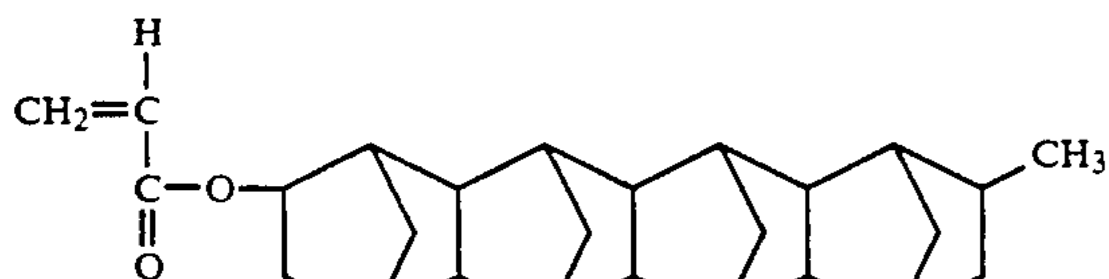
15-Methyloctacyclo[8.8.12.9.14.7.11.18.15.16.0.3.8.0.12.17]-docosyl-5-acrylate
