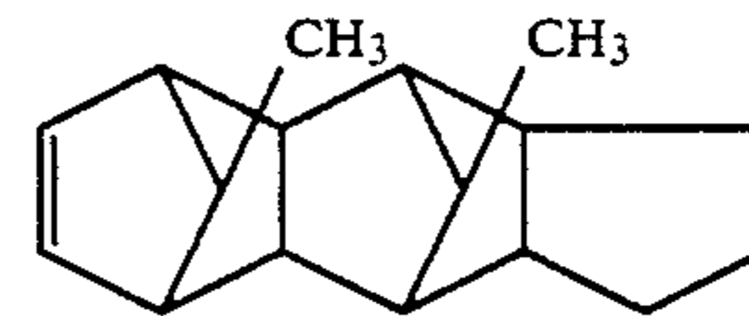
14,15-Dimethylpentacyclo[6.5.1.1.3.6.0.2.7.0.9.13]-4-pentadecene
