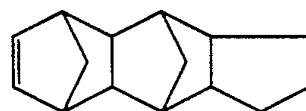
Pentacyclo[6.5.1.1.3.6.0.2.7.0.9.13]-4-pentadecene
