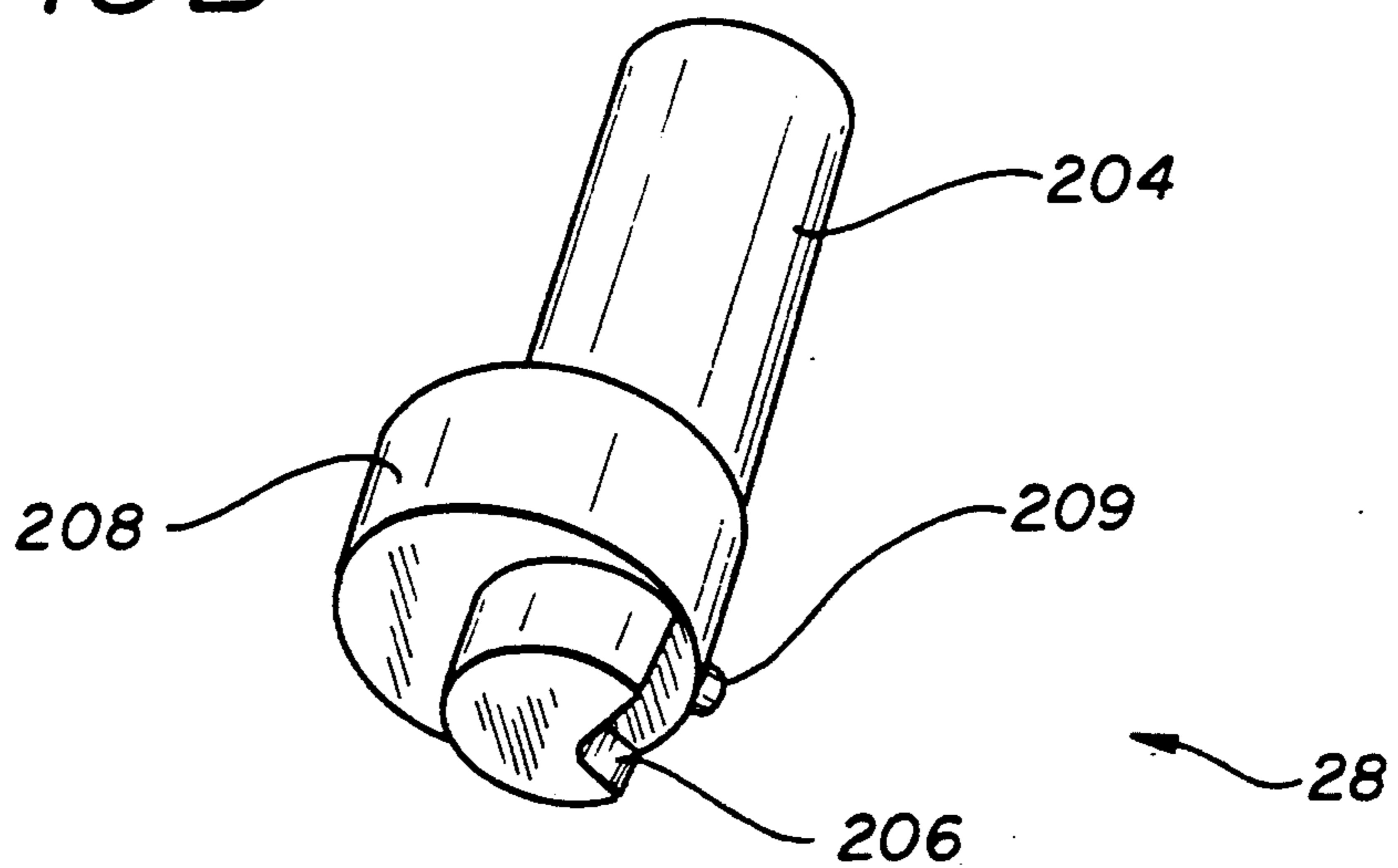
FIG-15B
