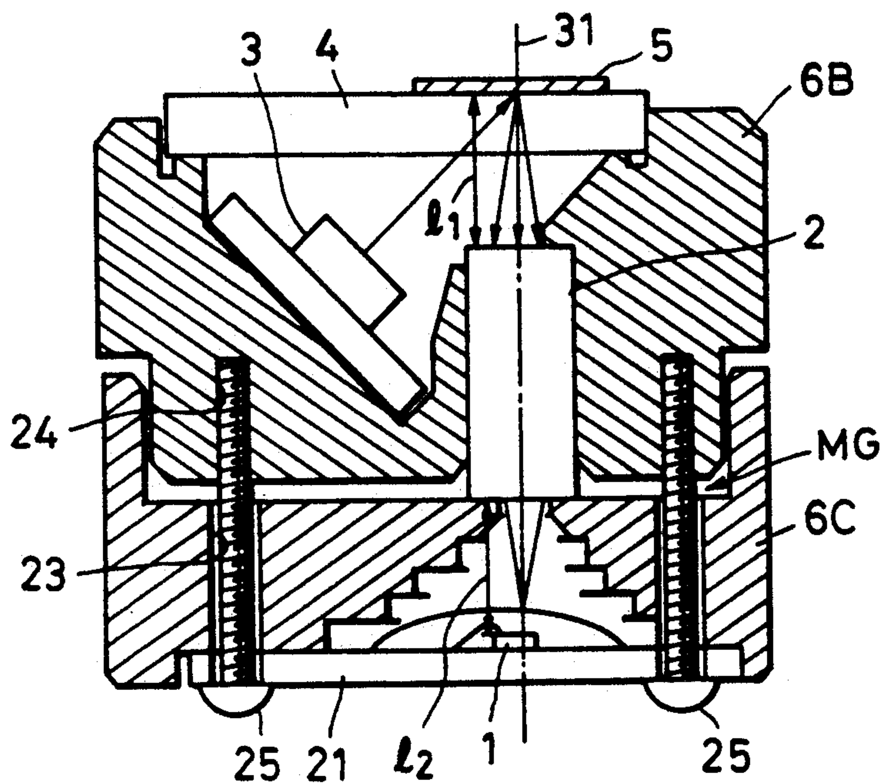
FIG. 6
