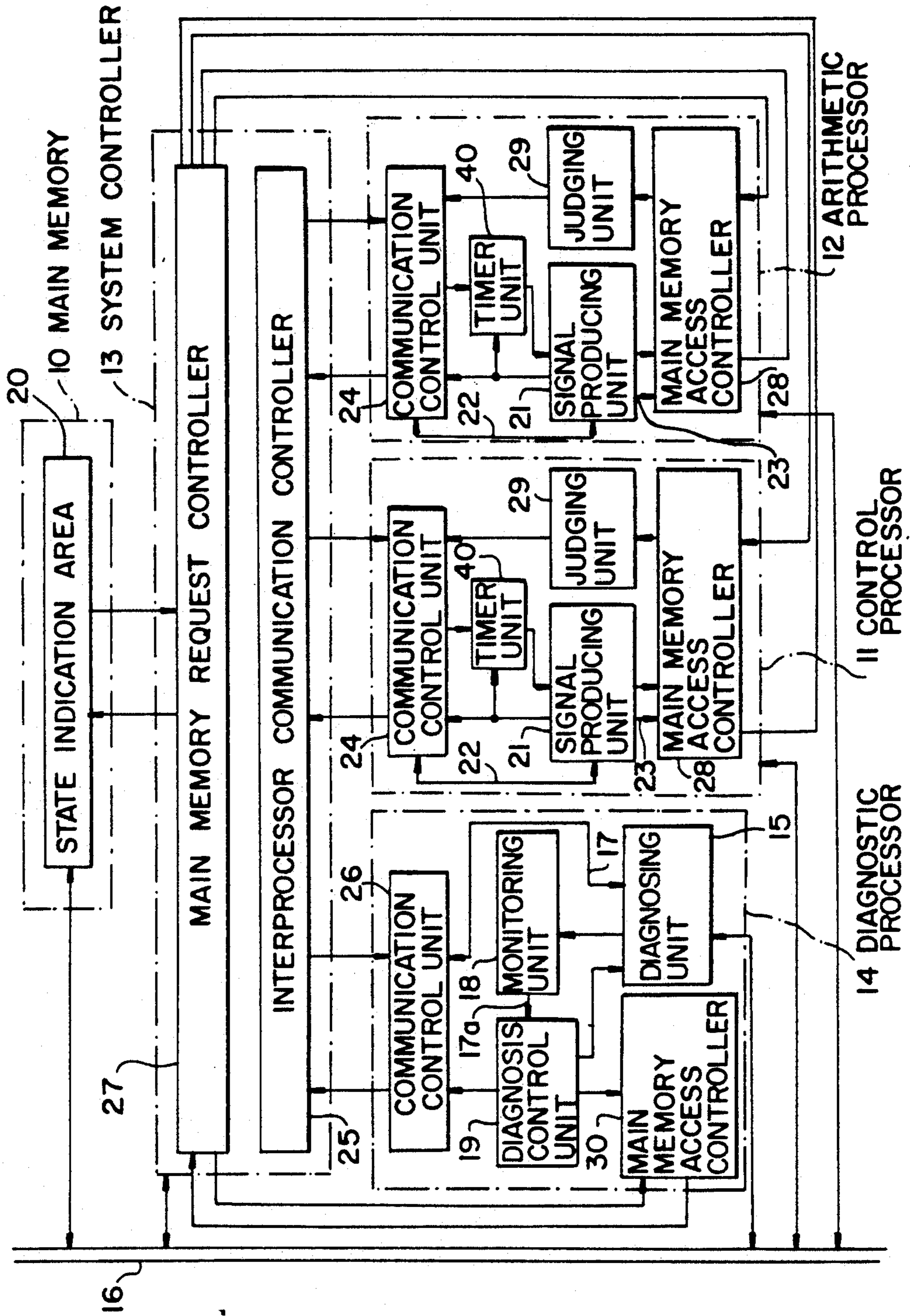
FIG. 1
