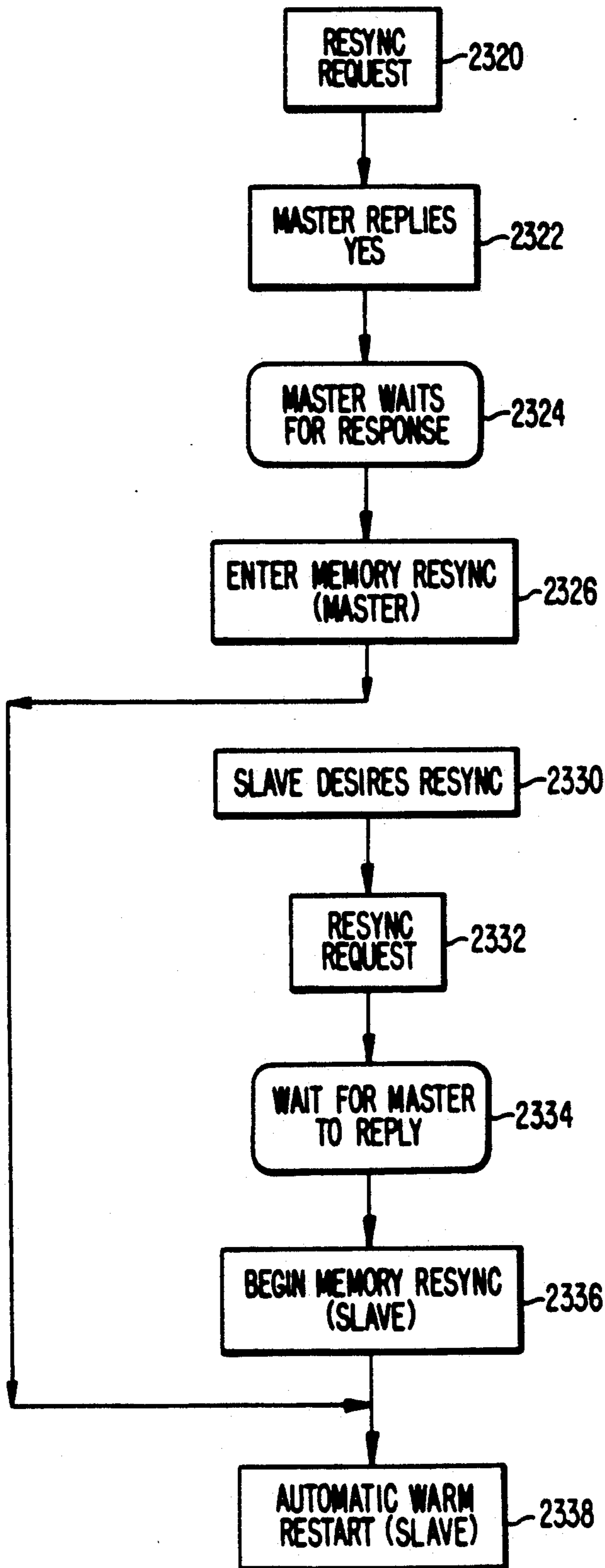
FIG. 23. MEMORY RESYNCHRONIZATION
