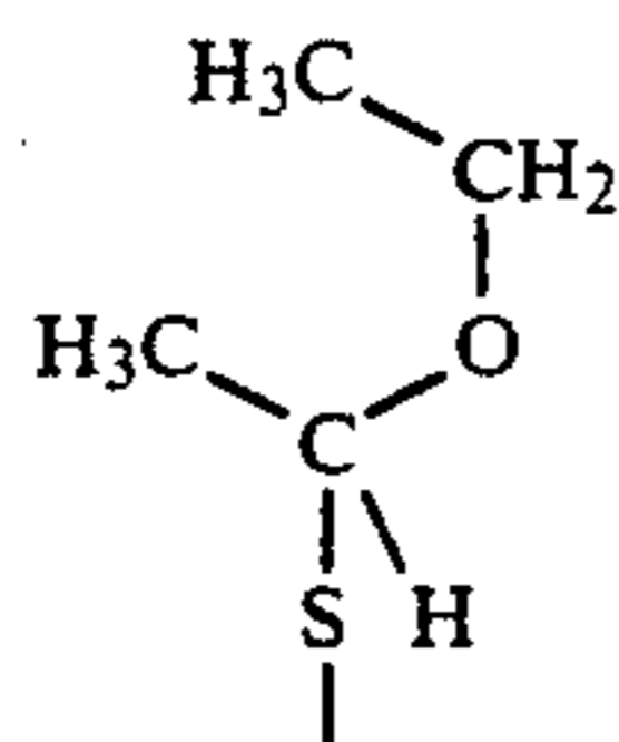
ethoxyethyl
