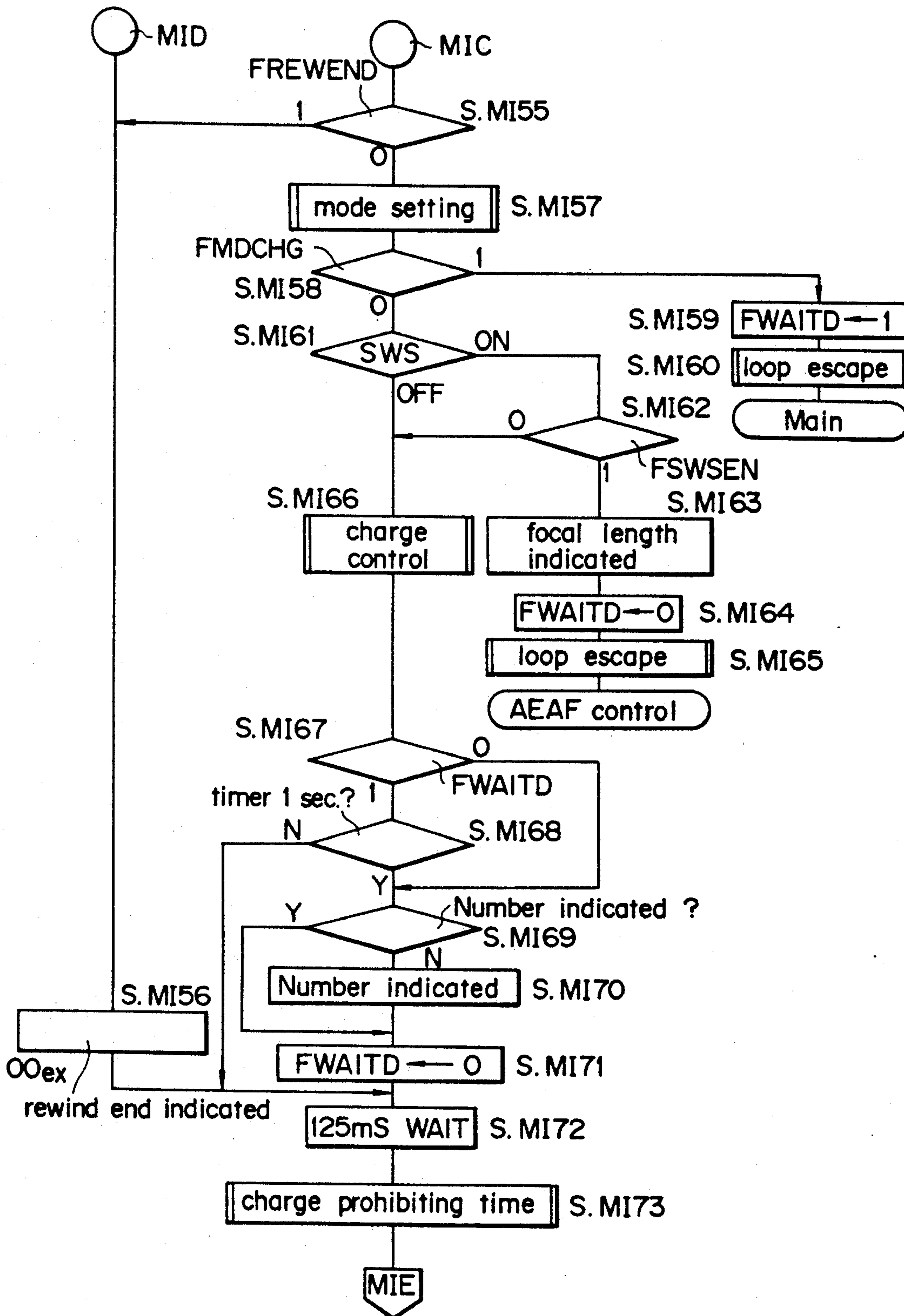
FIG. 15
