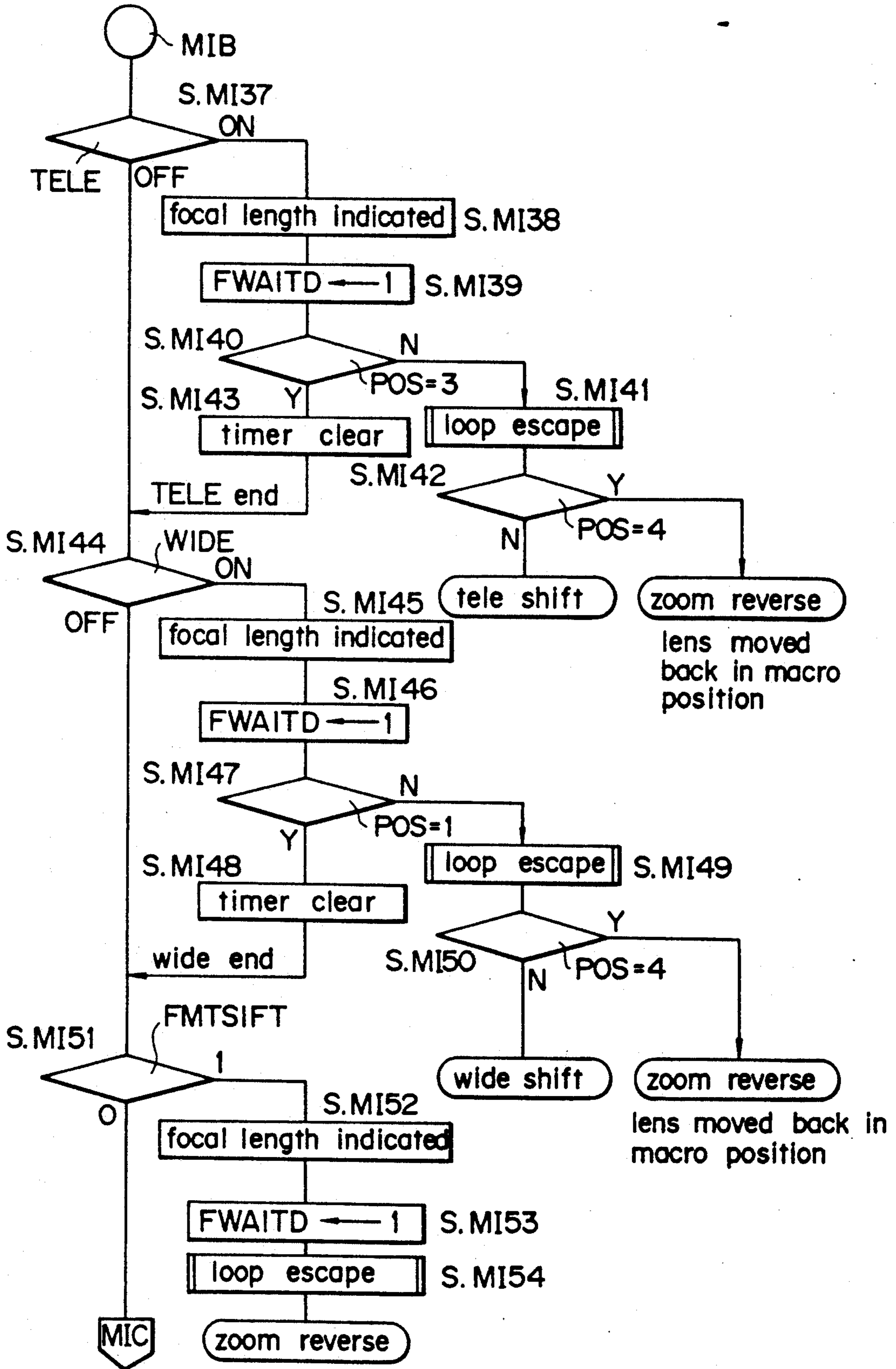
FIG. 14
