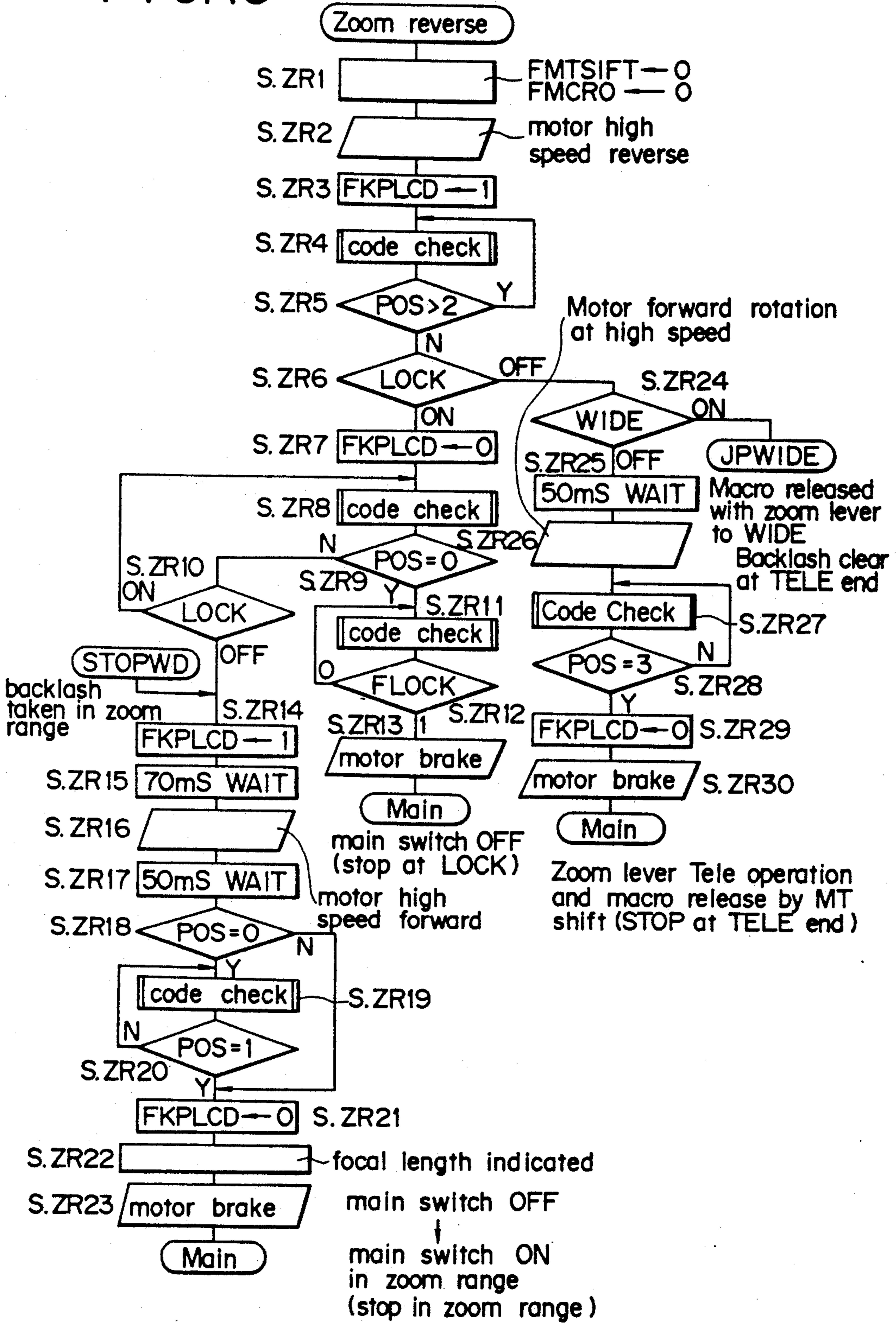
FIG. 19
