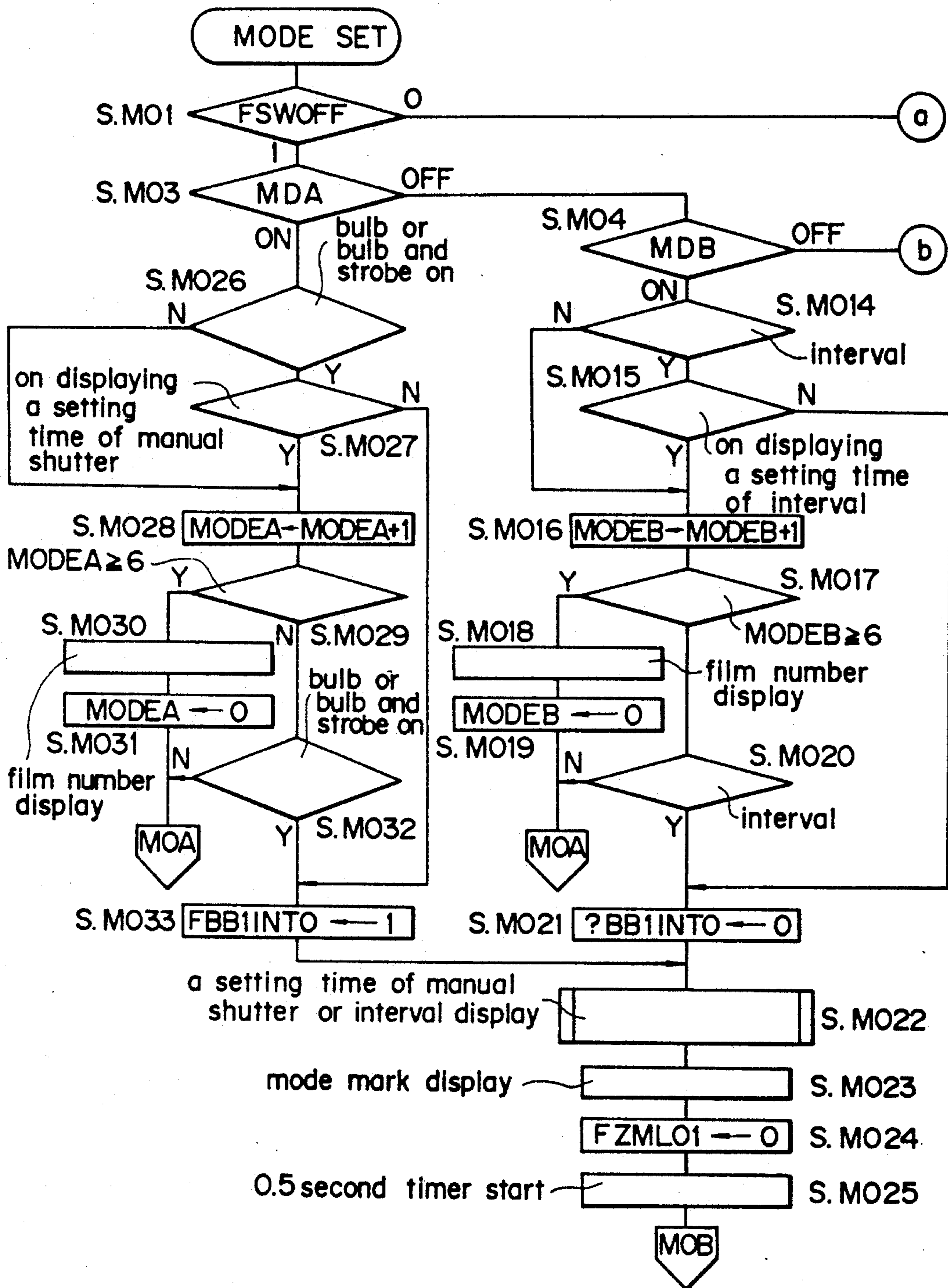
FIG. 25A
