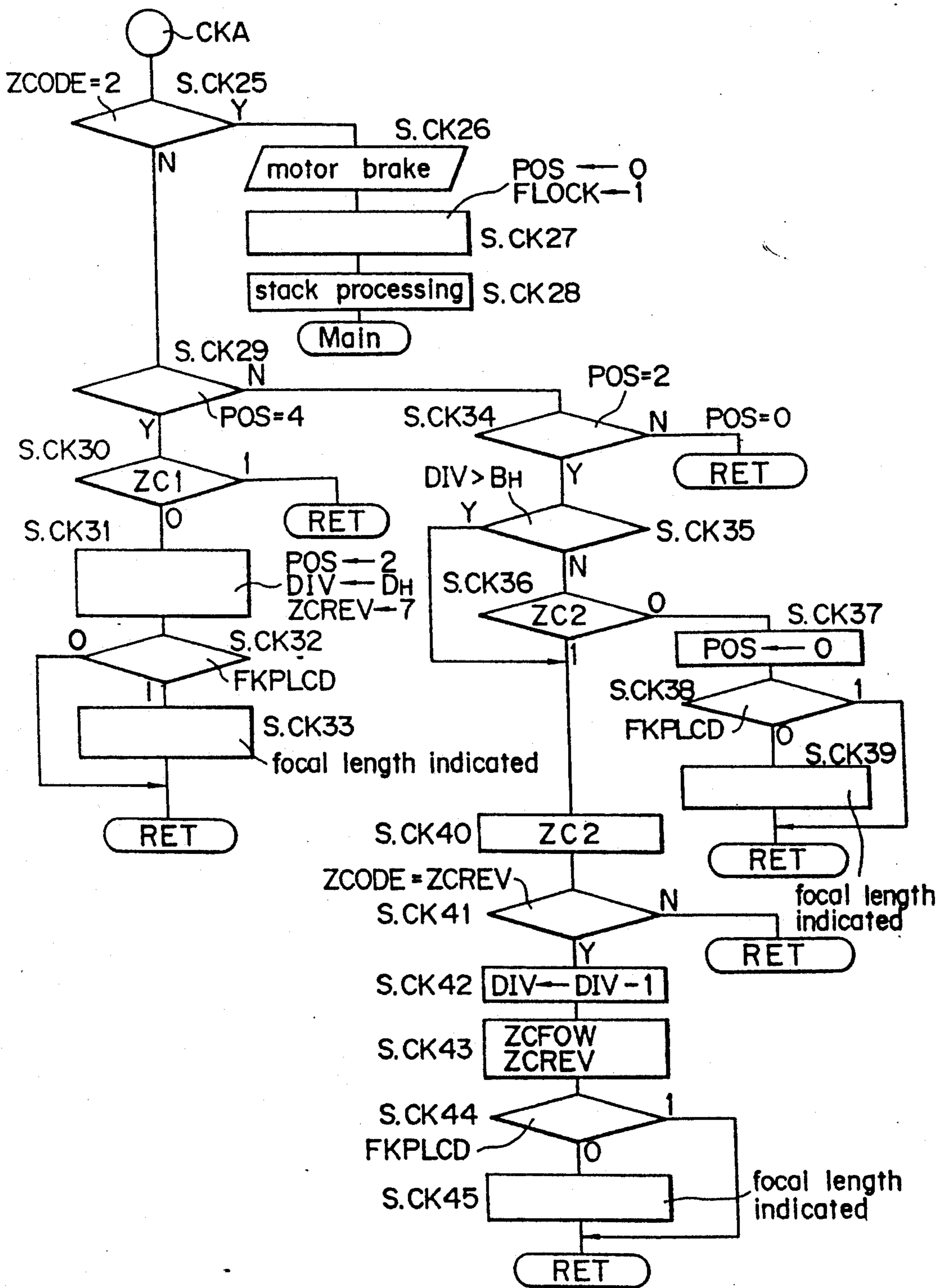
FIG. 18
