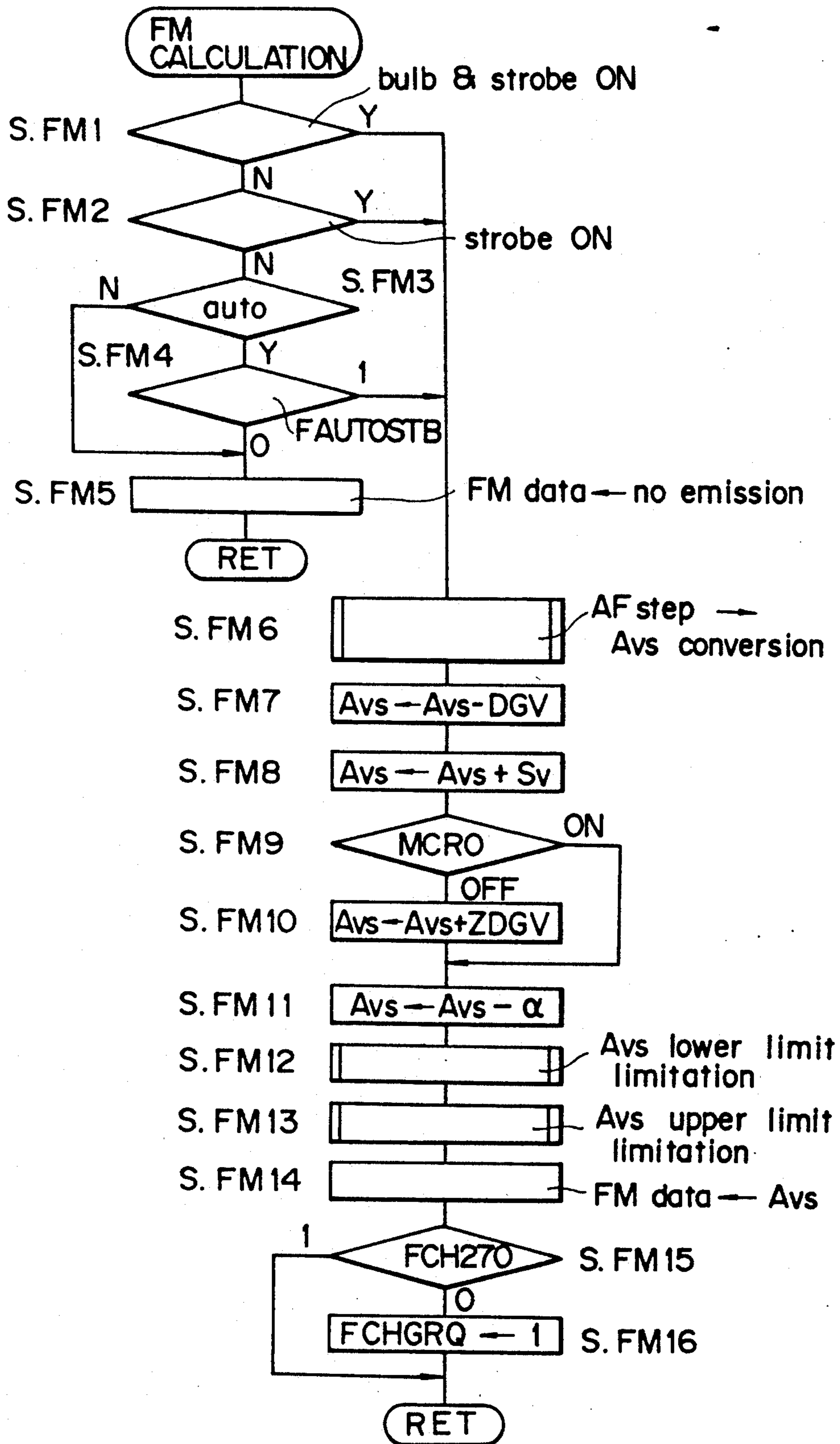
FIG. 34
