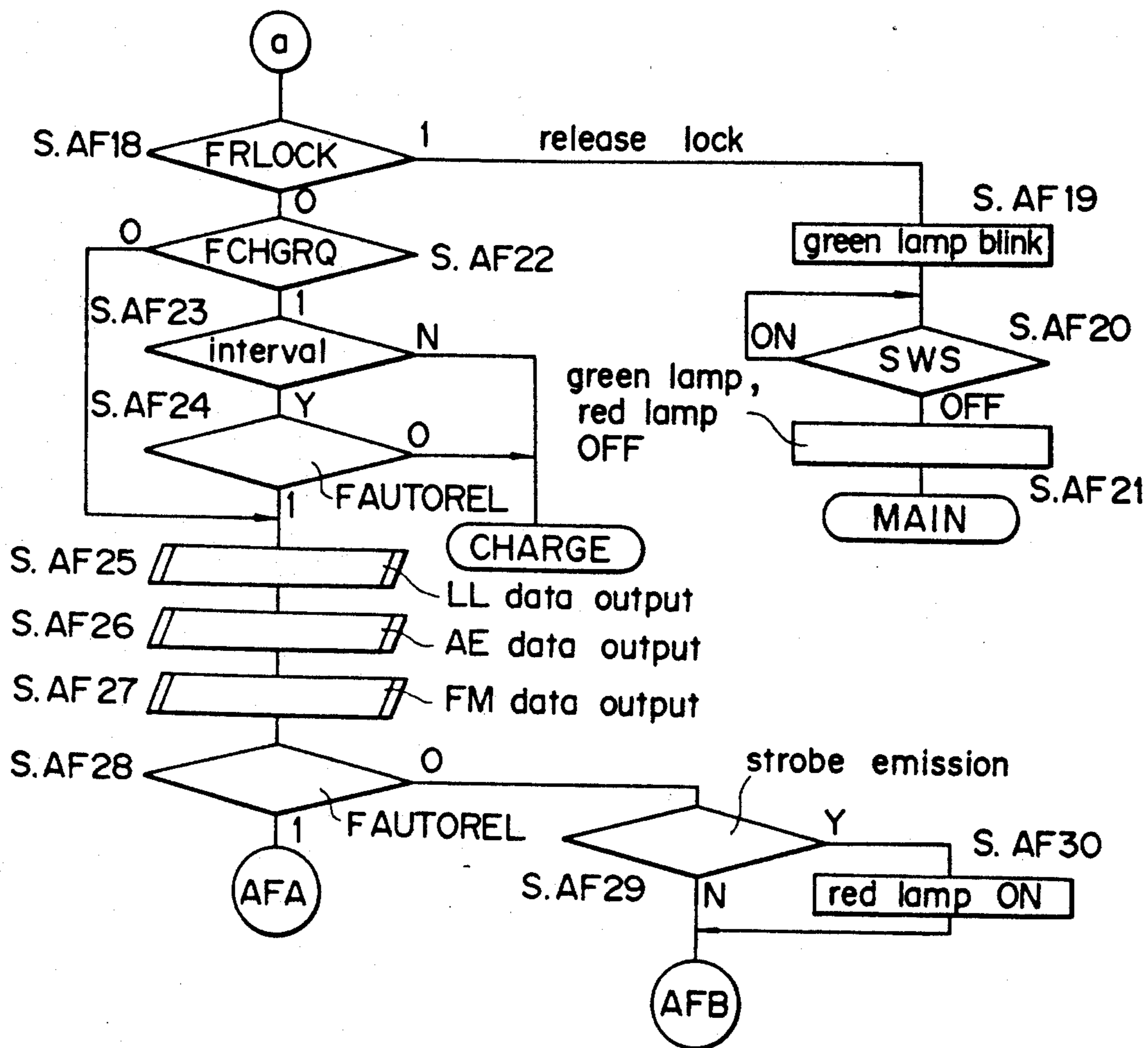
FIG. 29
