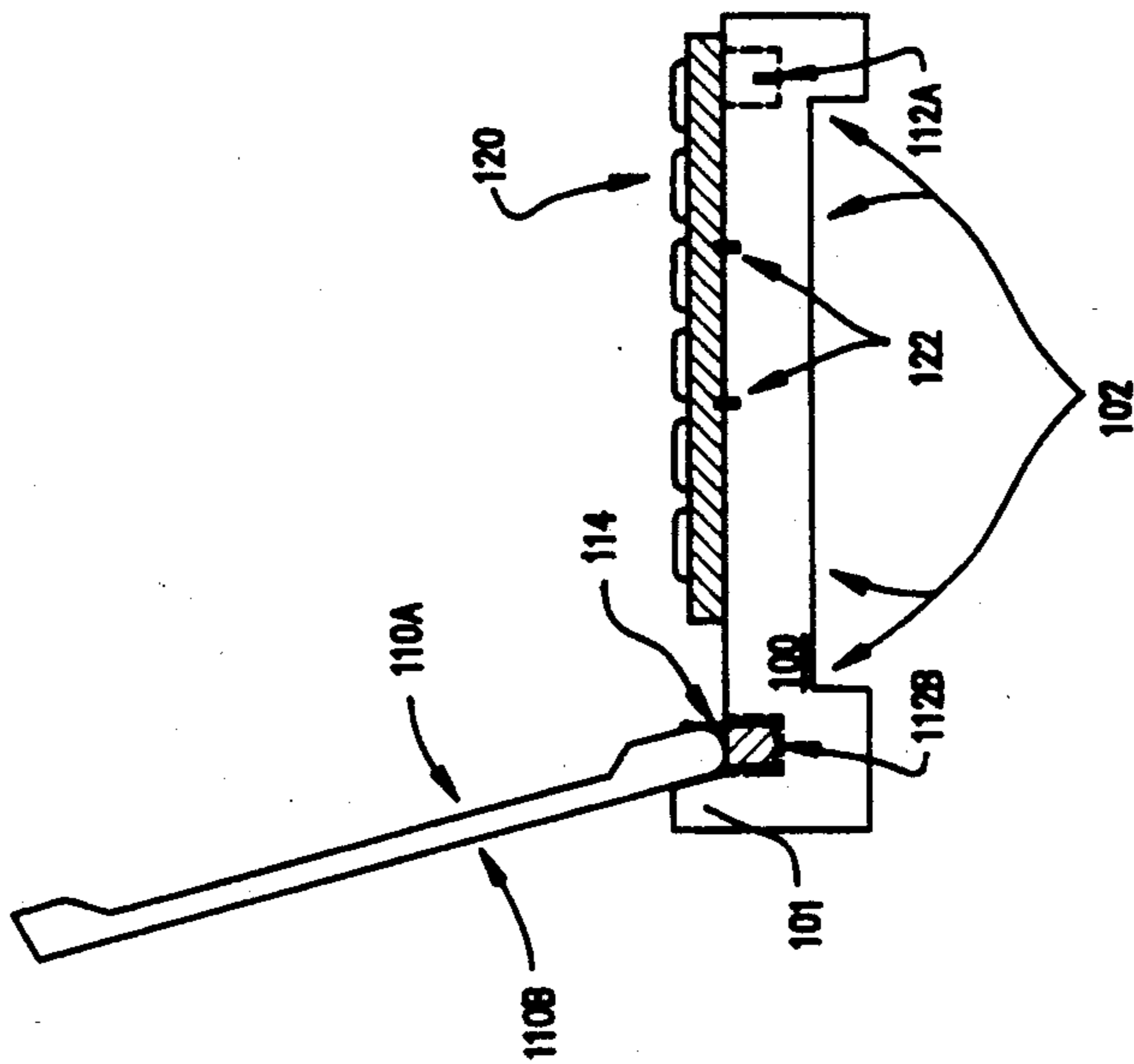
FIG. 1A TYPING POSITION
