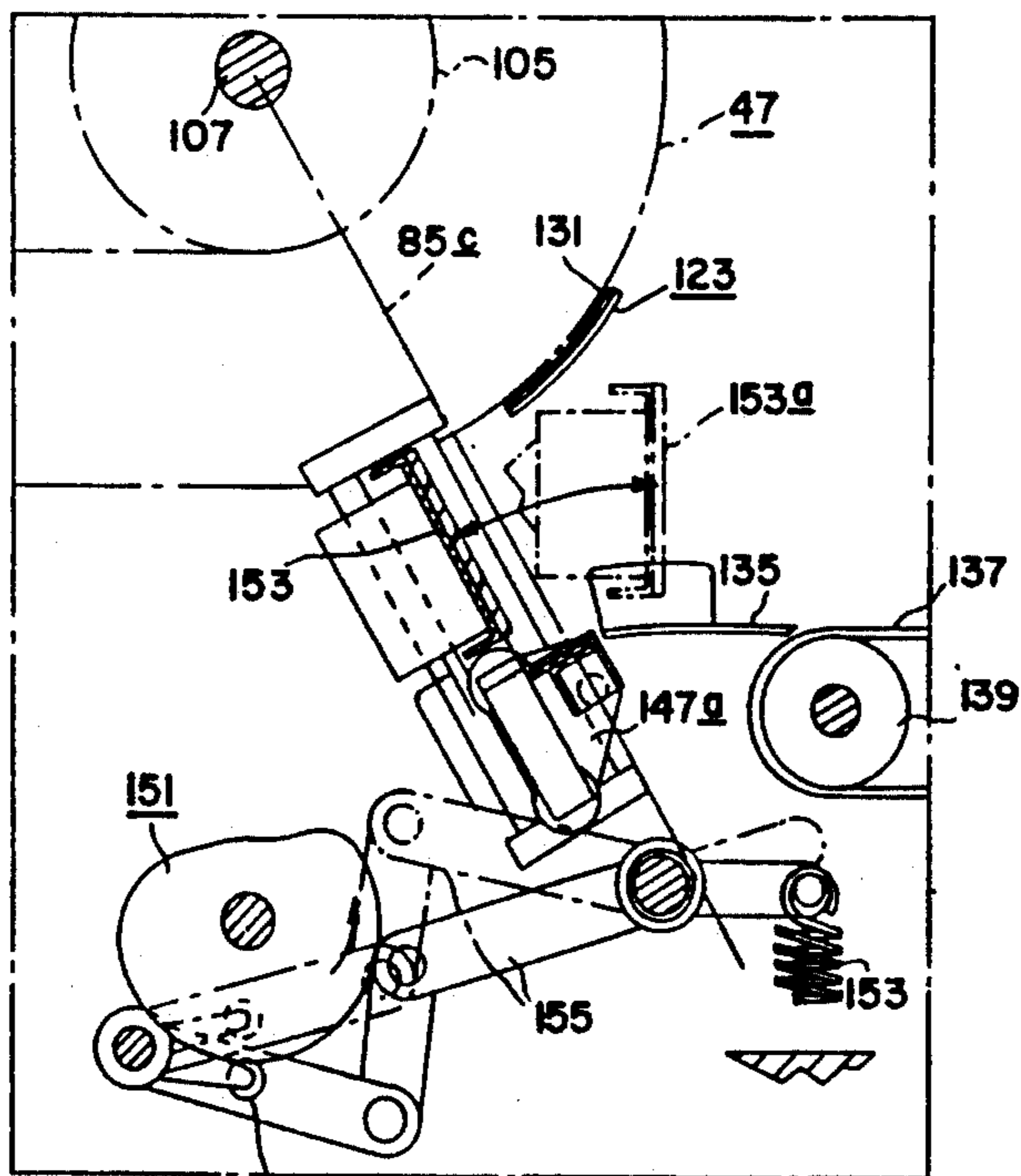
FIG. 5D (PUSHER CAM)
