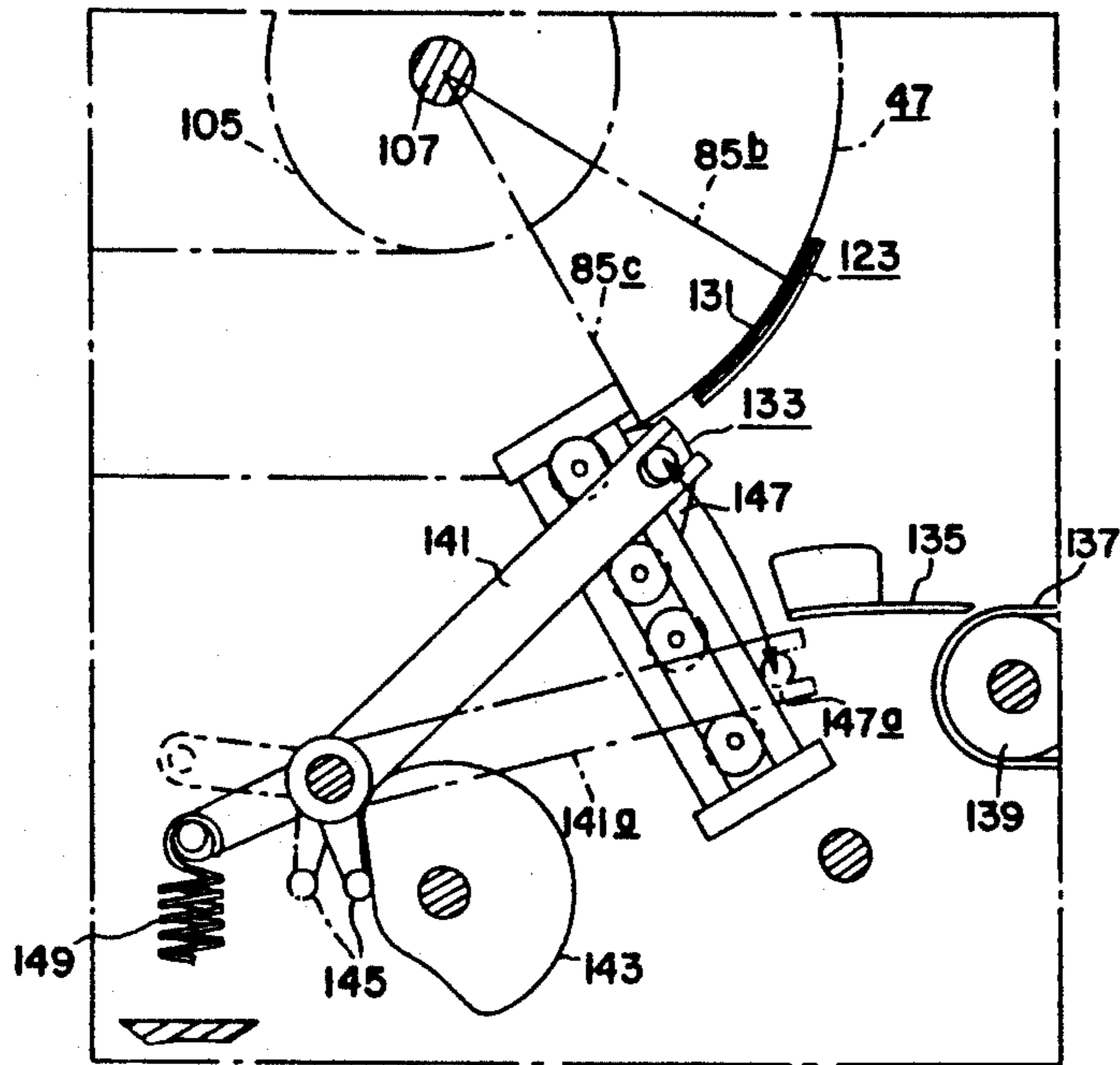
FIG. 5C (ELEVATOR CAM)
