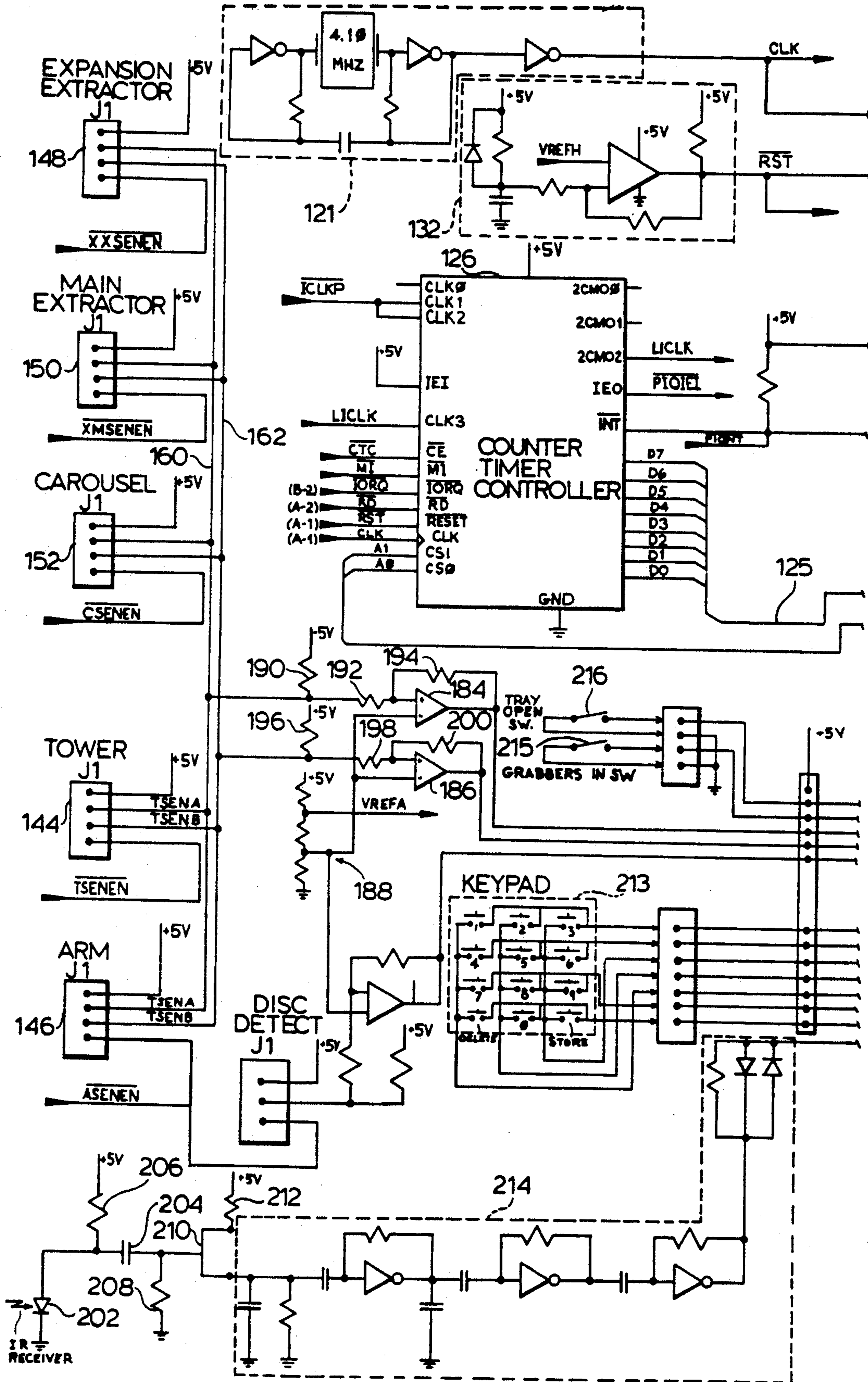
FIG.16A
