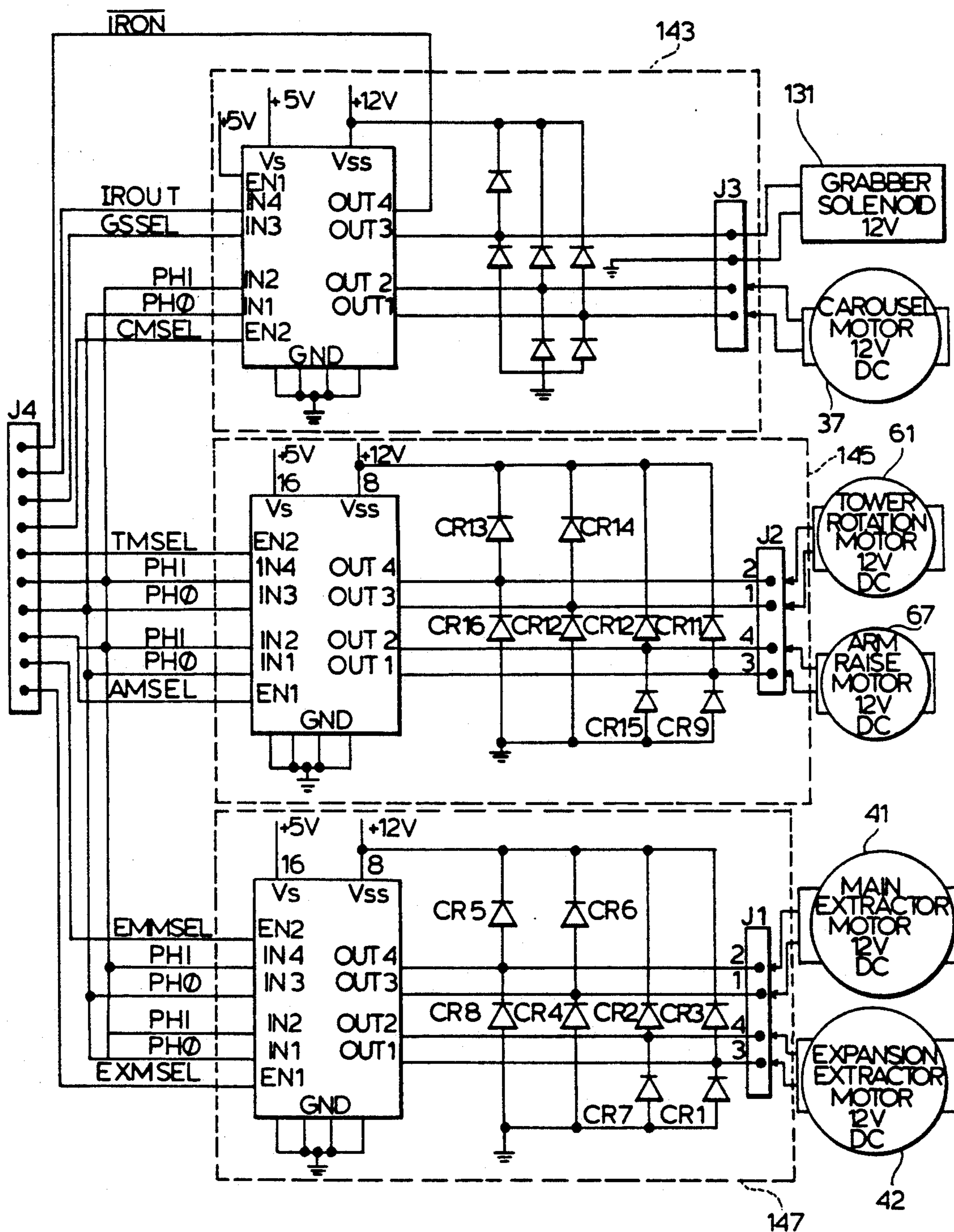
FIG. 18
