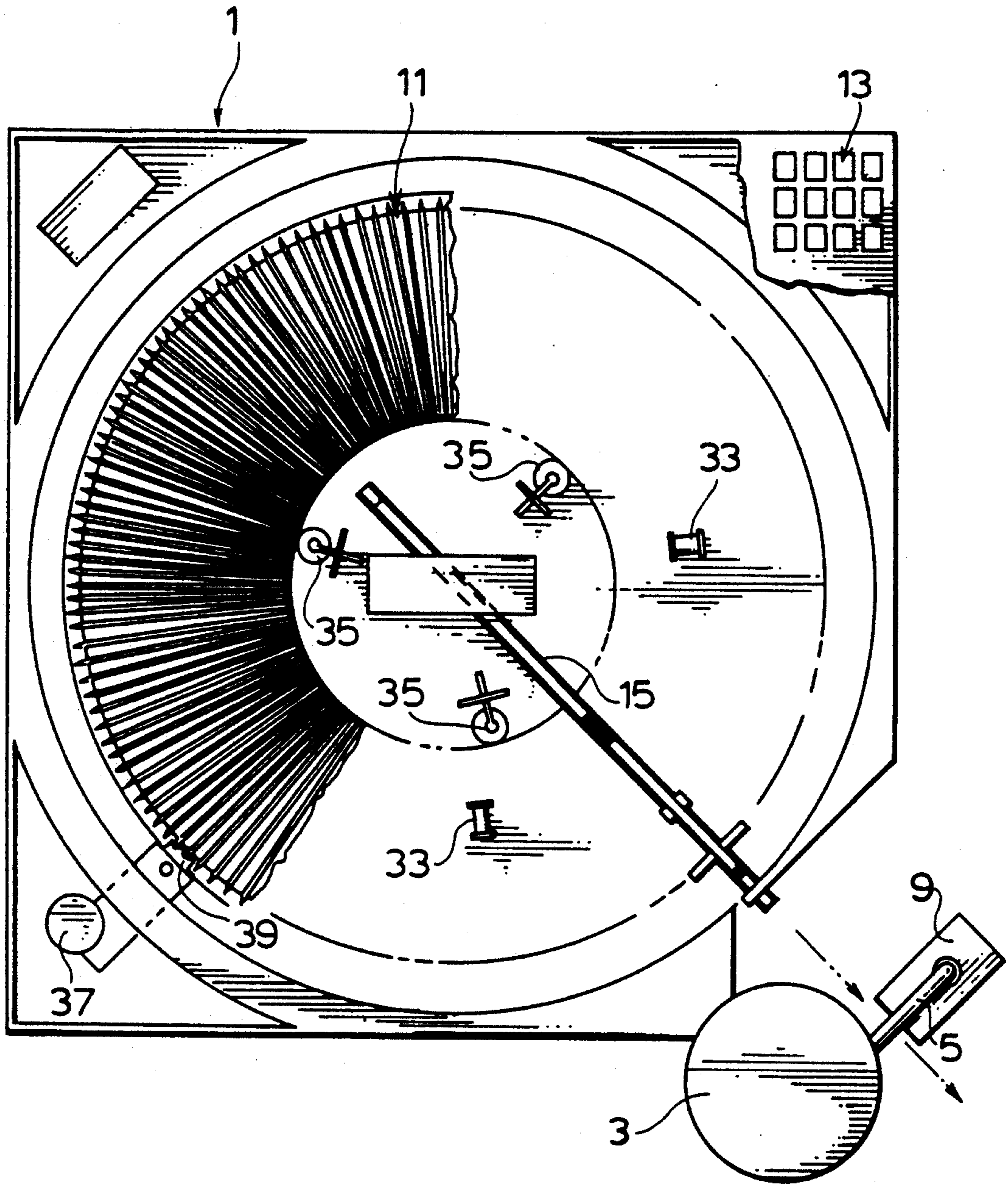
FIG. 4
