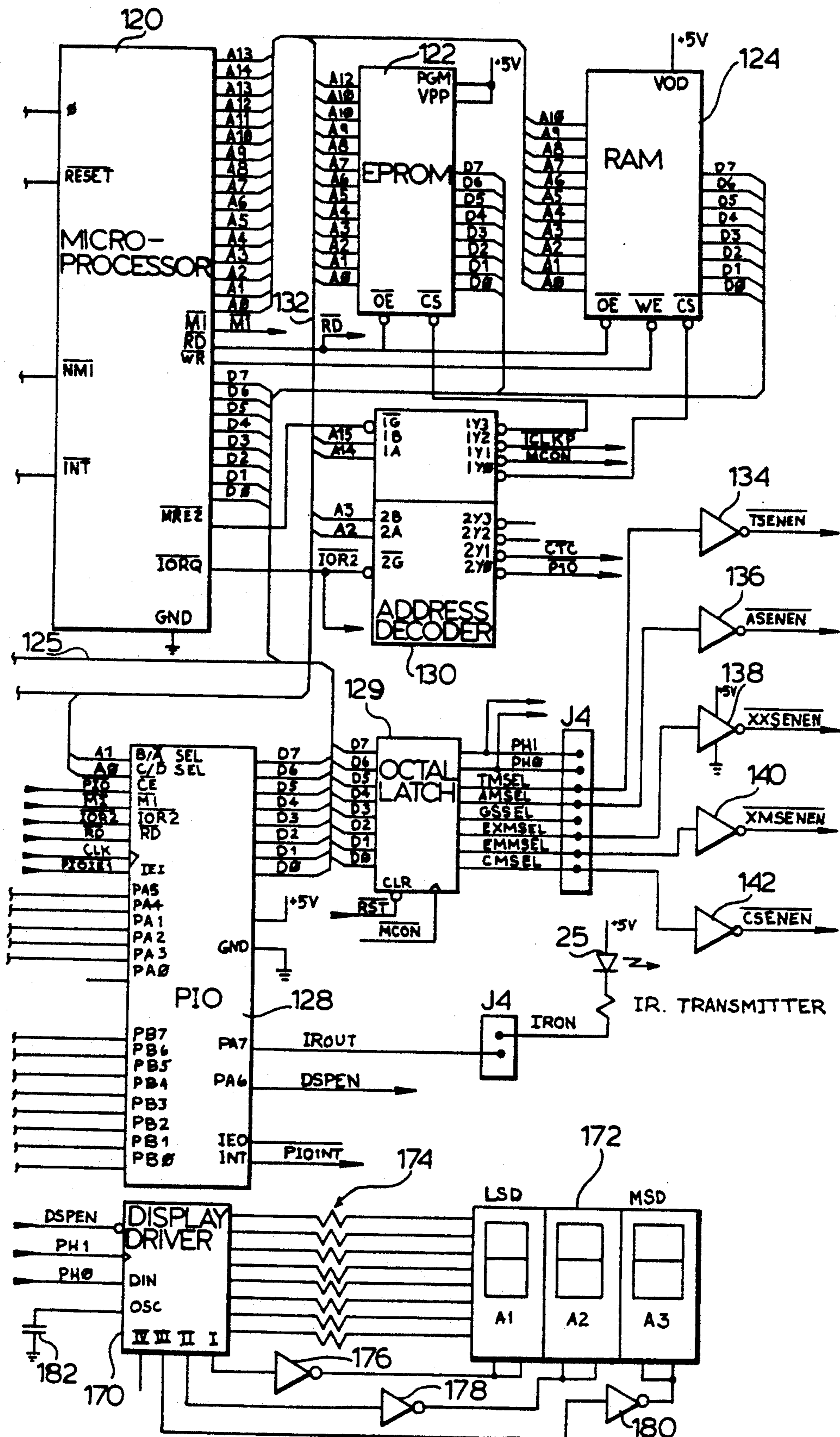
FIG. 16B
