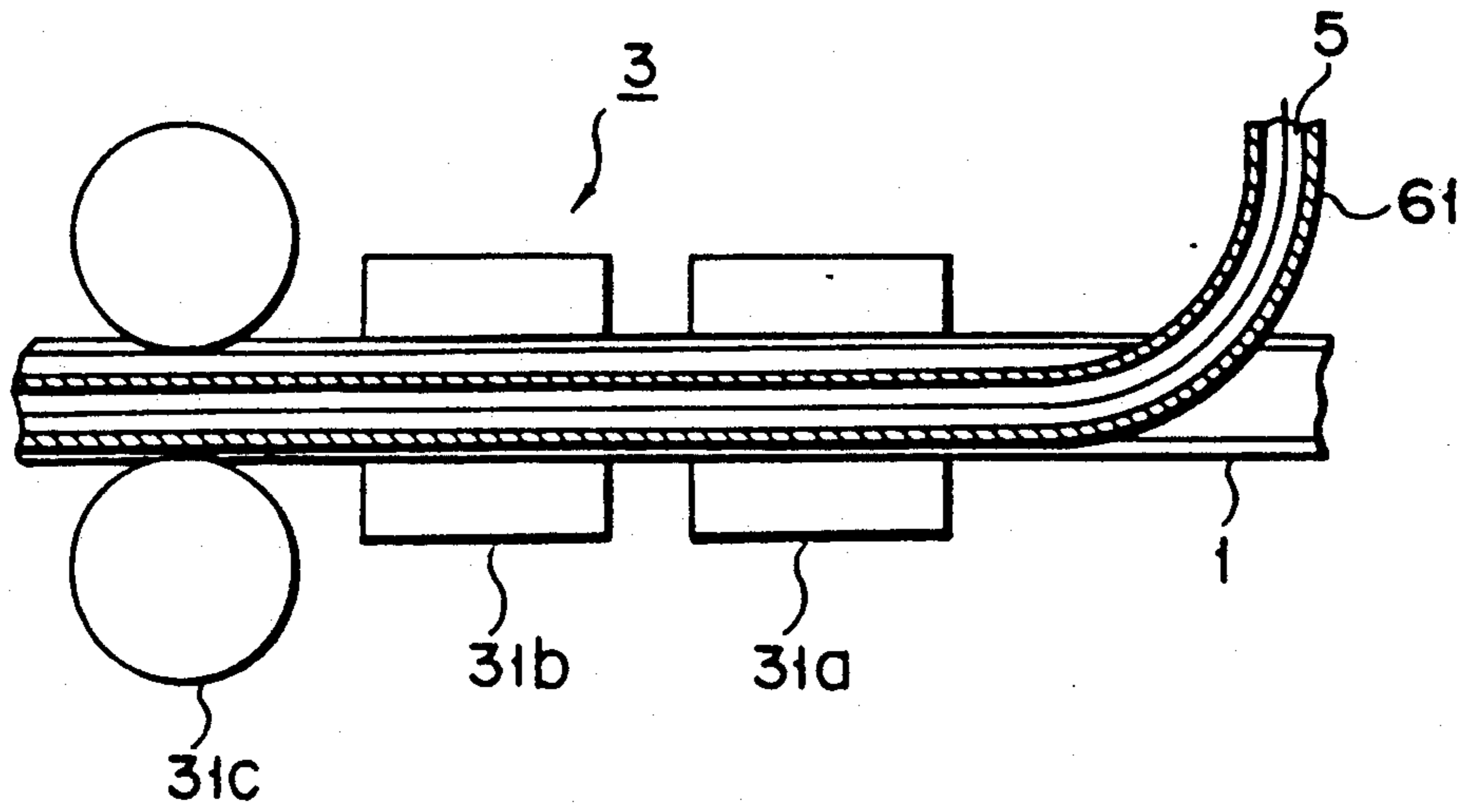
F I G. 18
