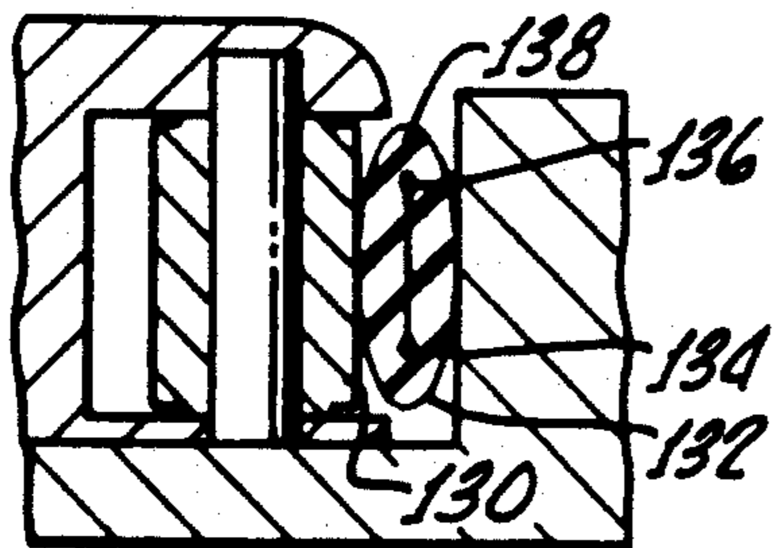
FIG. 5a. (PRIOR ART)
