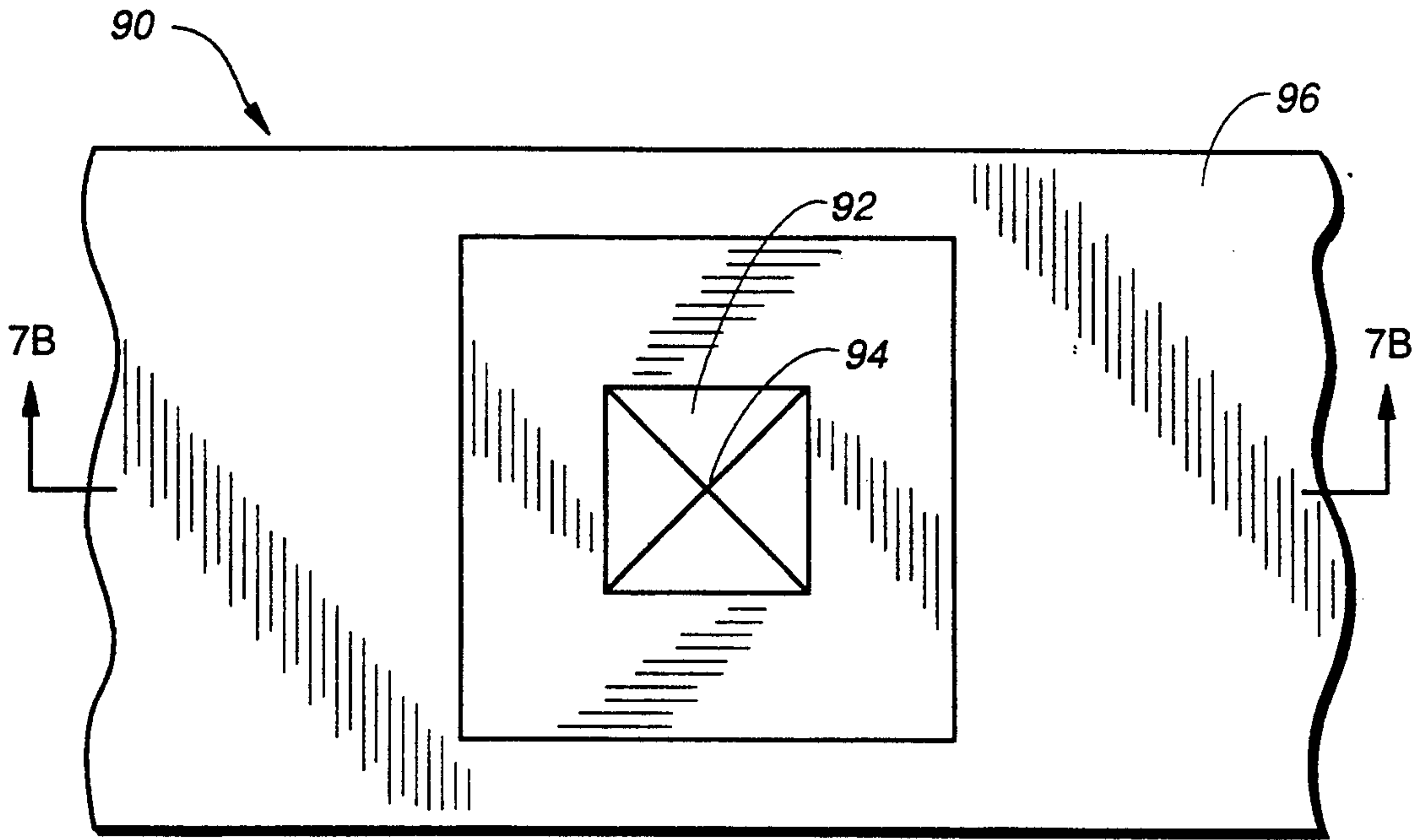
FIG. 7A
