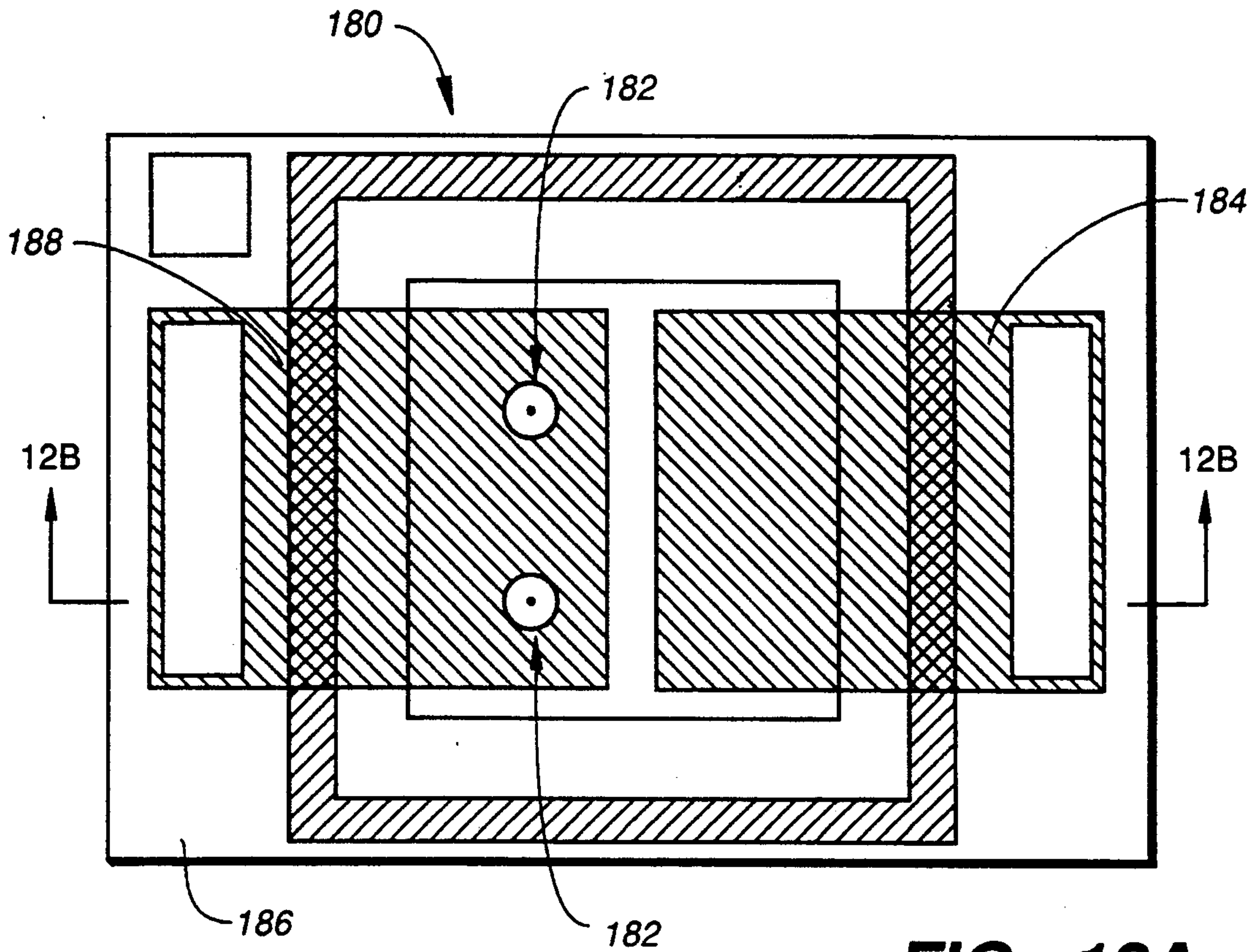
FIG. 12A
