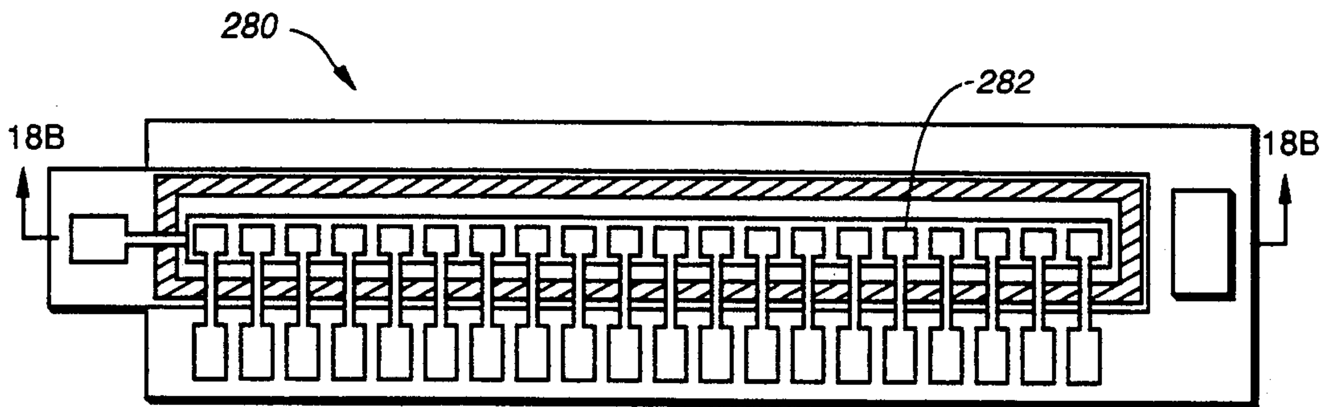
FIG. 18A
