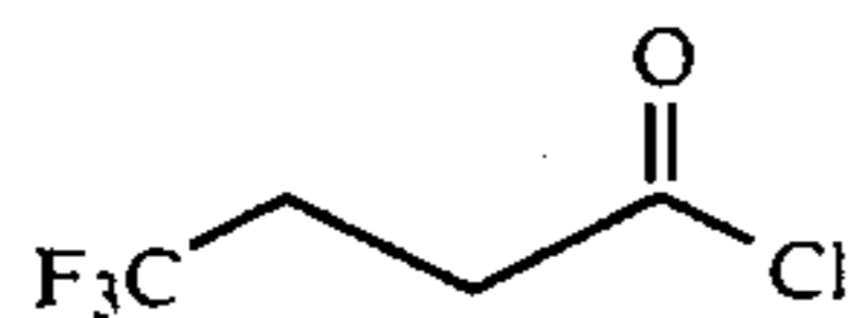
4,4,4-Trifluorobutanoyl chloride
