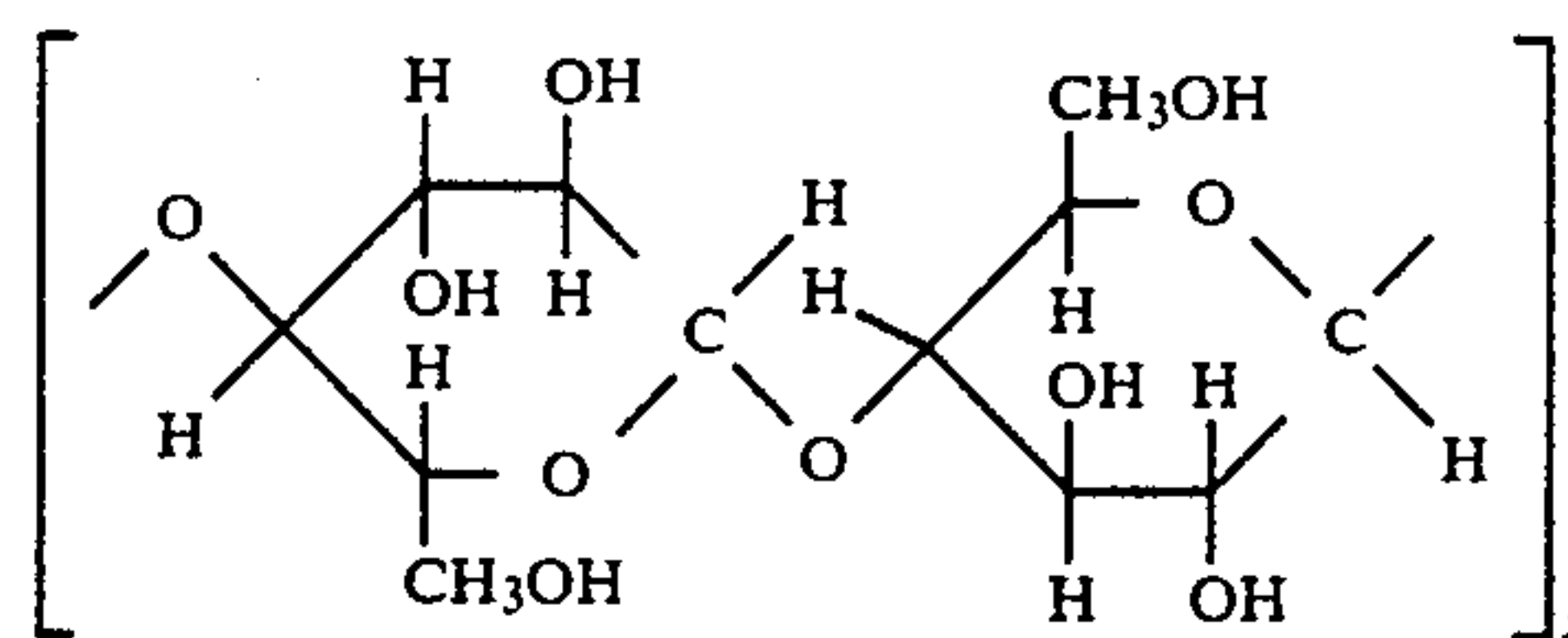
Cellulose
