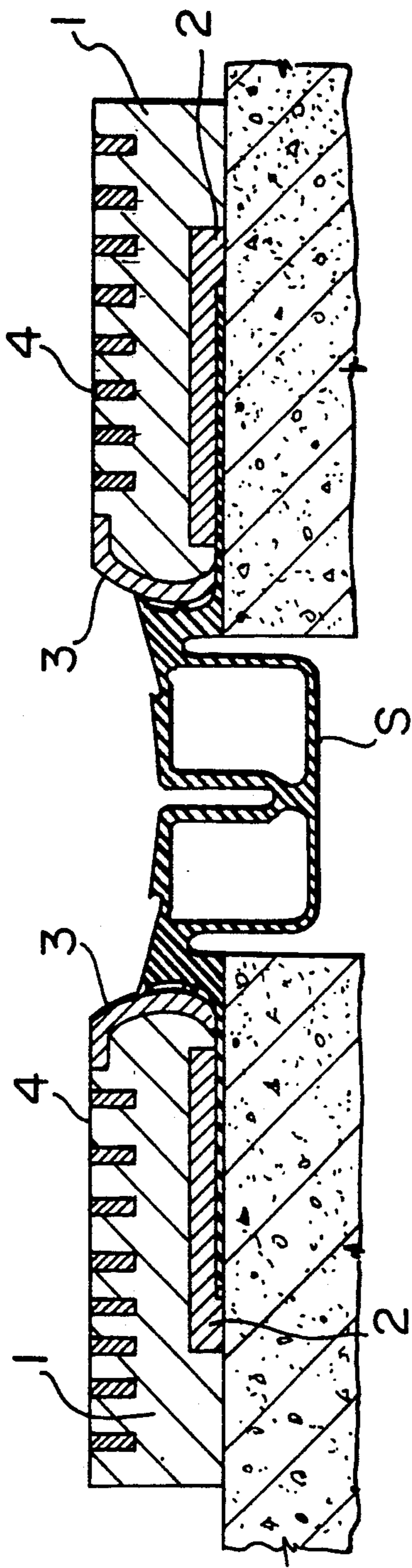
FIG. 3
