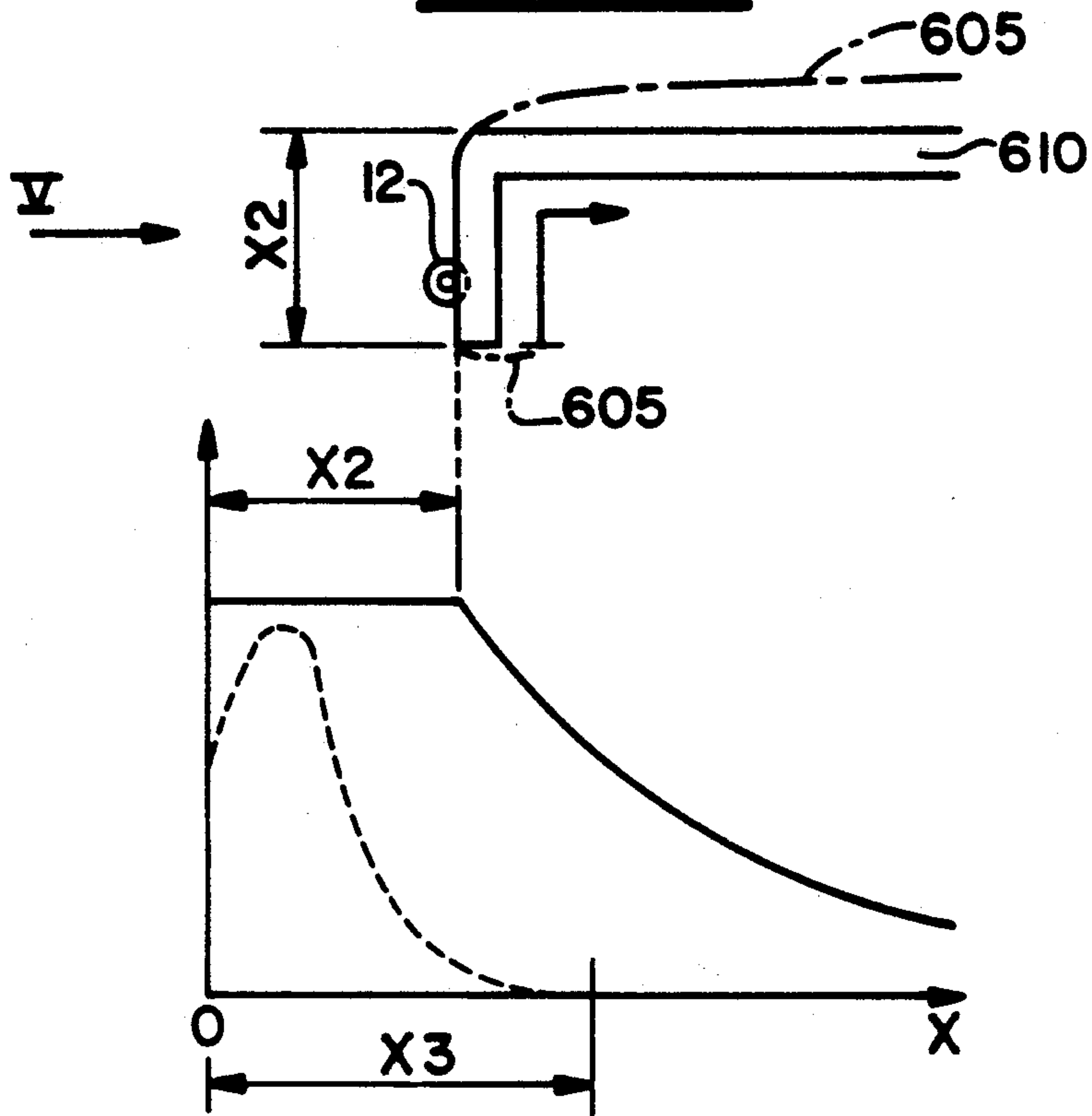
FIG. 24
