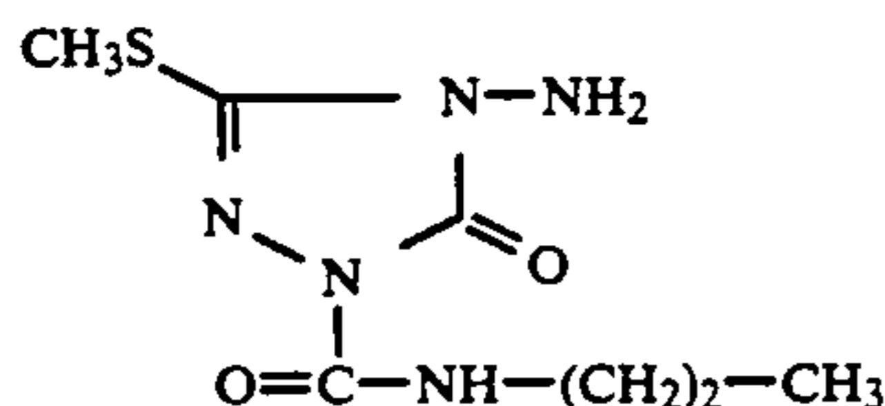
(D) 4-amino-1-(N-propylcarbamoyl)-3-methylthio-(1H,4H)-1,2,4-triazolin-5-one
