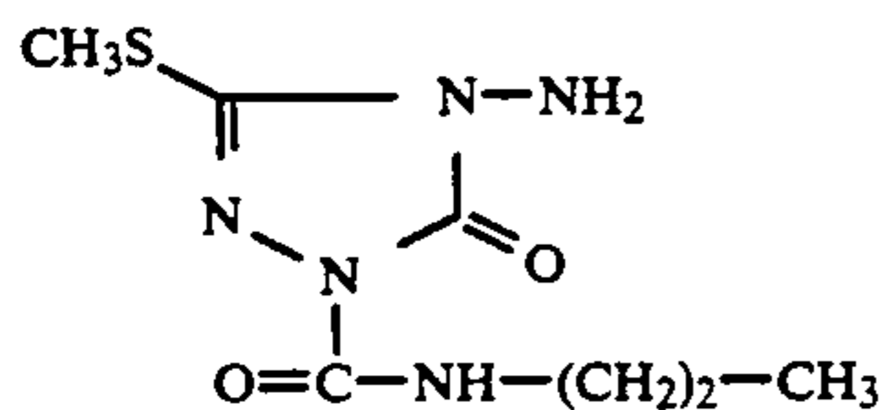
(D) 4-amino-1-(N-propylcarbamoyl)-3-methylthio-(1H,4H)-1,2,4-triazolin-5-one
