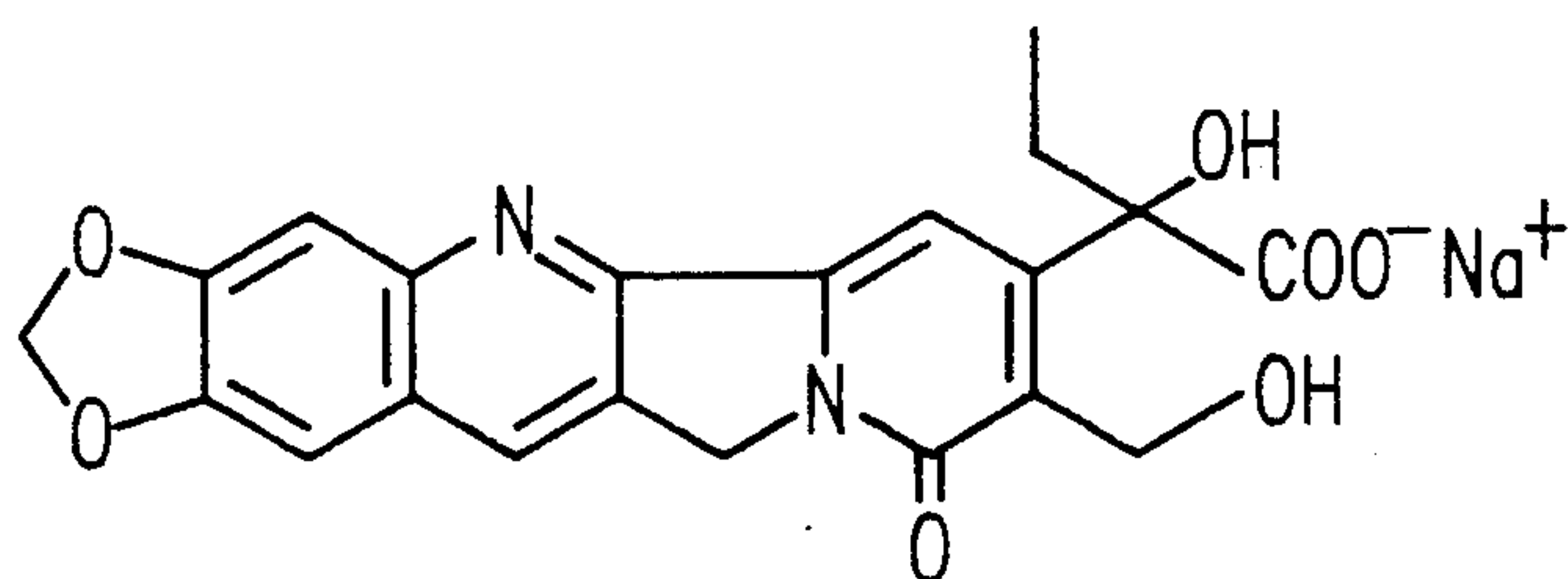
10-11-MDO-20(RS)-CPT-SODIUM SALT
