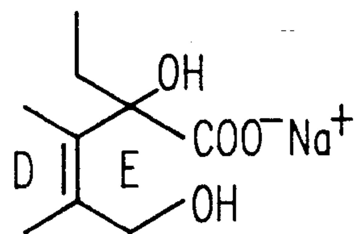
CPT-SODIUM SALT
