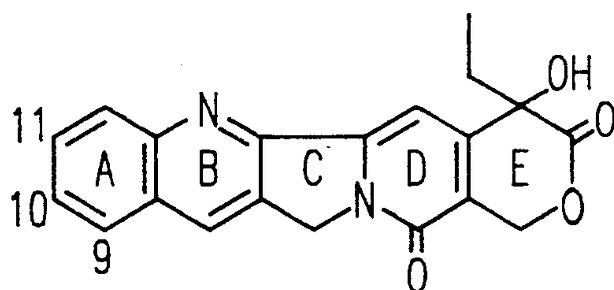
CAMPTOTHECIN (CPT)
