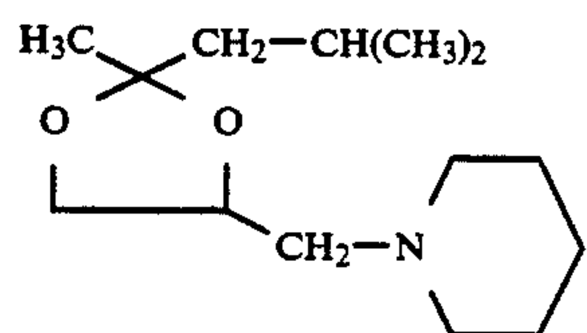
2-isobutyl-2-methyl-4-(1-piperidinylmethyl)-1,3-dioxolane
