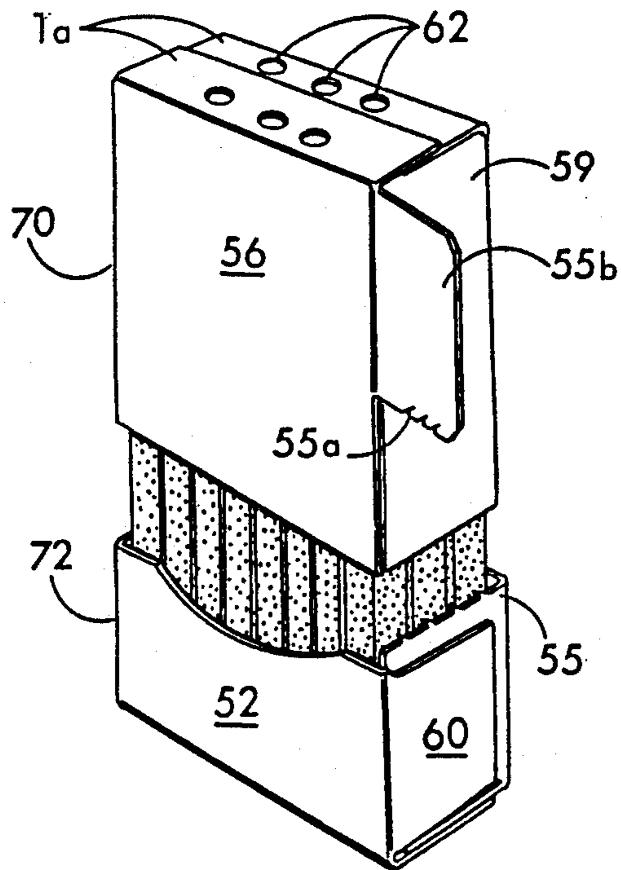
FIG. 19
