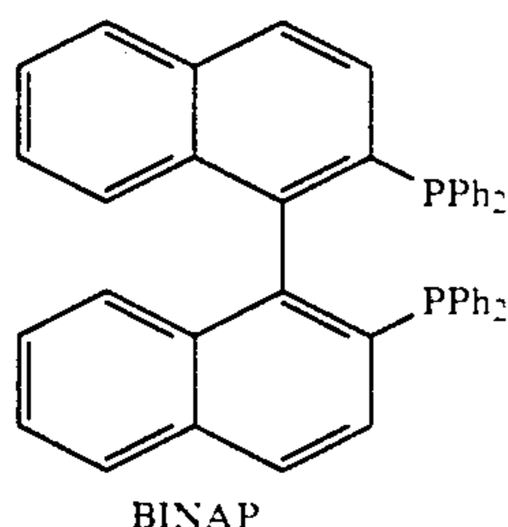
BINAP
