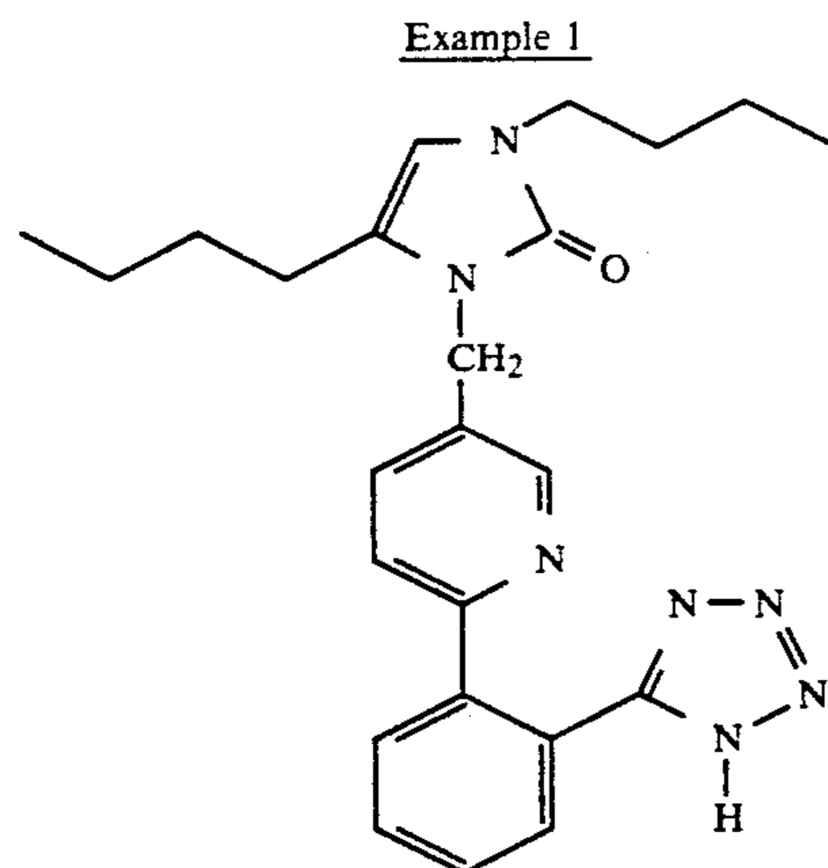
1,4-dibutyl-1,3-dihydro-3-[[6-[2-(1H-tetrazol-5-yl)phenyl]-3-pyridinyl]methyl]-2H-imidazol-2-one
