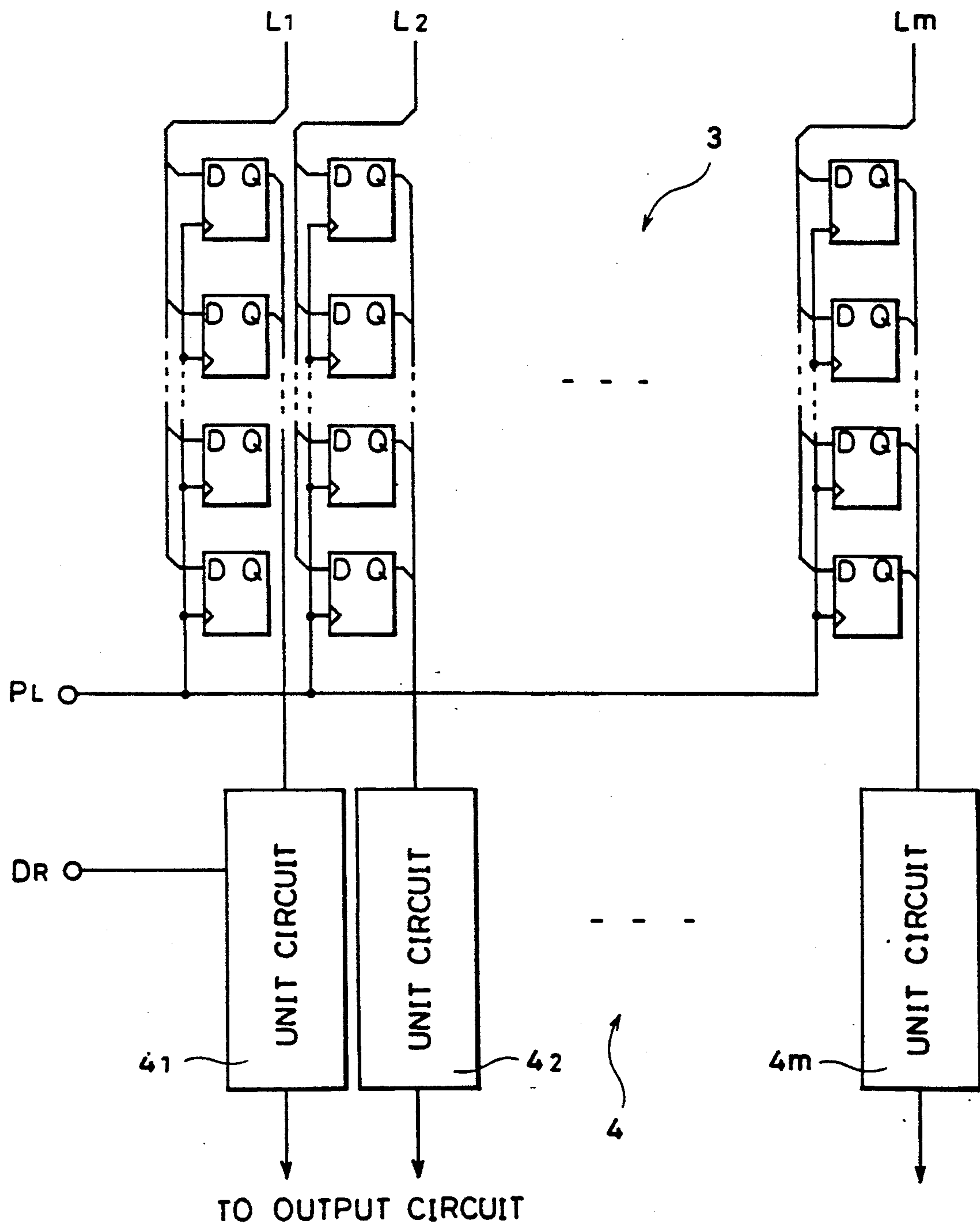
FIG. 2B
