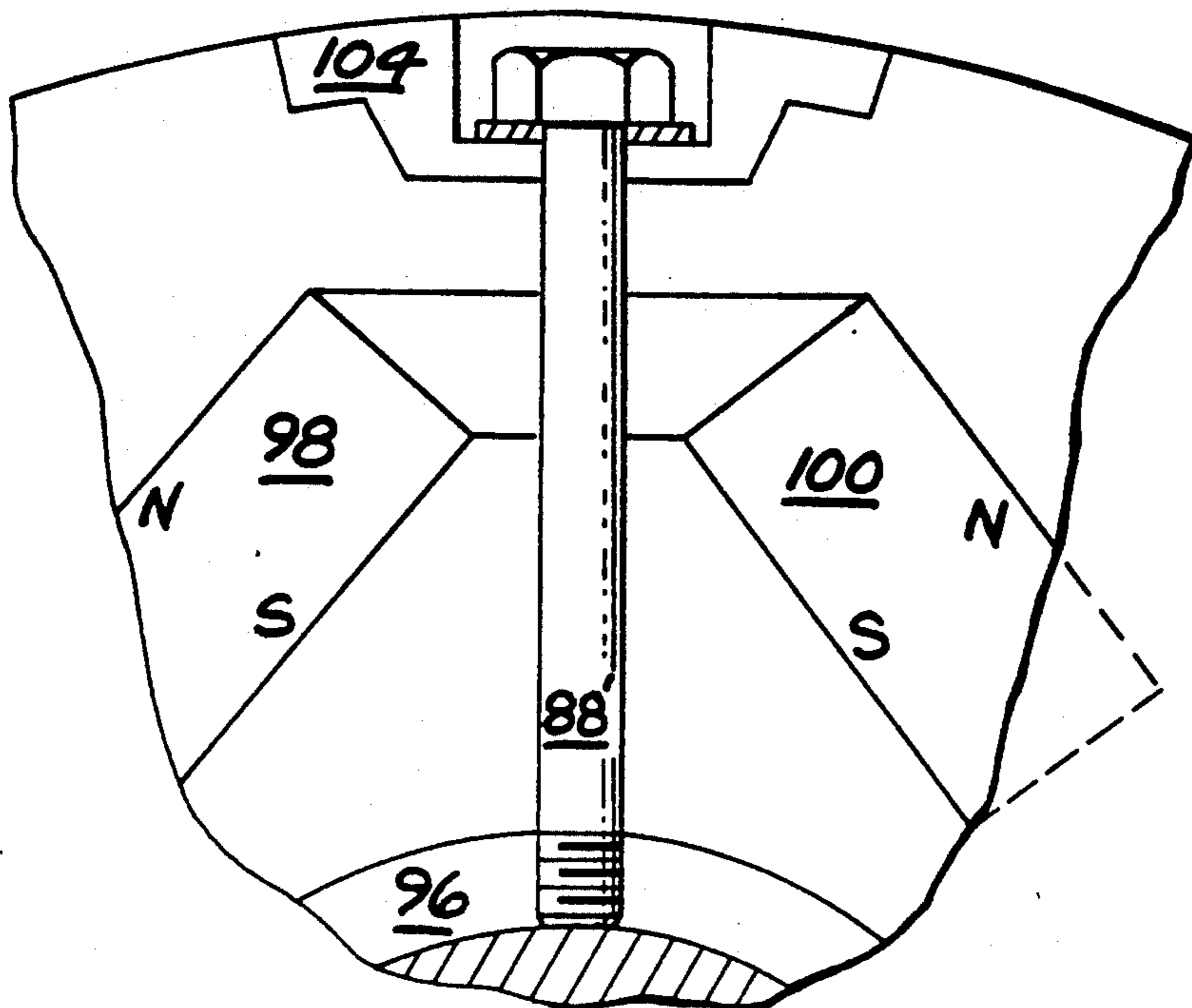
FIG. 7B
