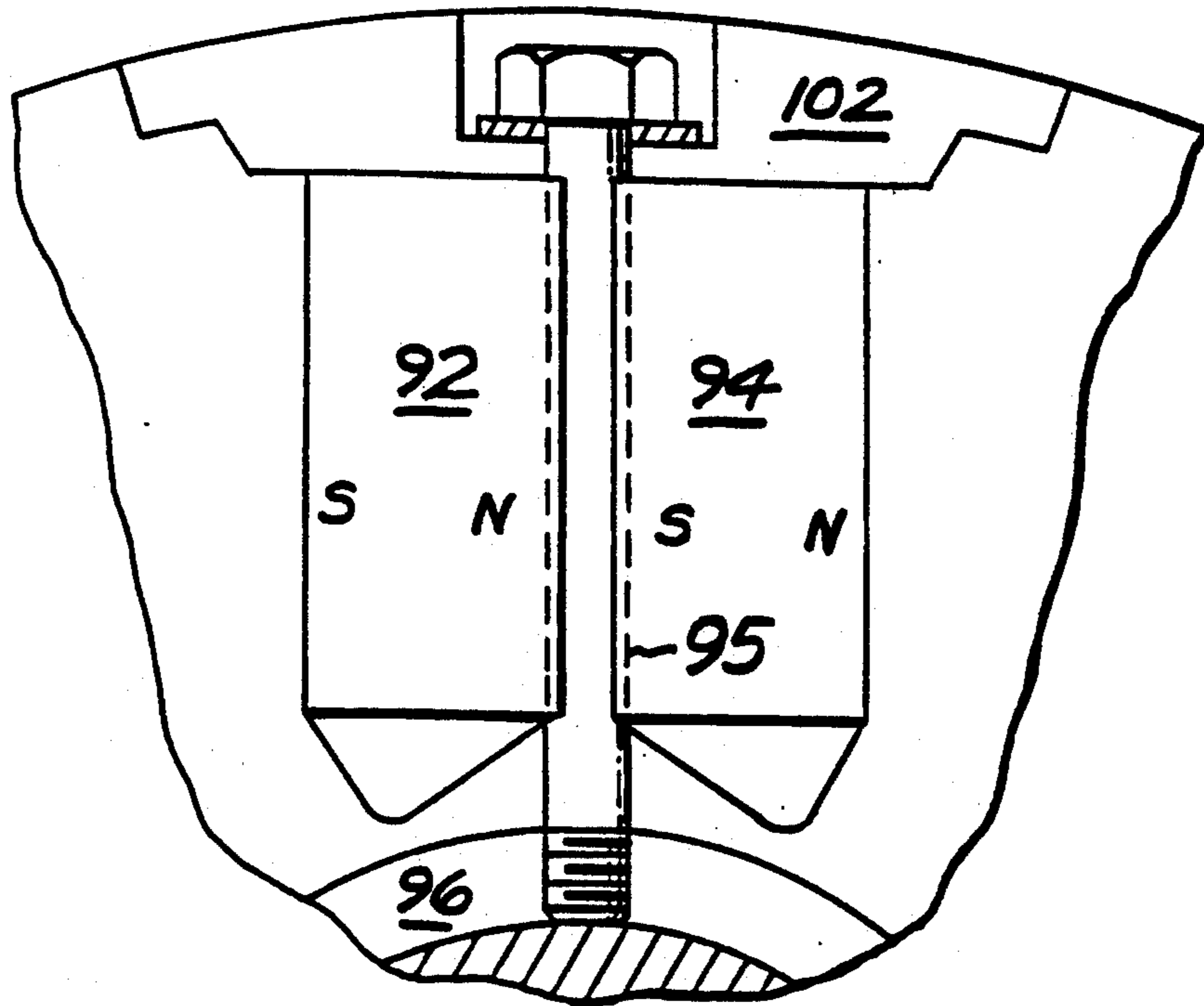
FIG. 7D
