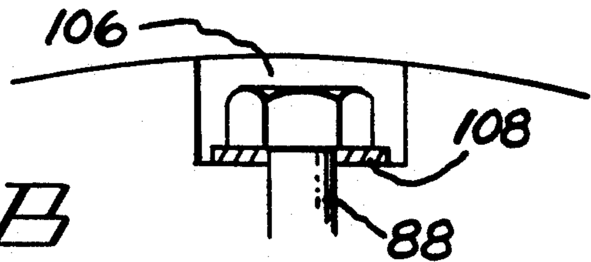
FIG. 7C
