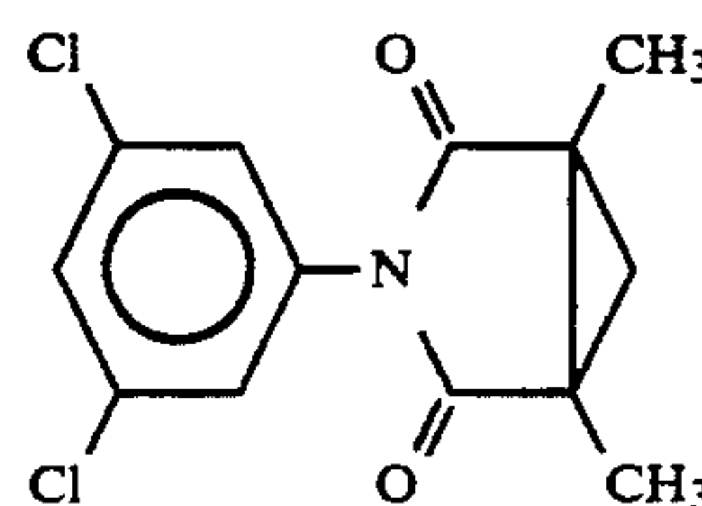
(PROCYMIDONE)
