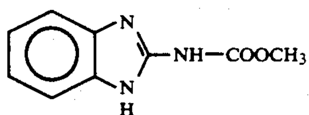
(CARBENDAZIM)
