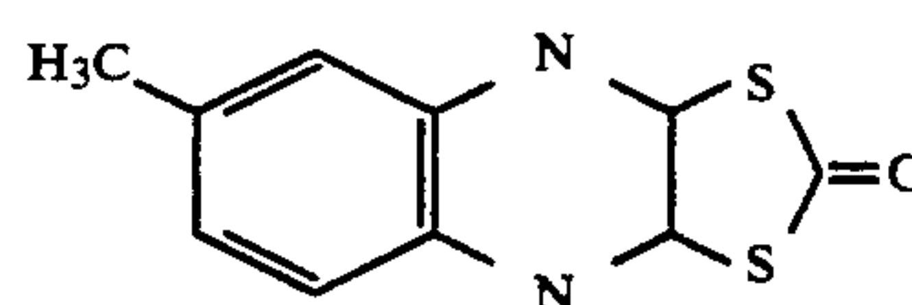
(QUINOMETHIONATE)
