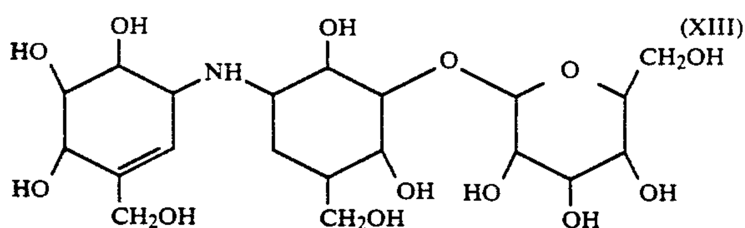
(VALIDAMYCIN)
