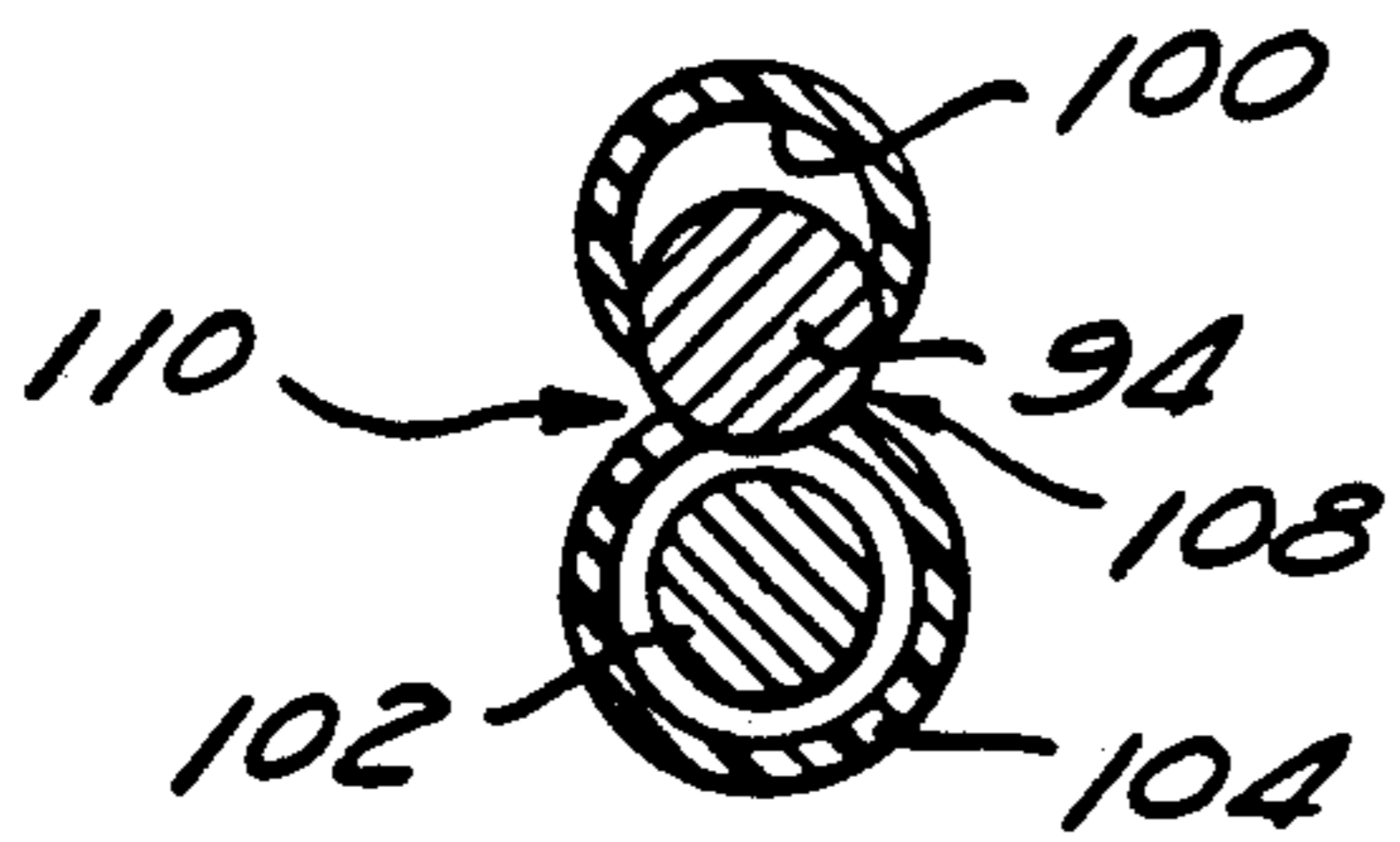
Fig. 13a
