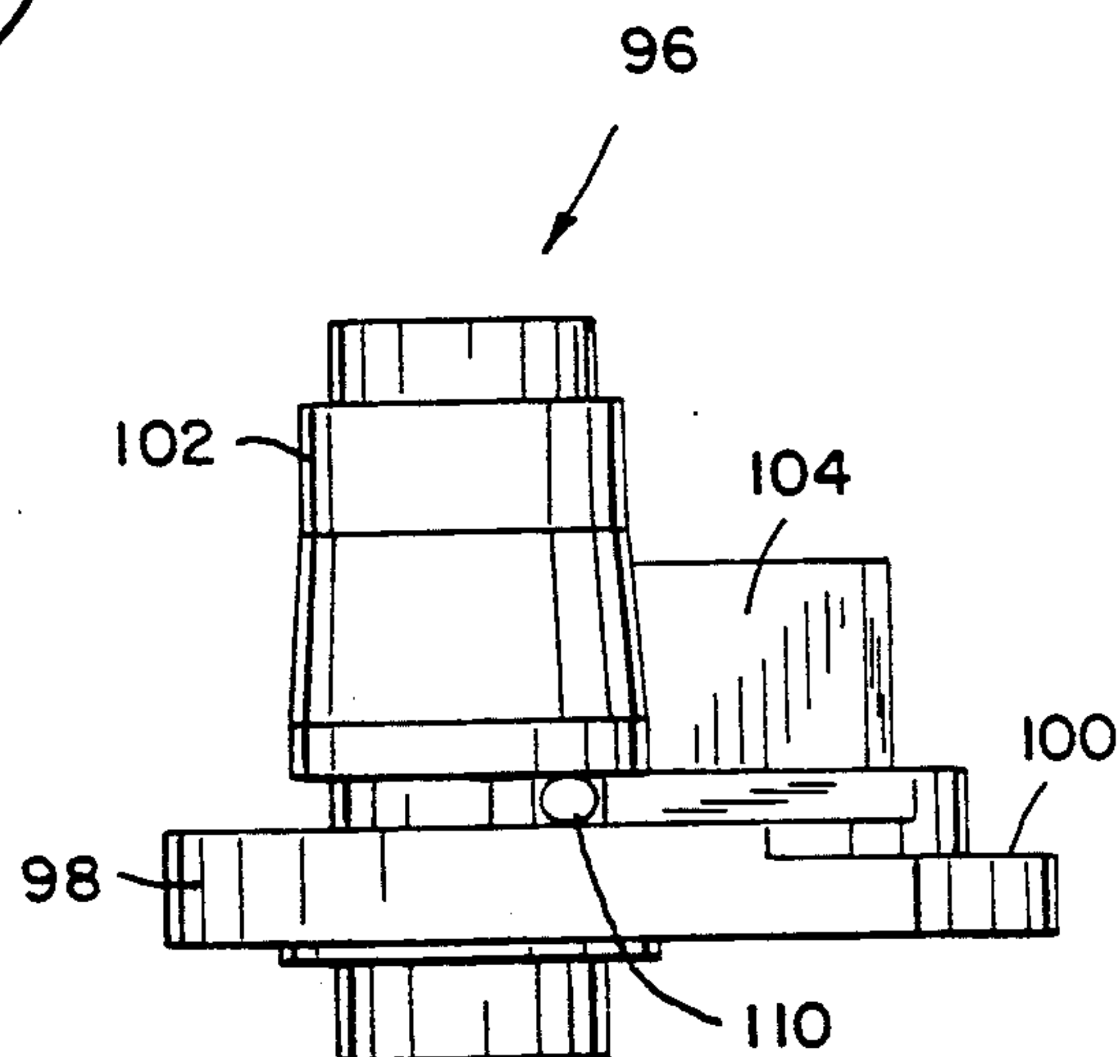
FIG. 12
