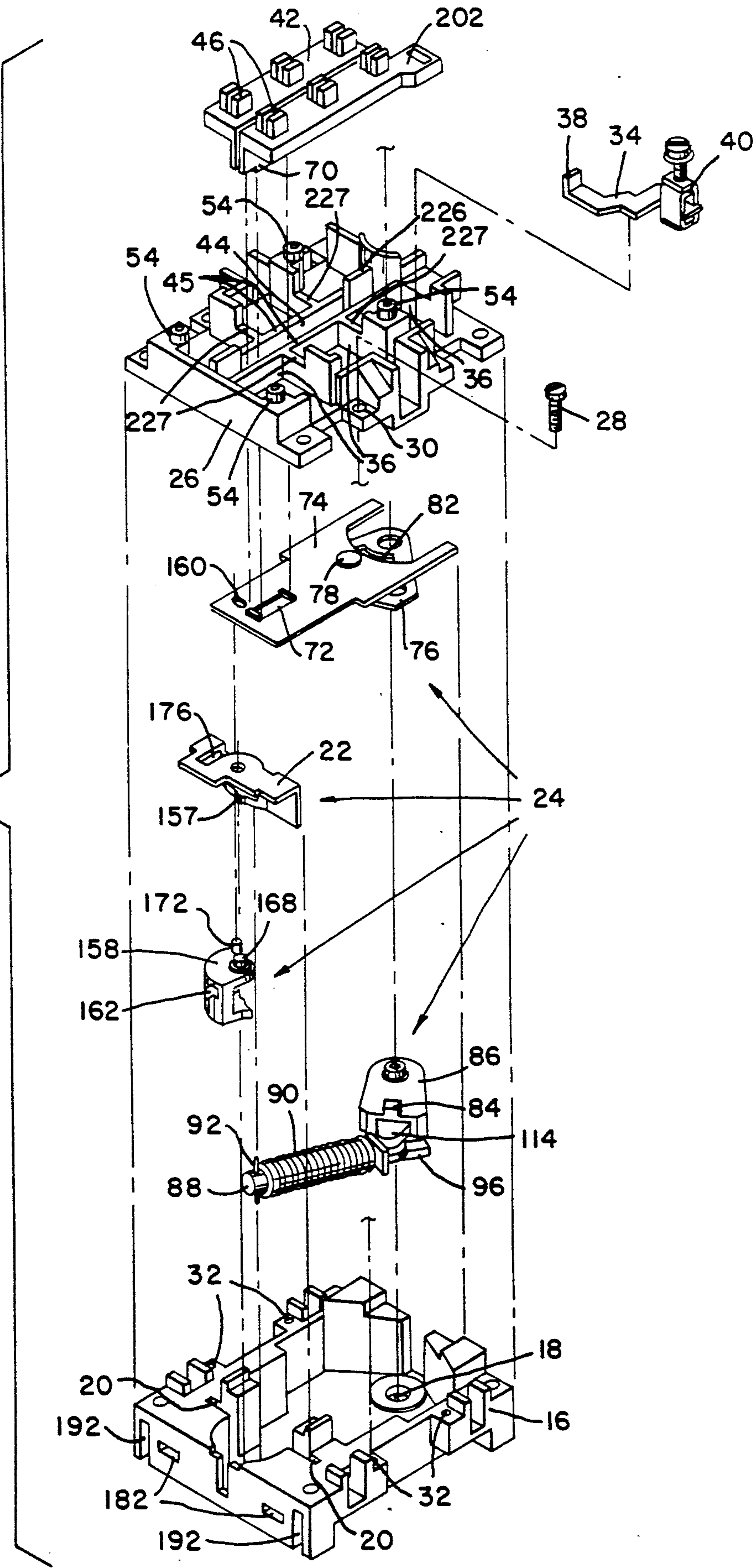
FIG. 2B
