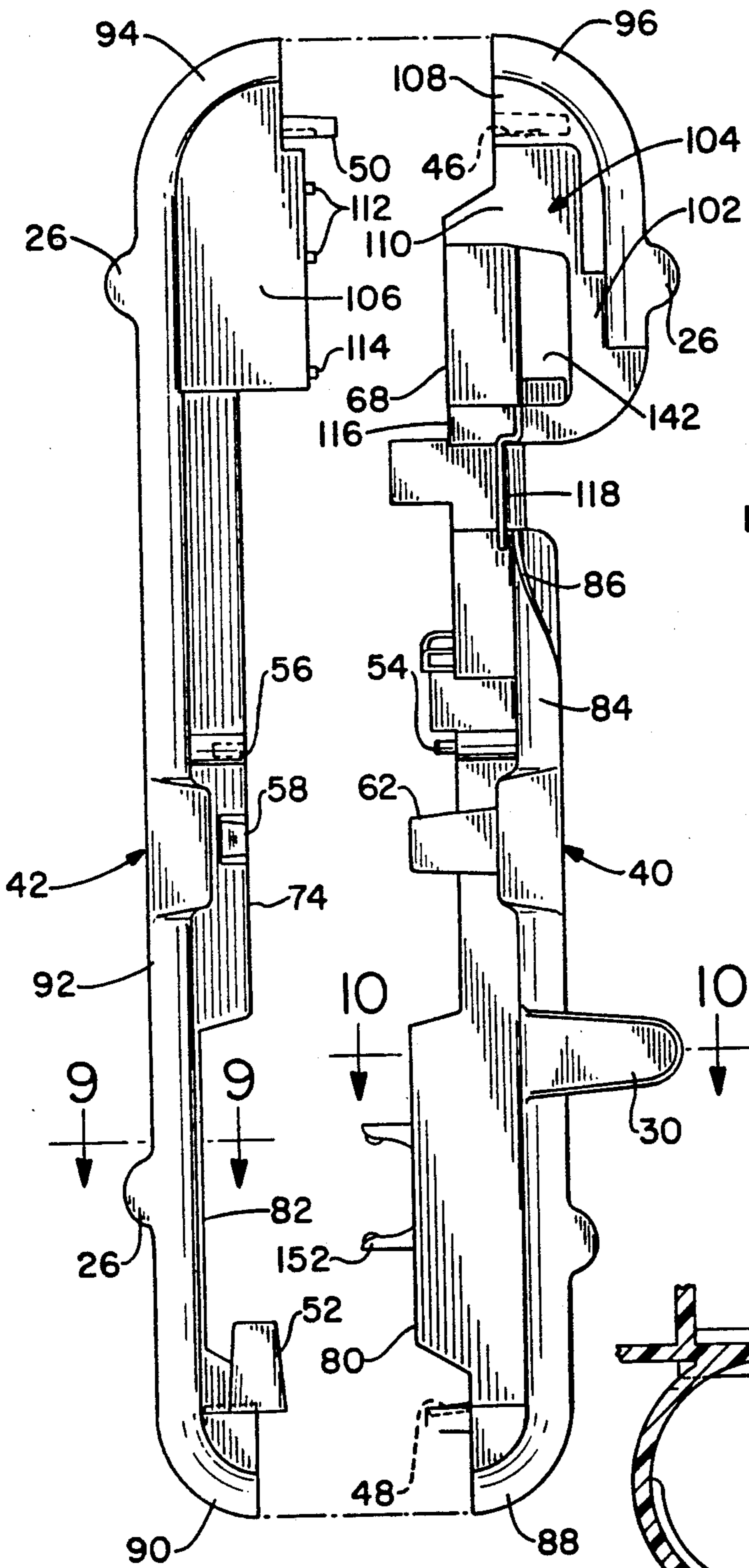
FIG. - 3
