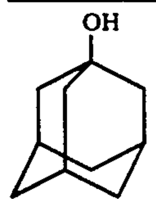
1-adamantanol
