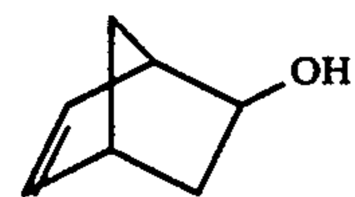
5-norbornen-2-ol
