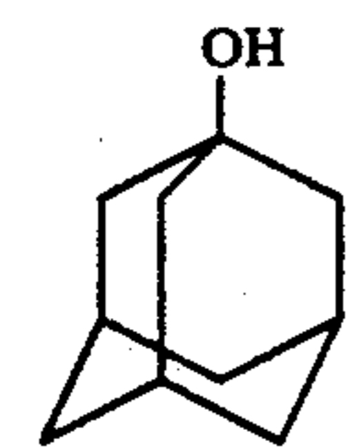
1-adamantanol
