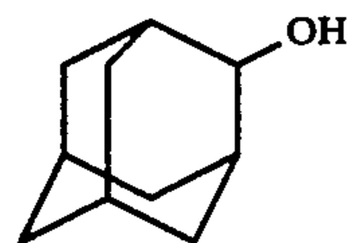
2-adamantanol
