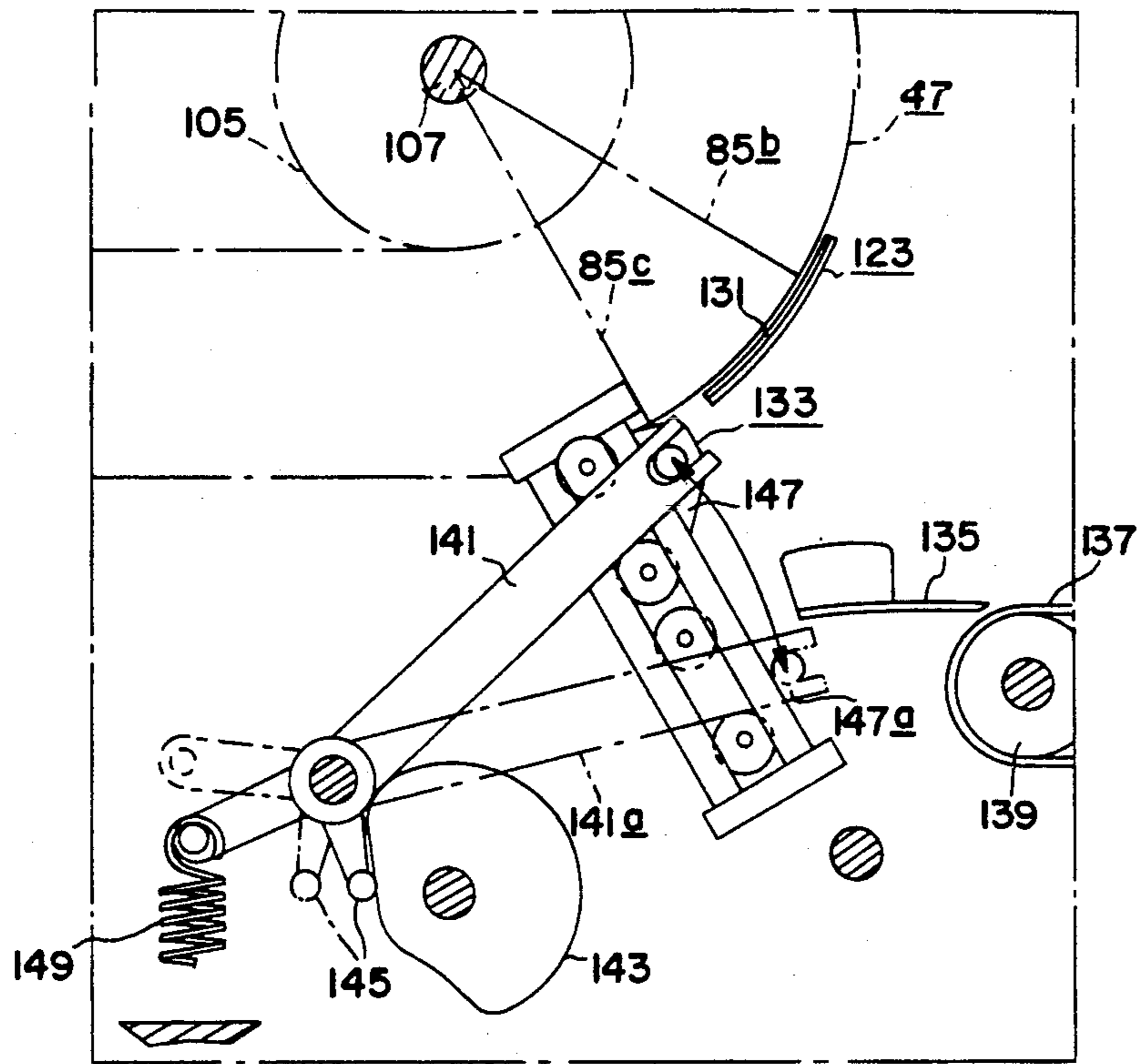
FIG. 5C (ELEVATOR CAM)
