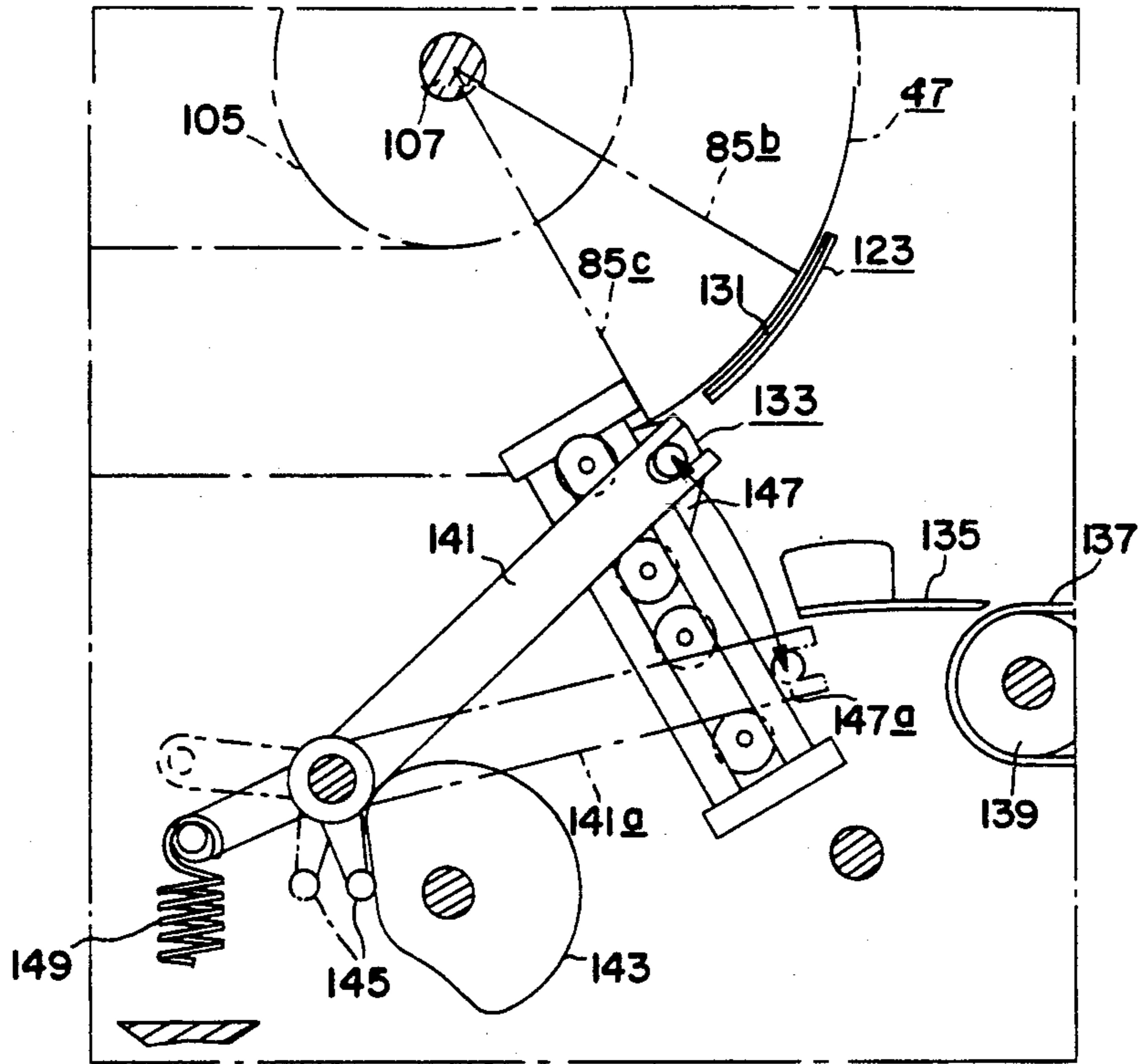
FIG. 5C (ELEVATOR CAM)
