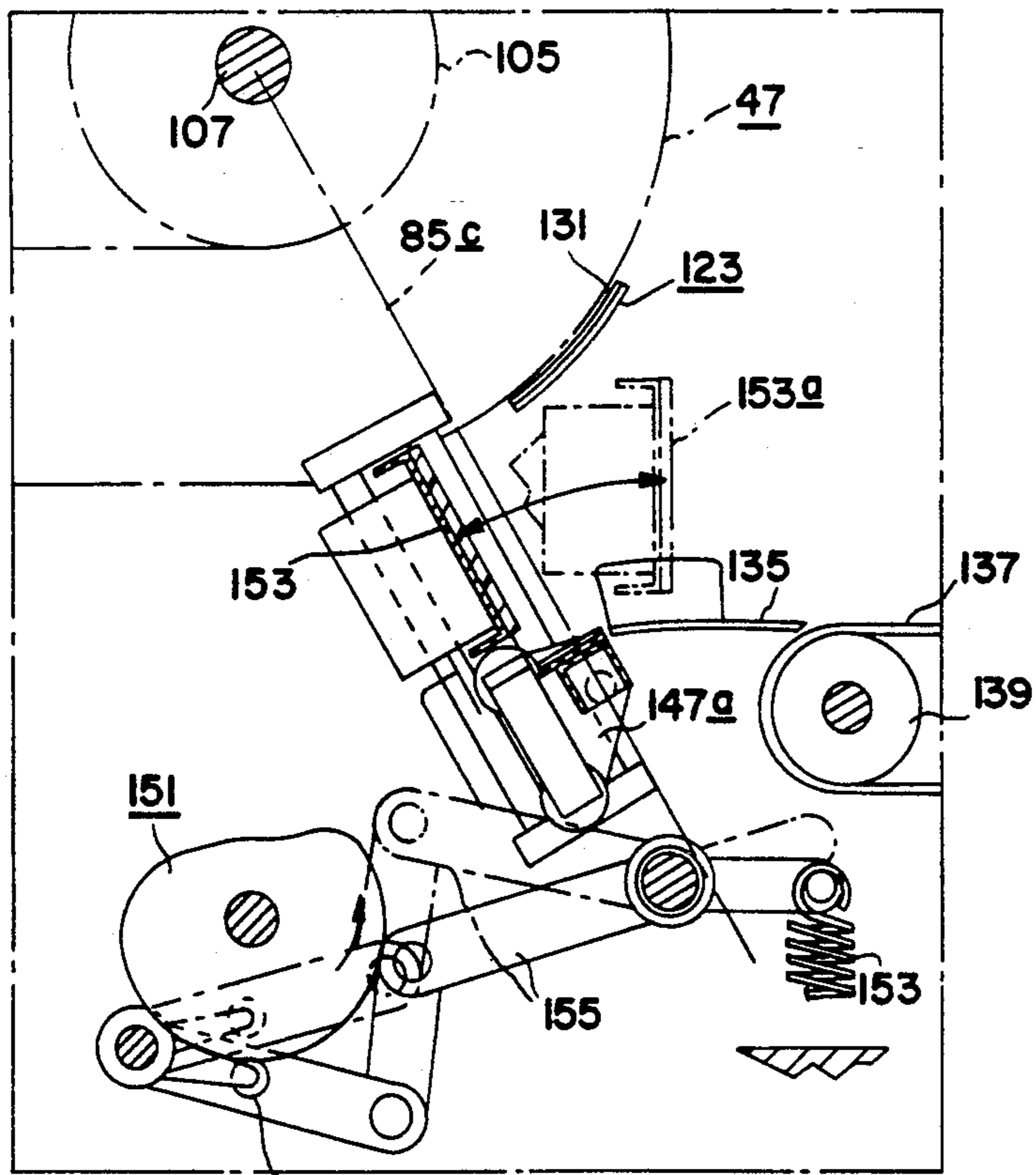
FIG. 5D (PUSHER CAM)
