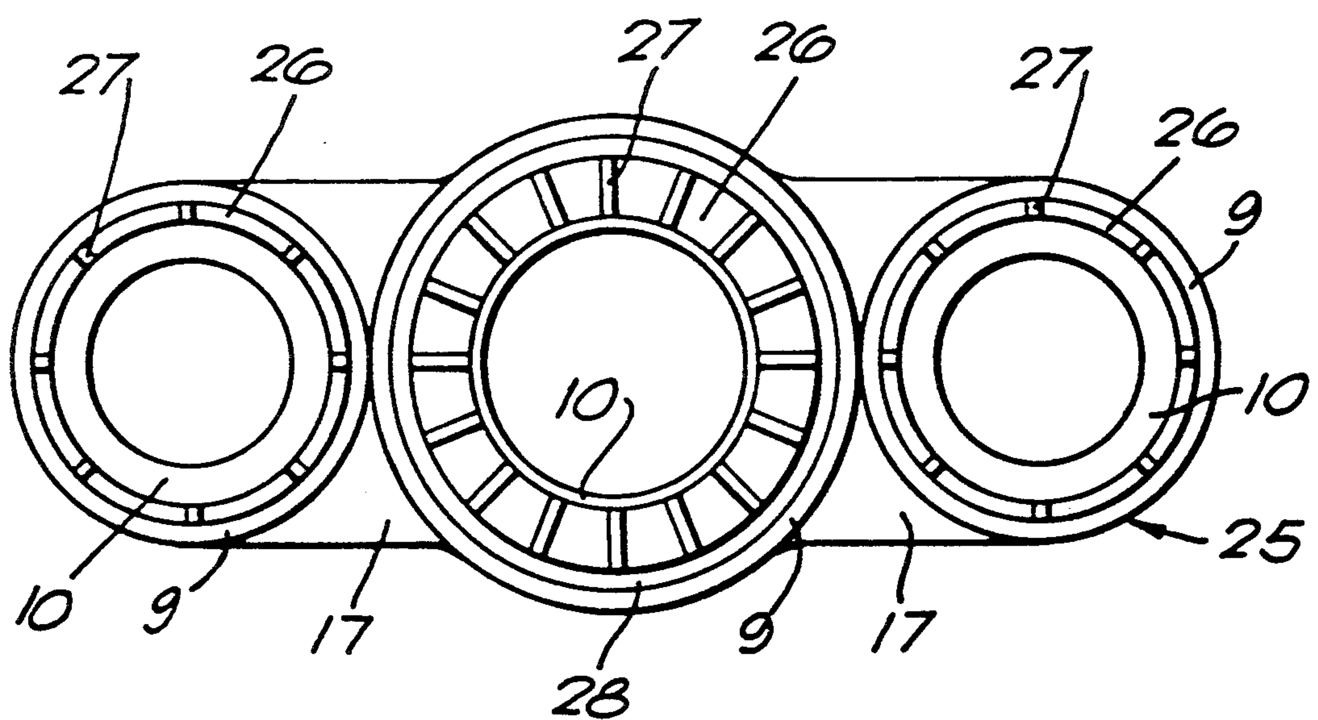
FIG. 5C
