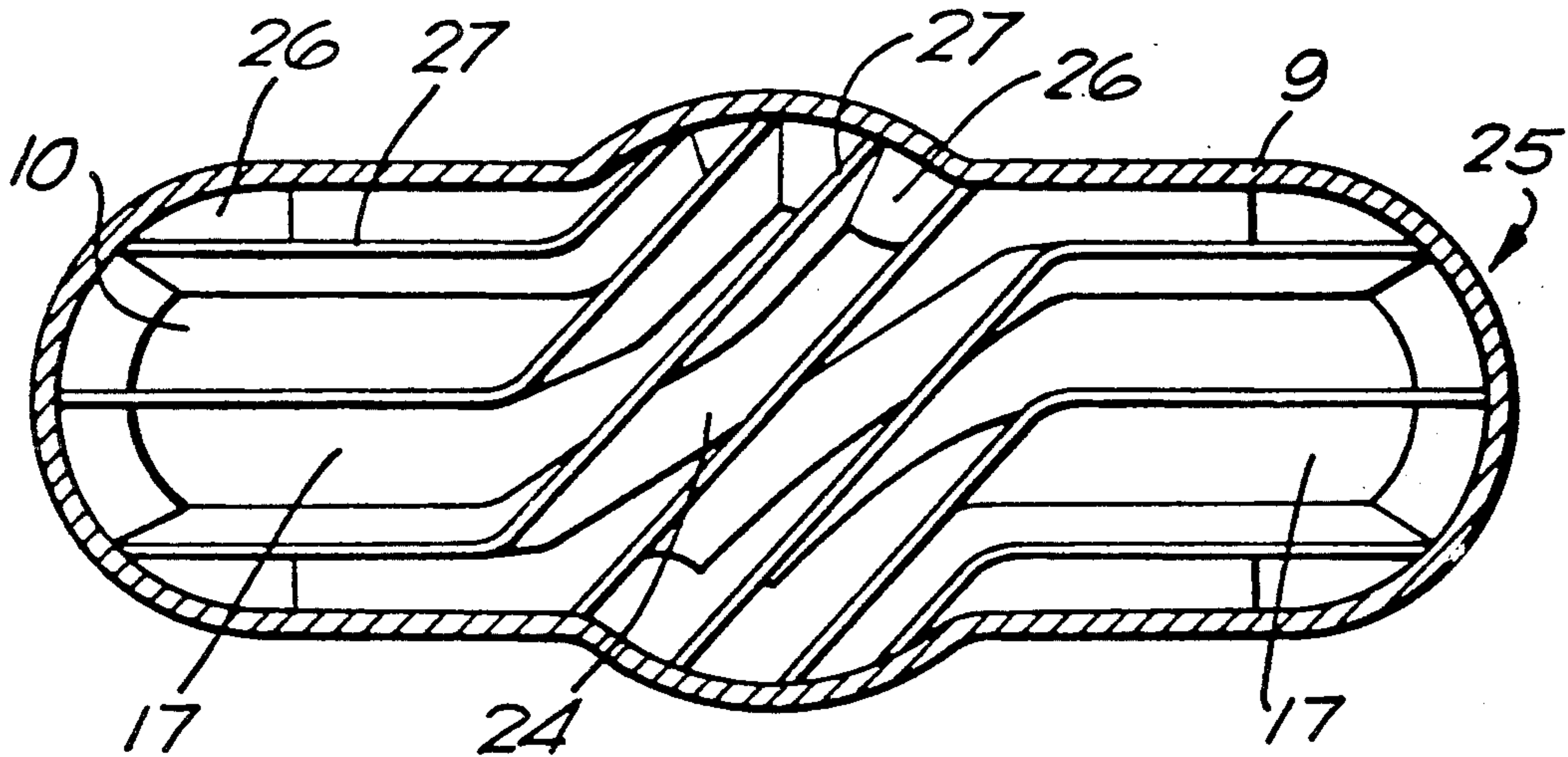
FIG. 5B
