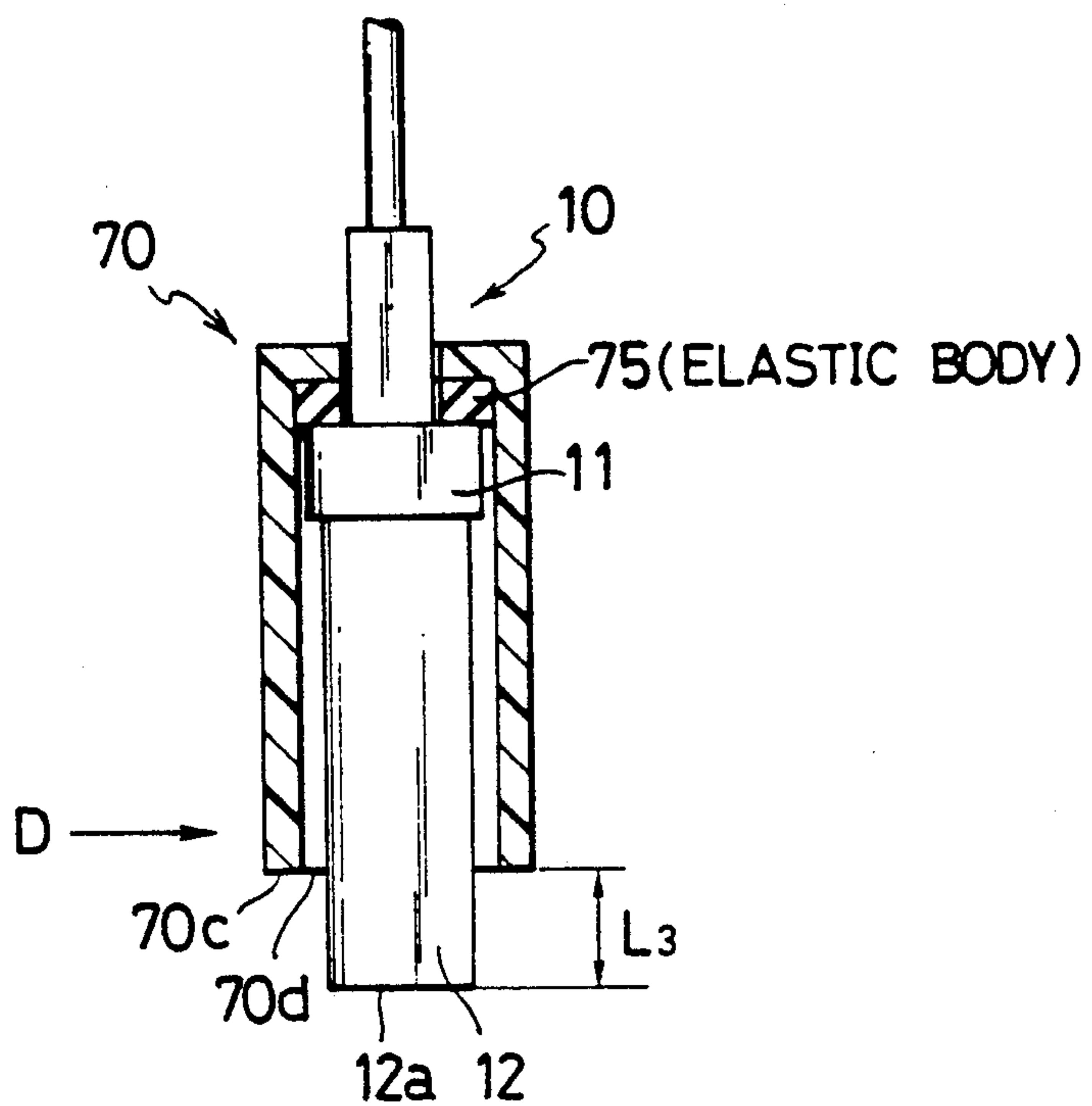
FIG. 8(B)
