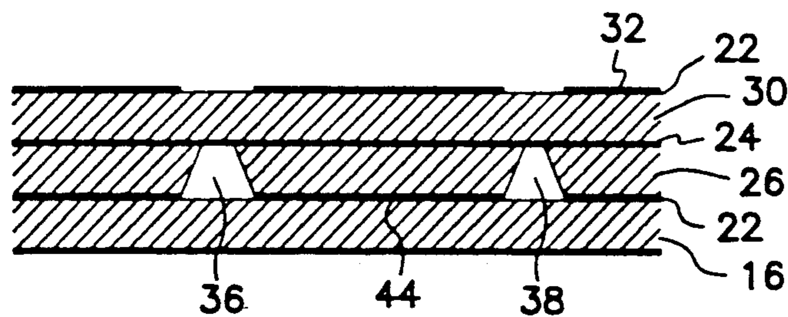
BOND BOTTOM STOP ANISOTROPIC Si ETCH FIG. 3E
