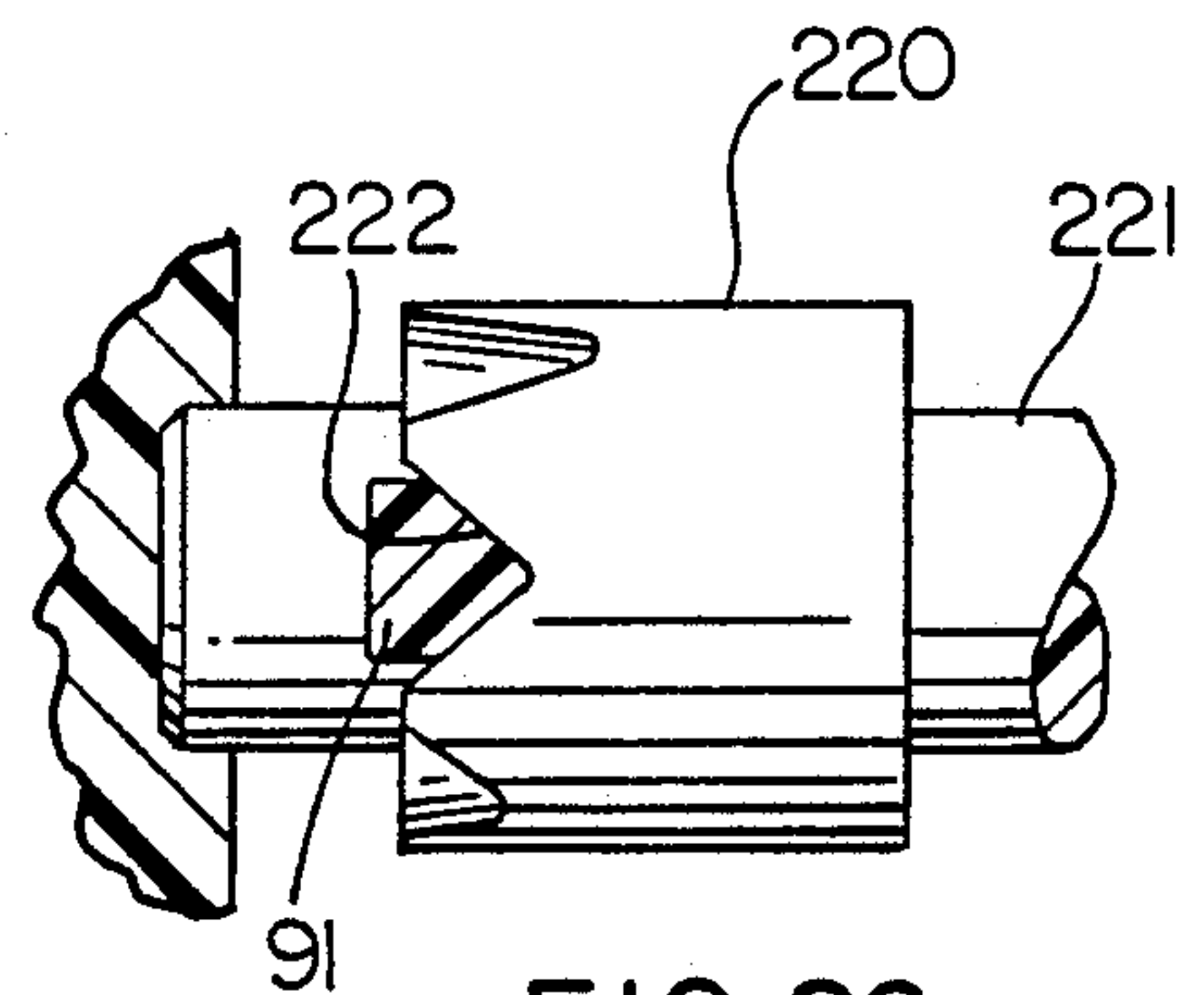
FIG. 26
