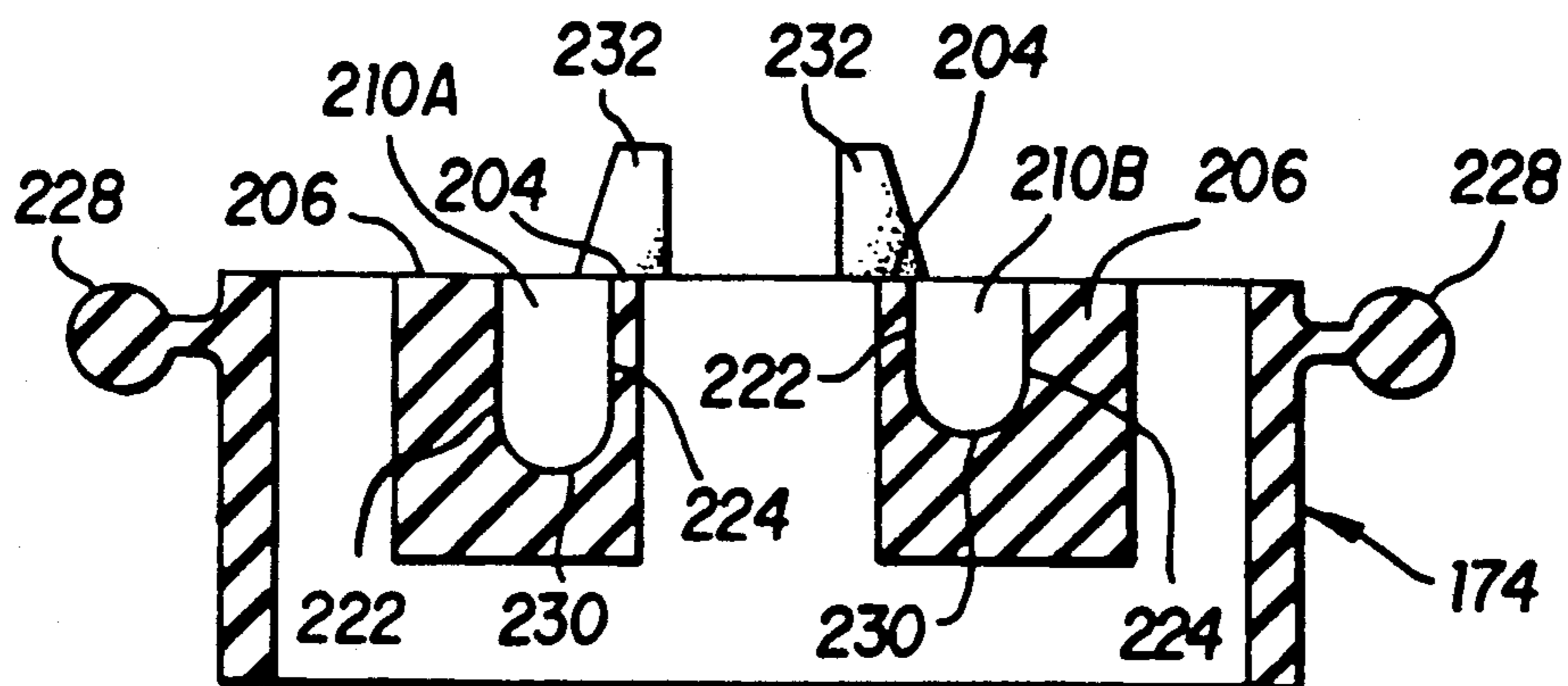
52 FIG. 11C
