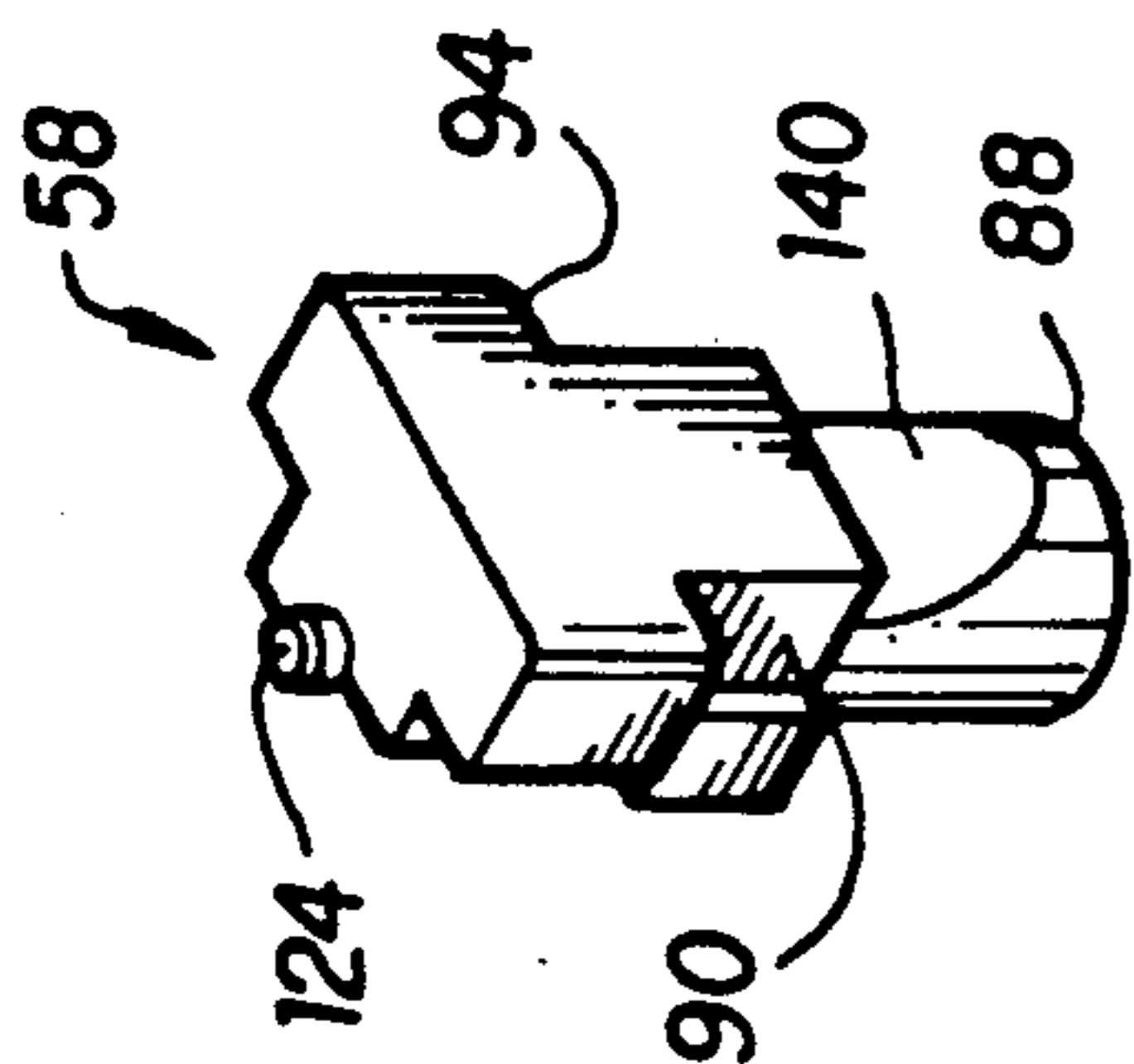
FIG. 8A
