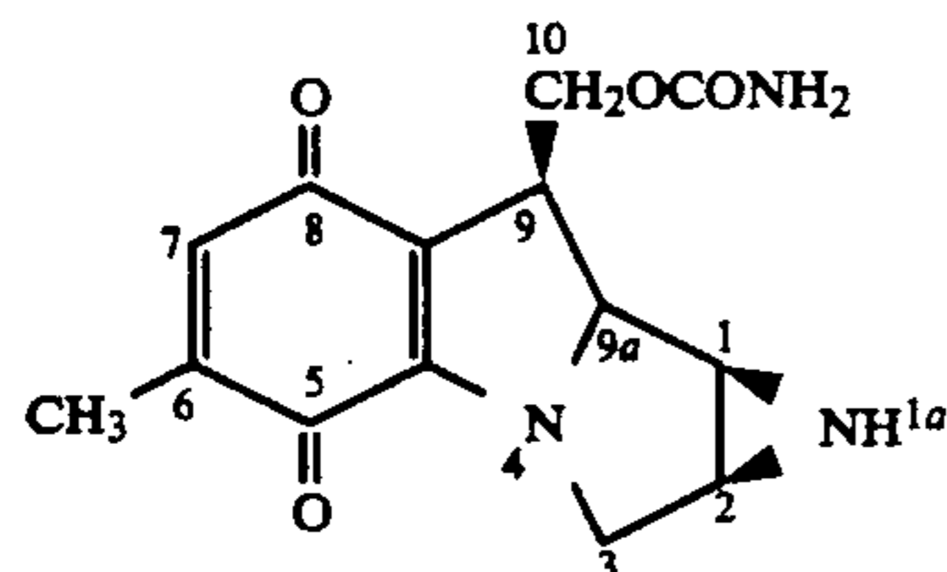
Mitosane
