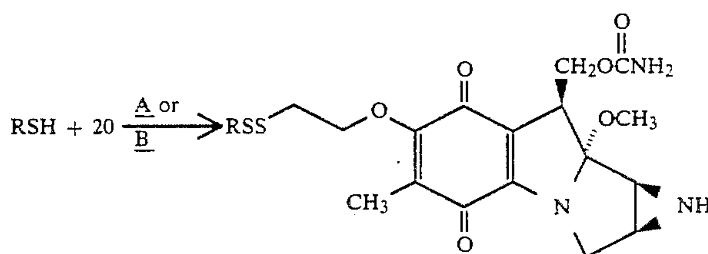
7-Alkoxydithio-9a-methoxymitosanes
