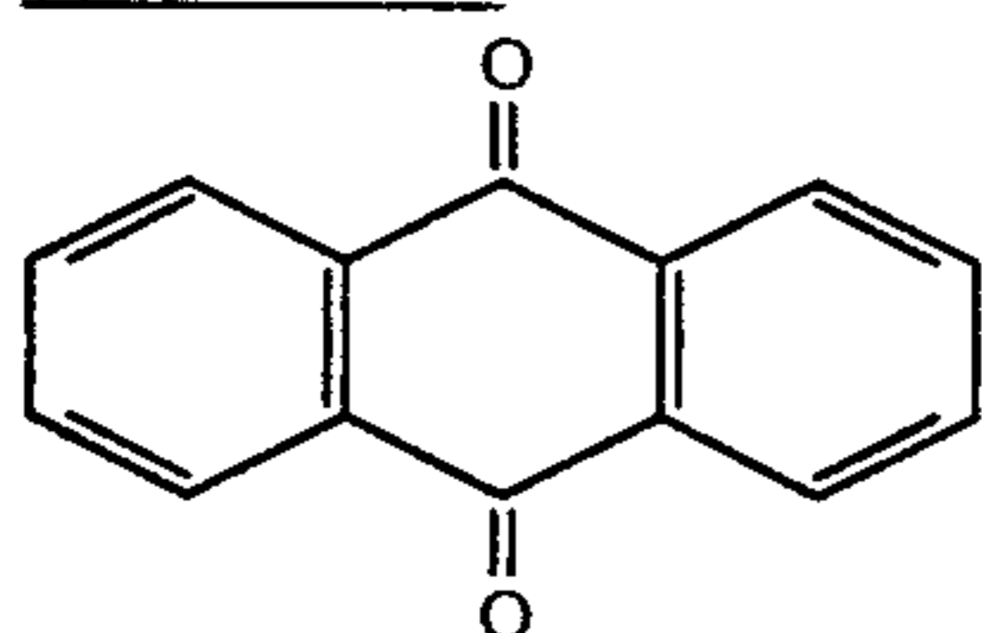
9,10-anthraquinone
