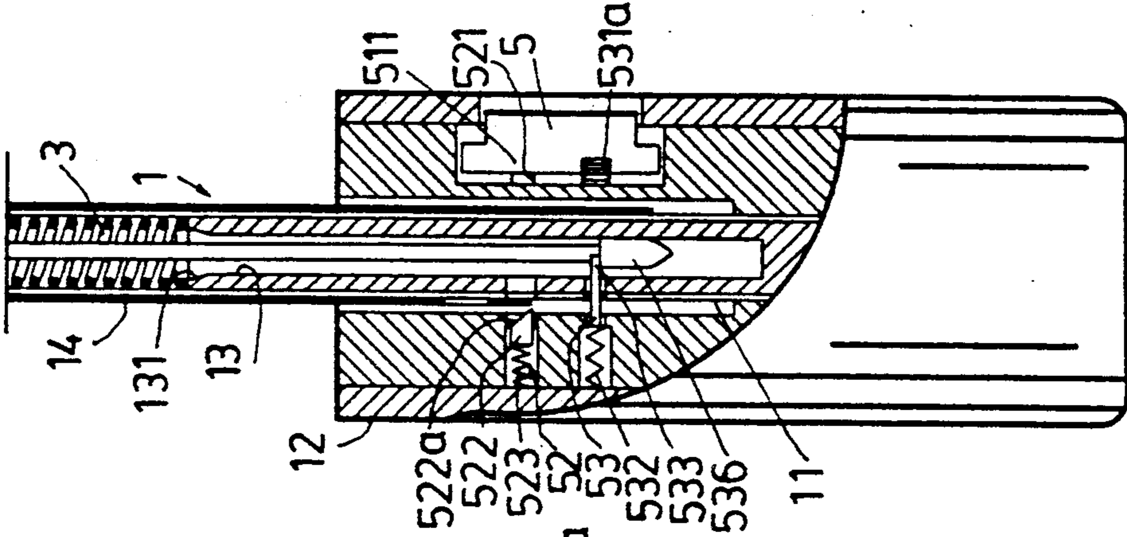
FIG.11
