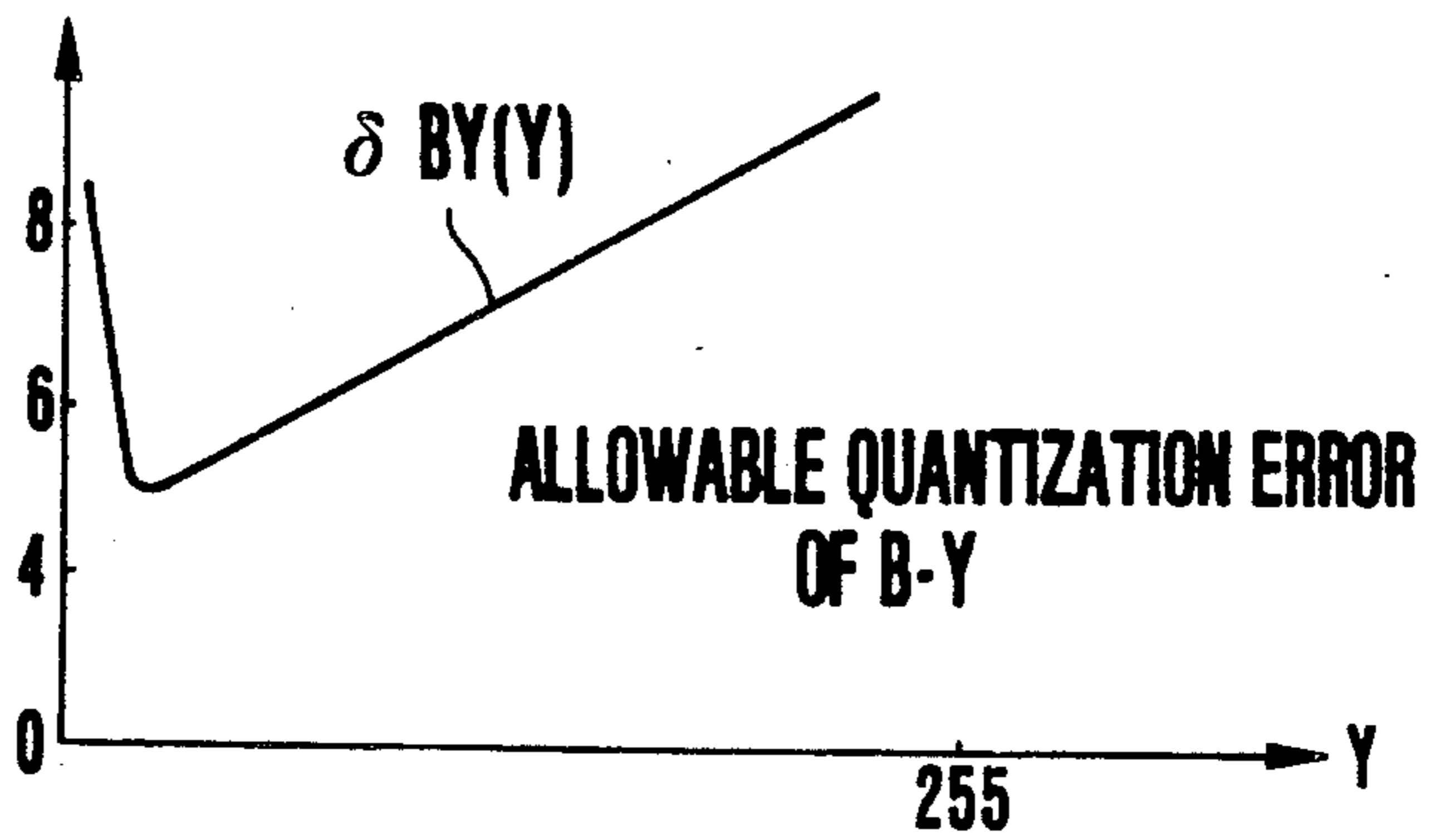
FIG.11(C)
