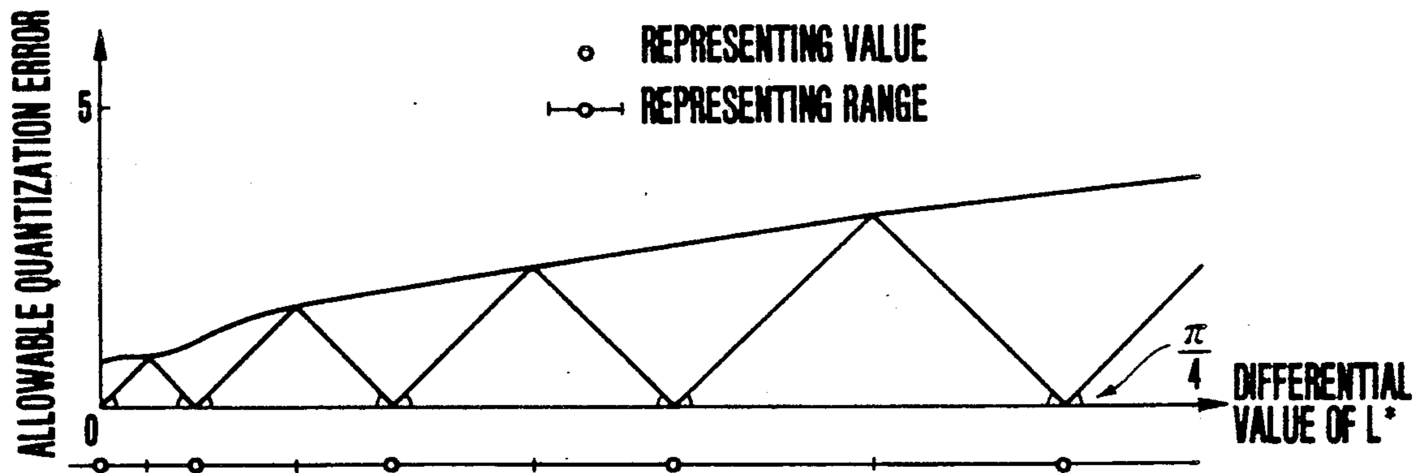
FIG. 31
