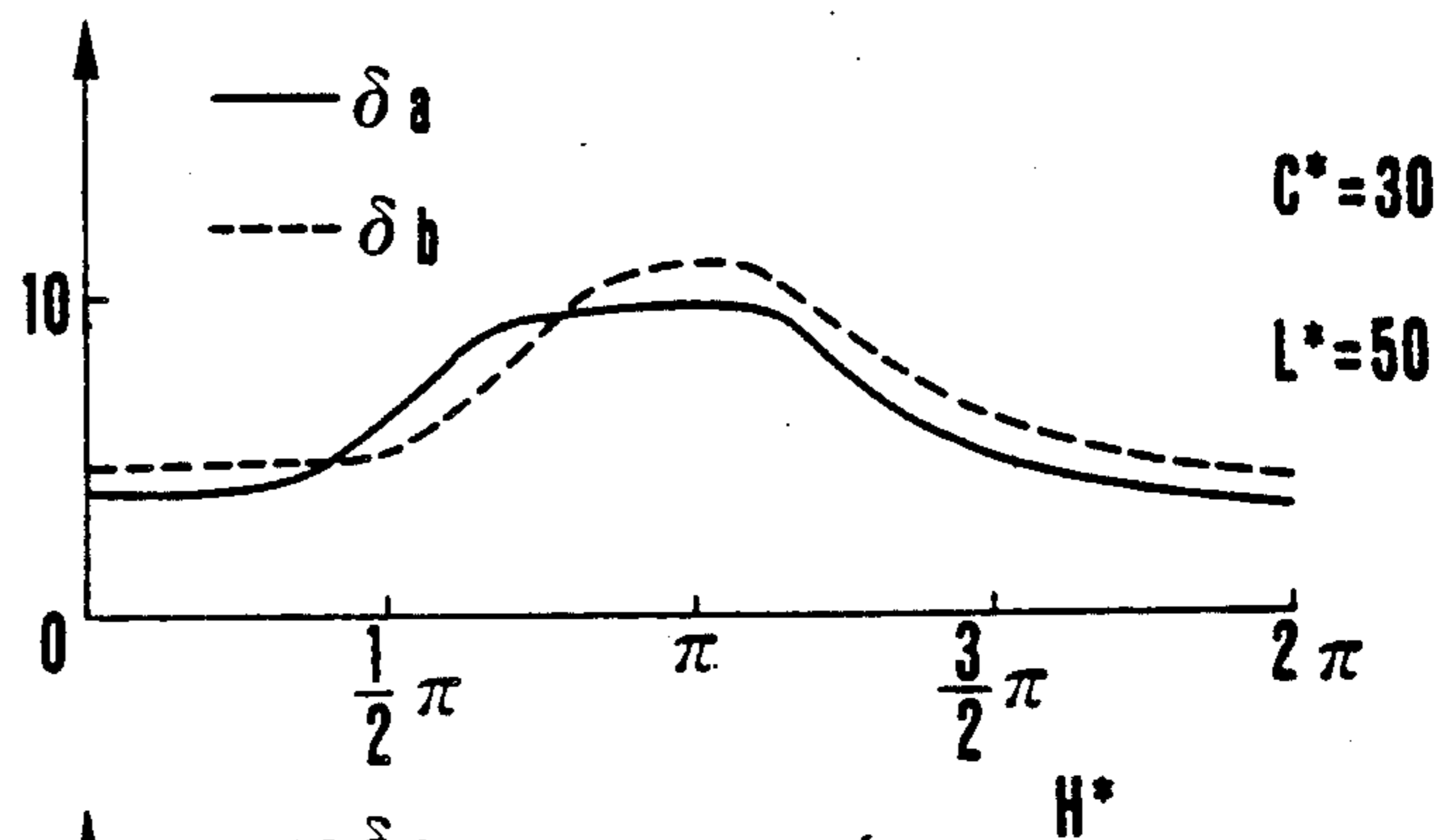
FIG. 28(C)
