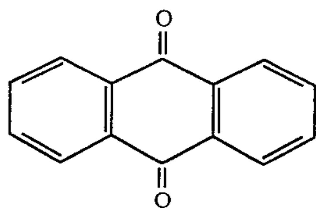
9,10-anthraquinone
