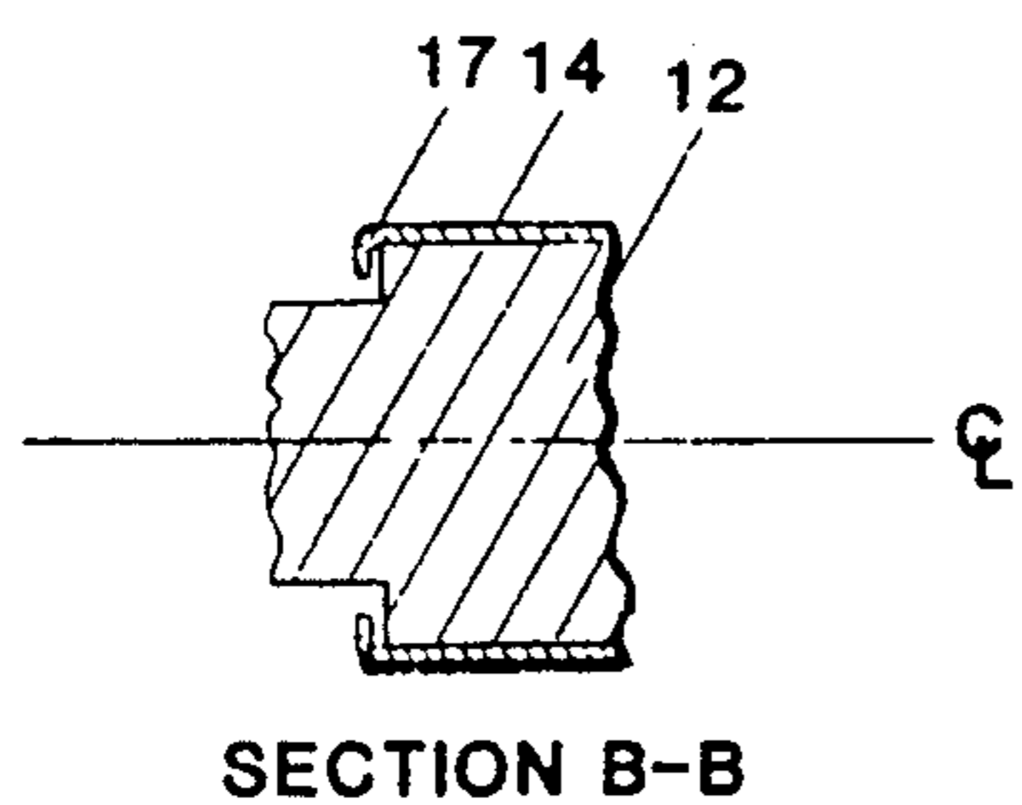
SECTION B-B FIG. 4
