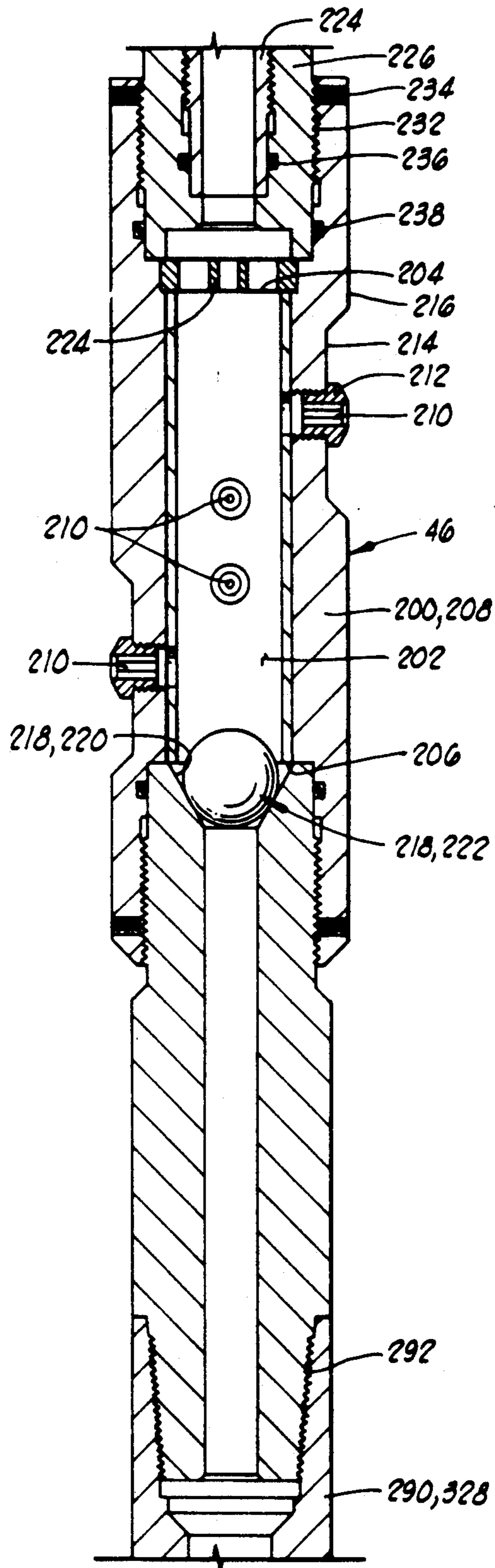
FIG. 30
