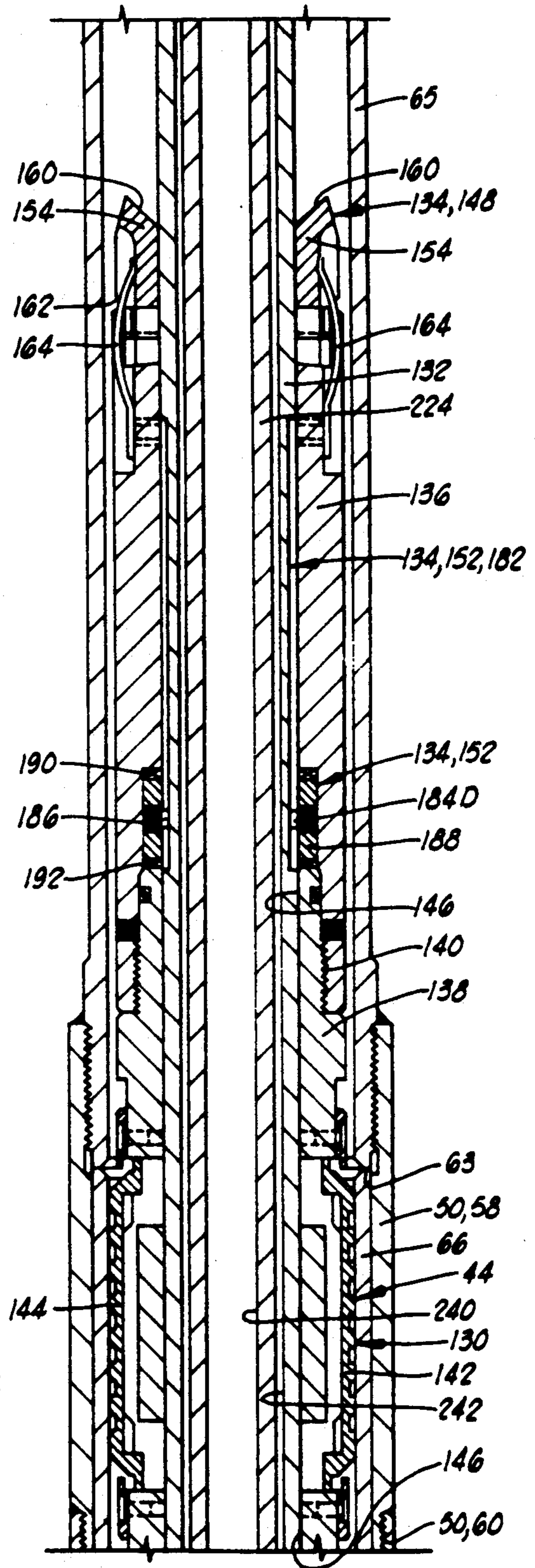
FIG. 4B
