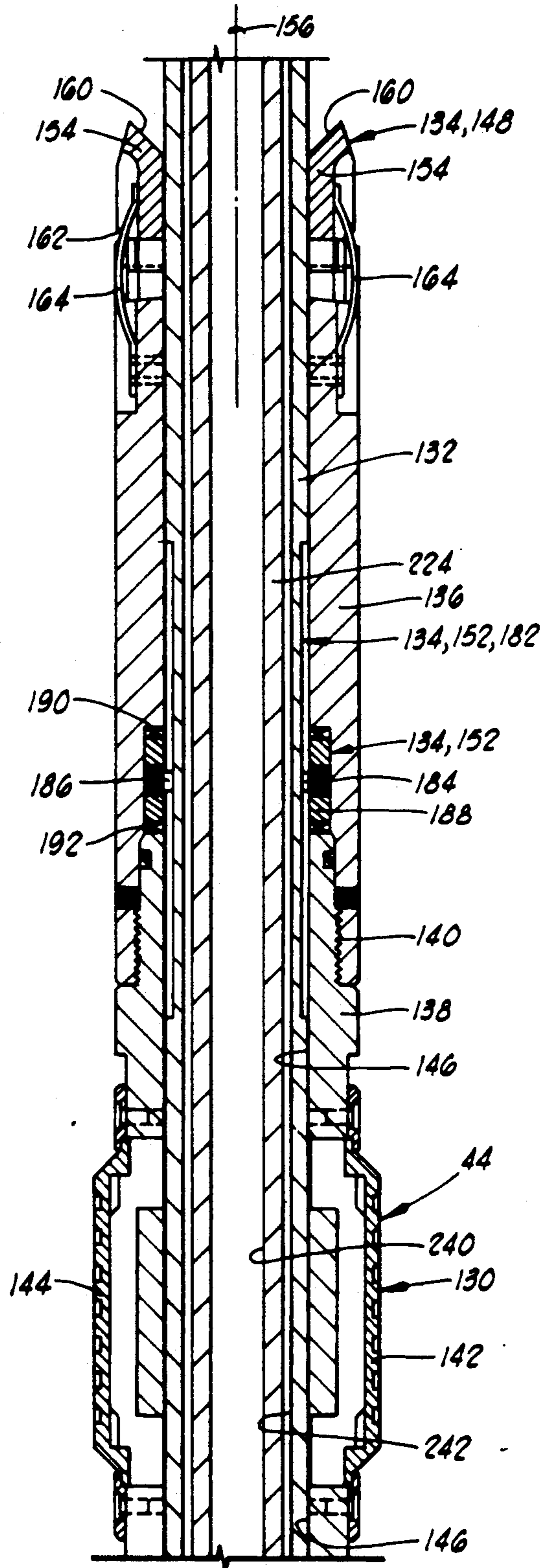
FIG. 3B
