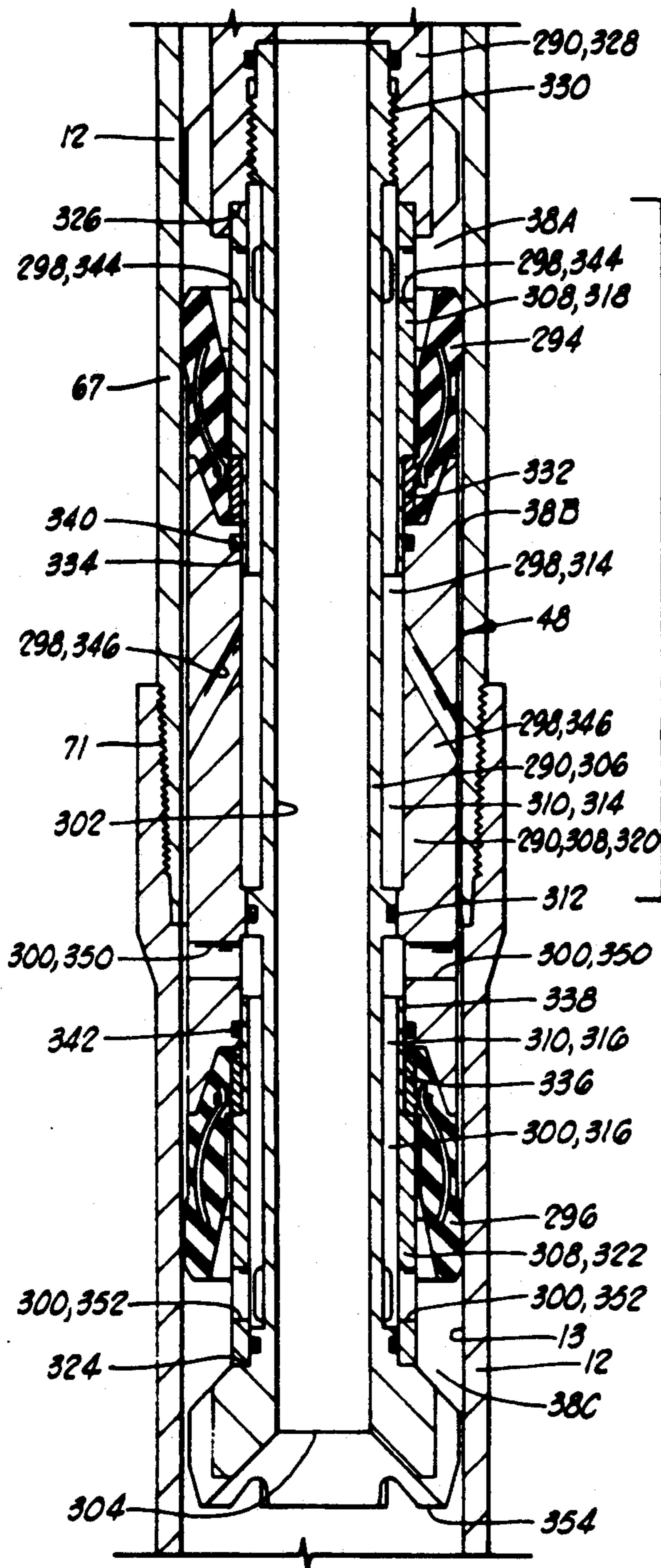
FIG. 4E
