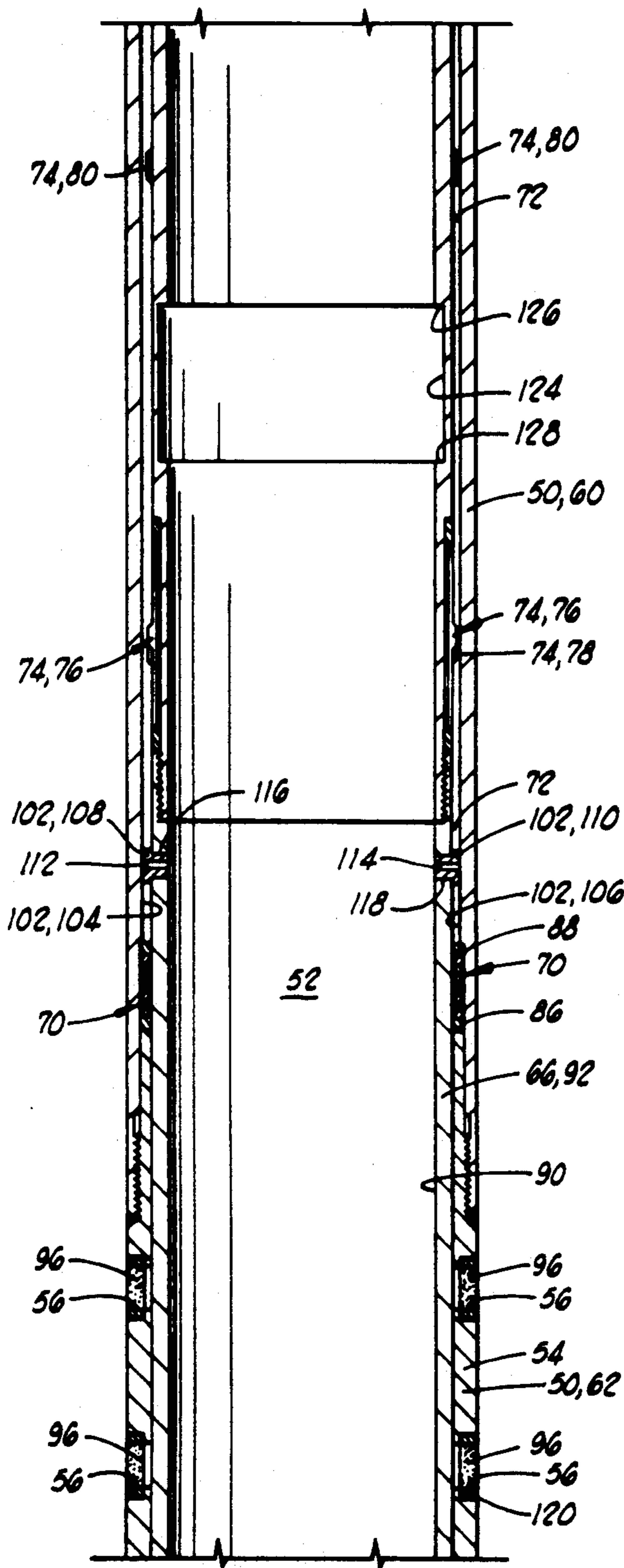
FIG. 2C
