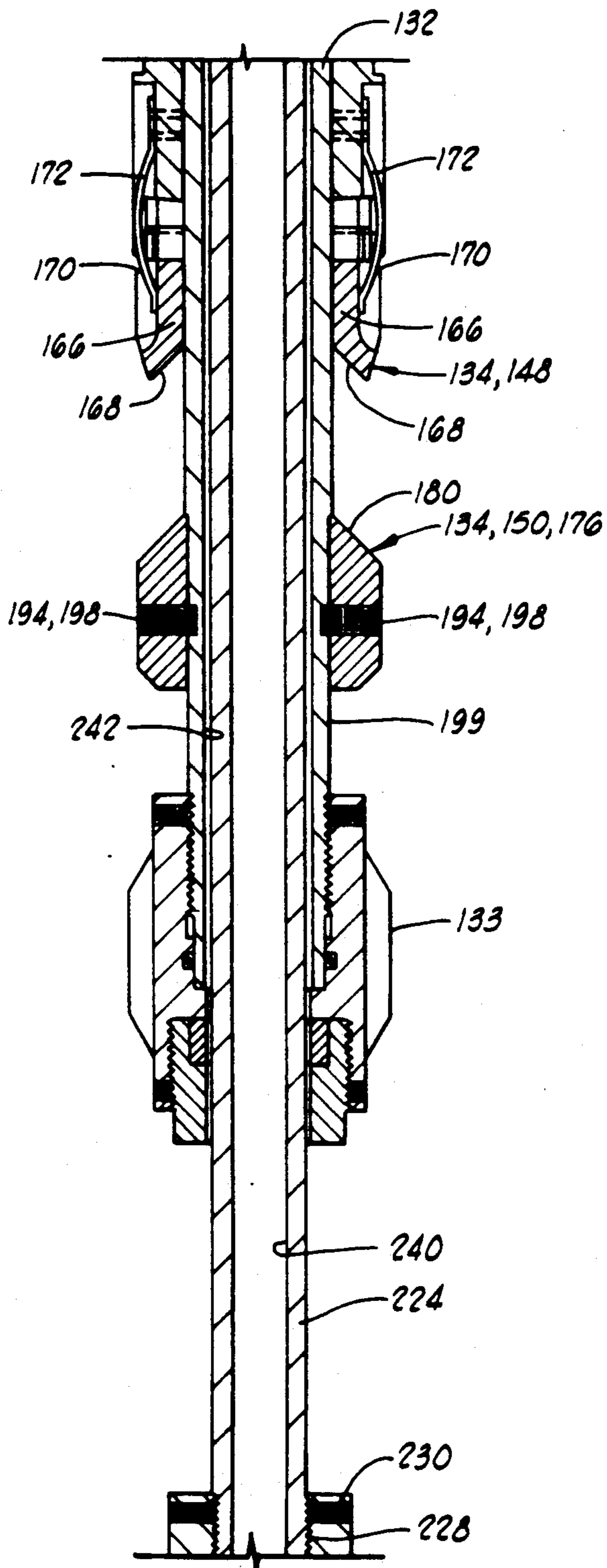
FIG. 30
