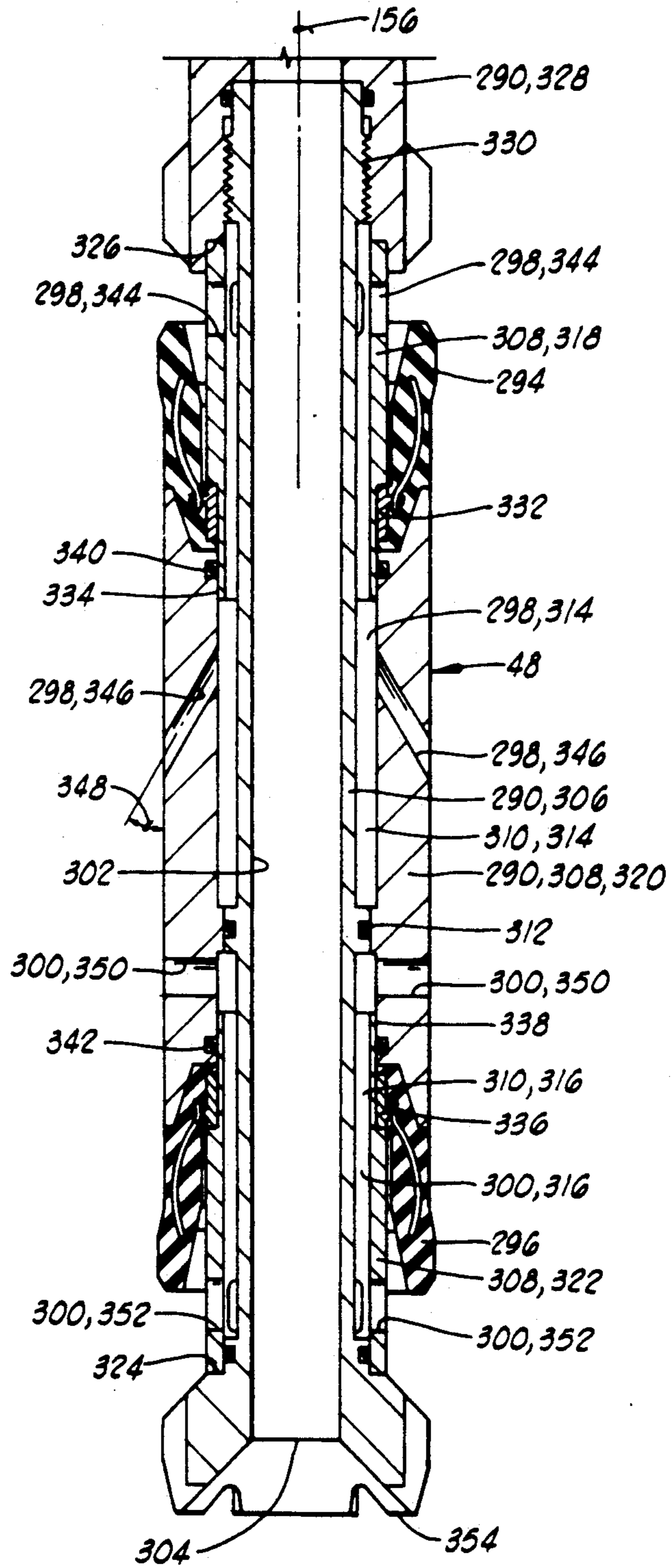
FIG. 3E
