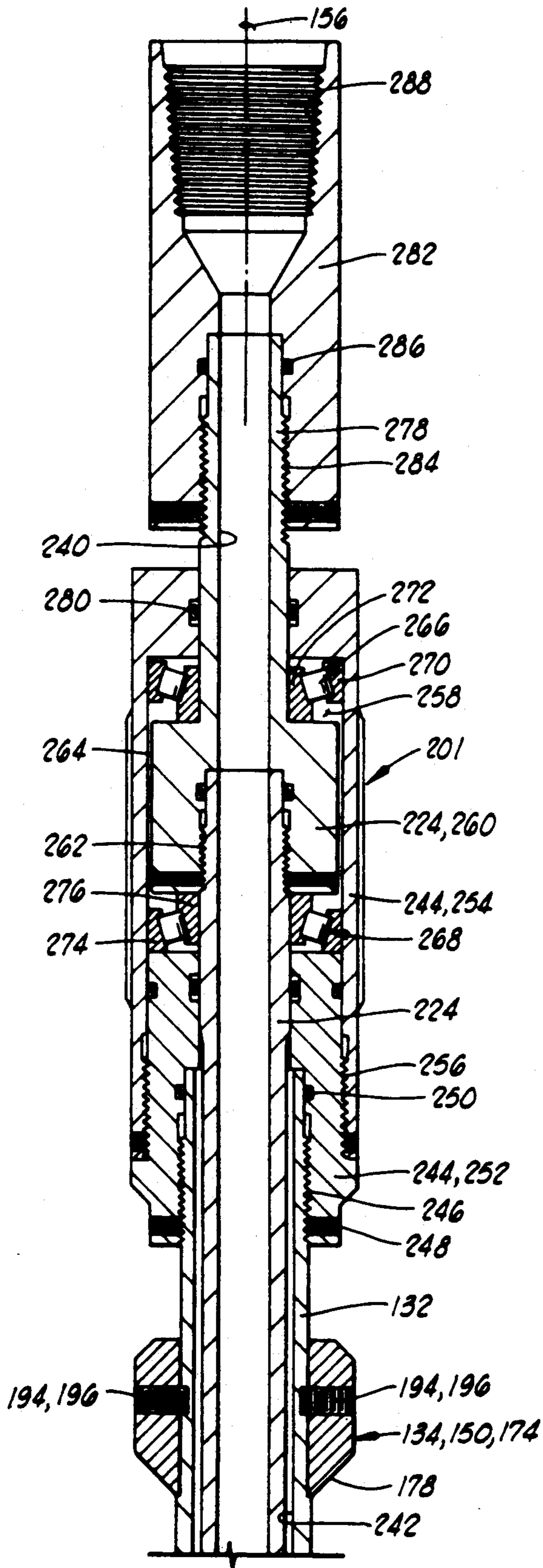
FIG. 3A
