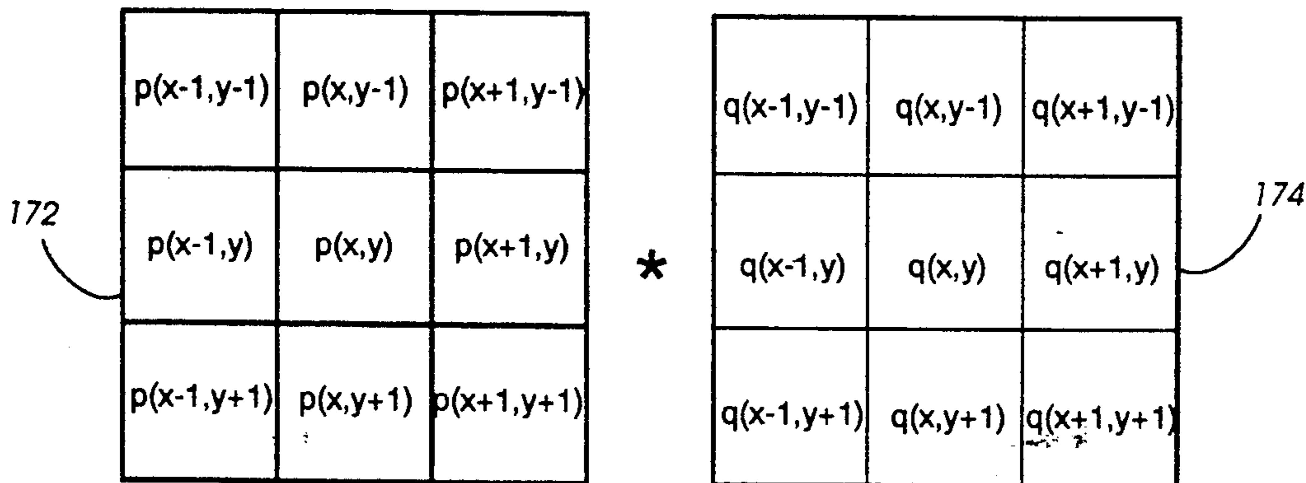
gradient mask
