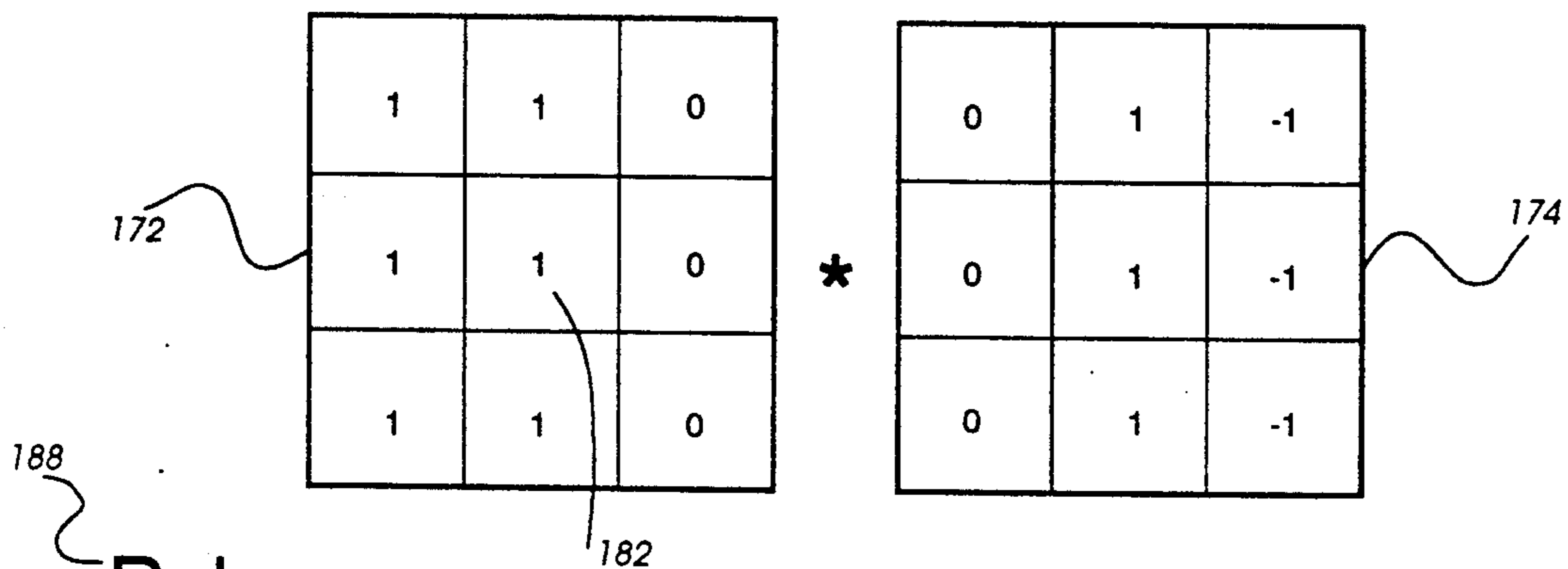
gradient mask
