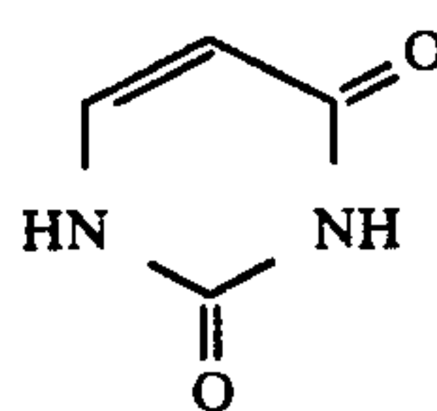
Uracil
